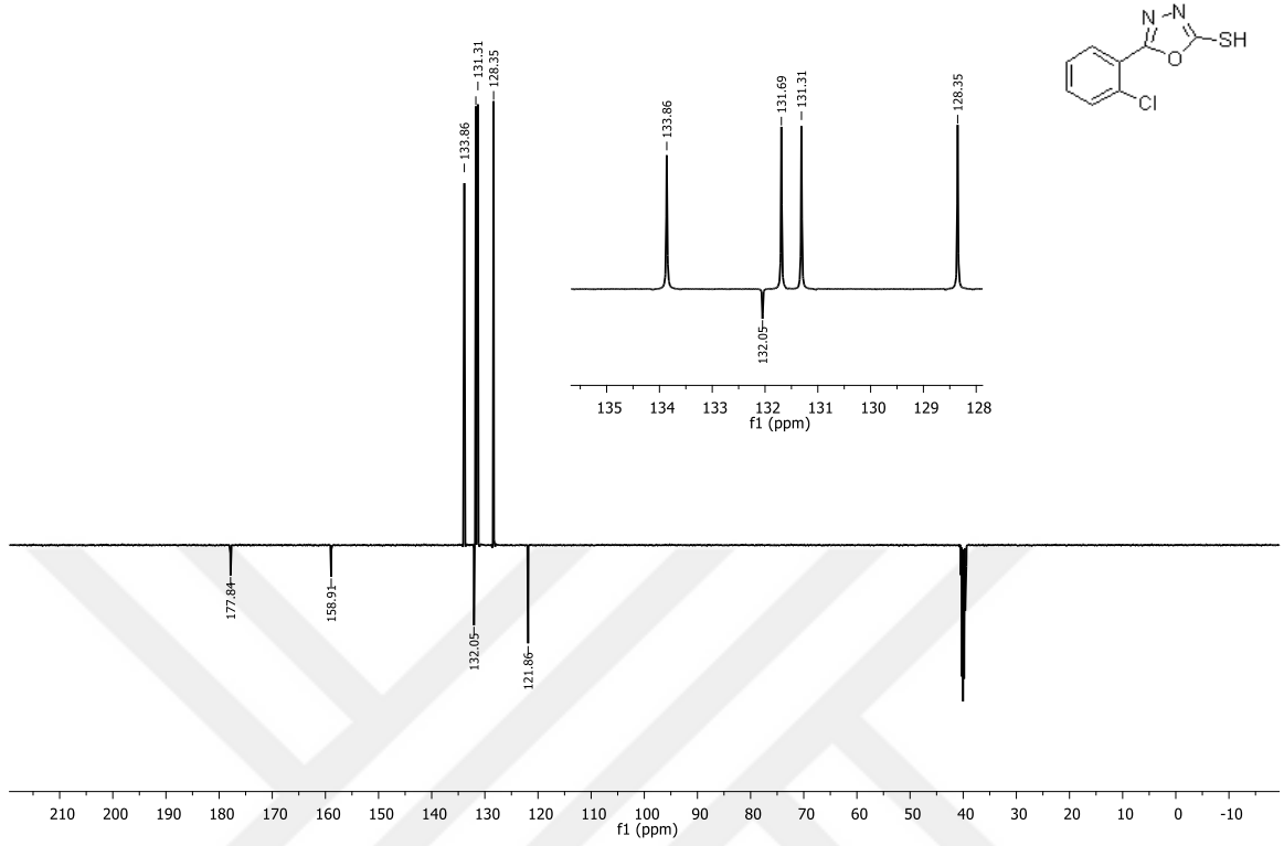
Şekil 3. 18. 2f'nin ^{13}\text{C} APT-NMR spektrumu
