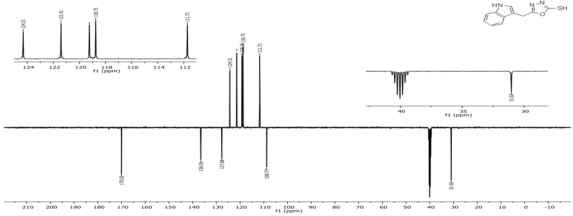
Şekil 3. 3: 2a'nın 13 C APT-NMR spektrumu
