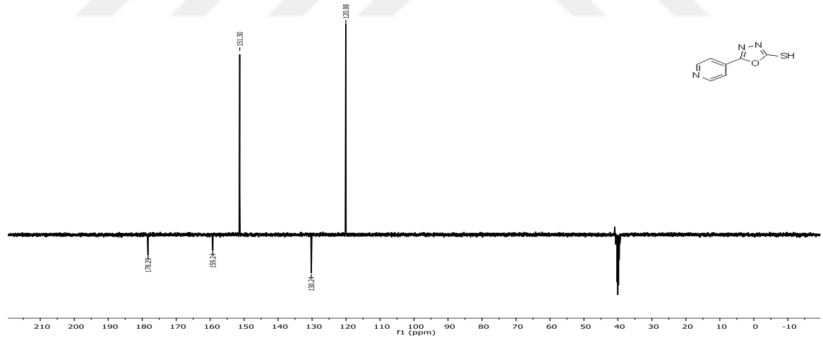
Şekil 3. 6. 2b'nin 13 C APT-NMR spektrumu
