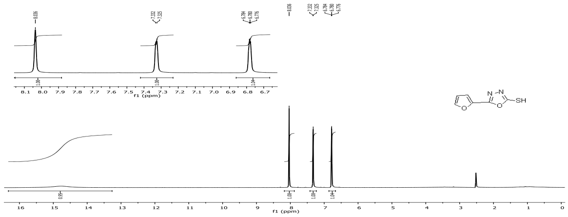
Şekil 3. 23. 2h'nin 1 H-NMR spektrumu
