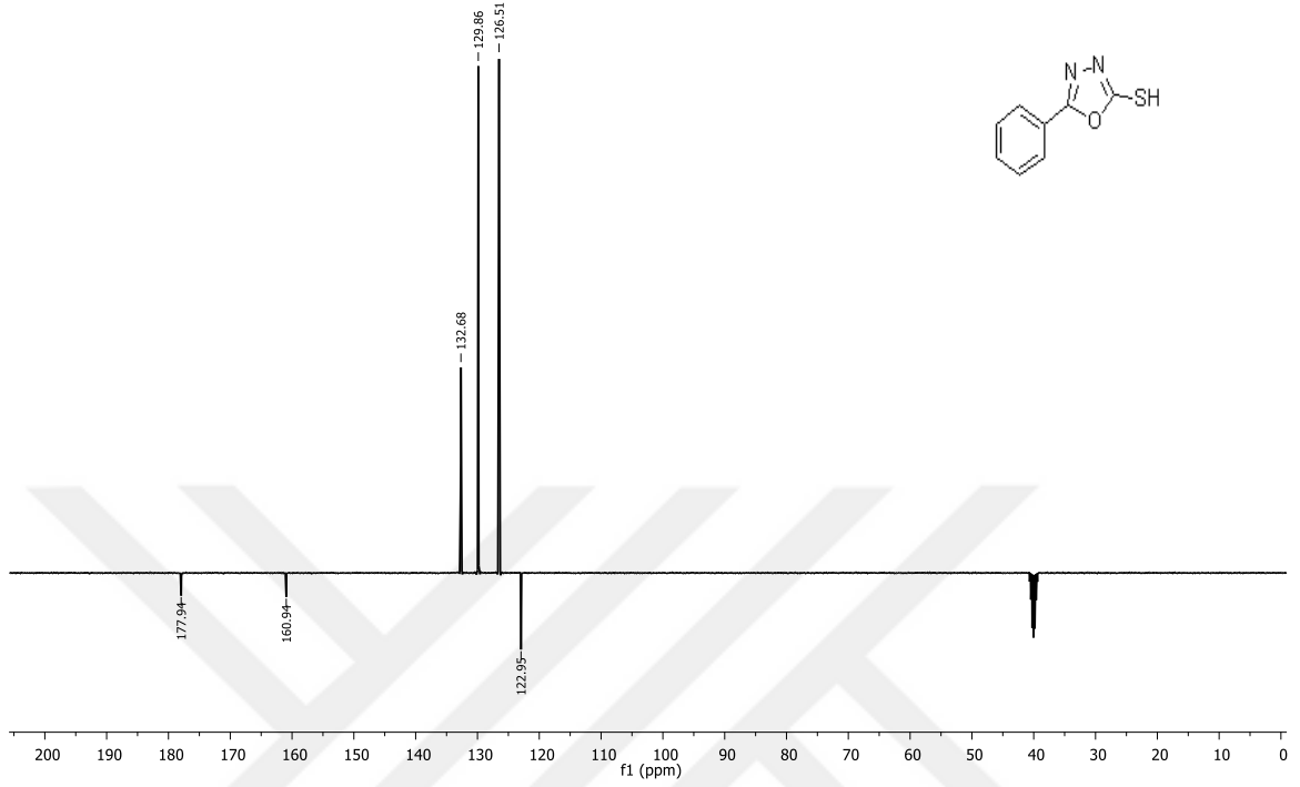
Şekil 3. 12. 2d'nin ^{13}\text{C} APT-NMR spektrumu
