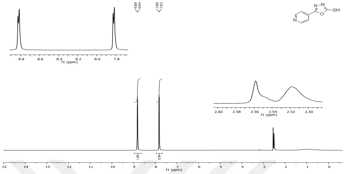
Şekil 3. 5. 2b'nin 1 H-NMR spektrumu
