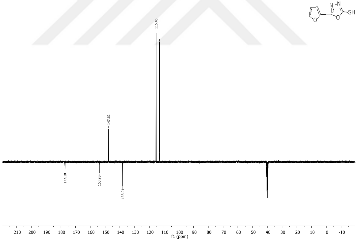
Şekil 3. 24. 2h'nin 13 C APT-NMR spektrumu
