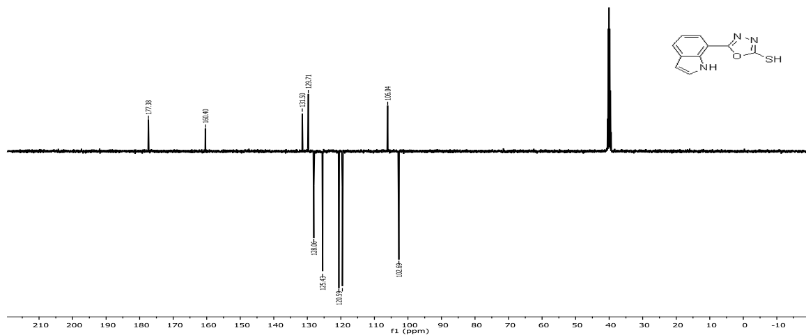
Şekil 3. 32. 2k'nın 13 C APT-NMR spektrumu
