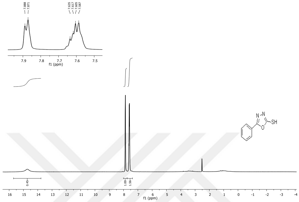
Şekil 3. 11. 2d'nin ^1\text{H} -NMR spektrumu
