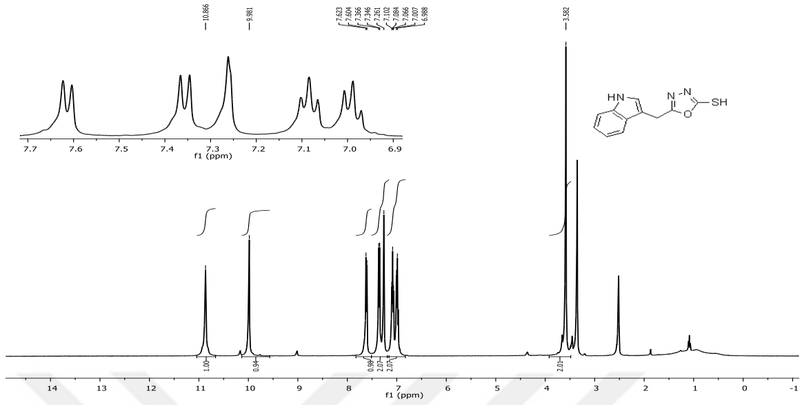
Şekil 3. 2. 2a'nın 1 H-NMR spektrumu
