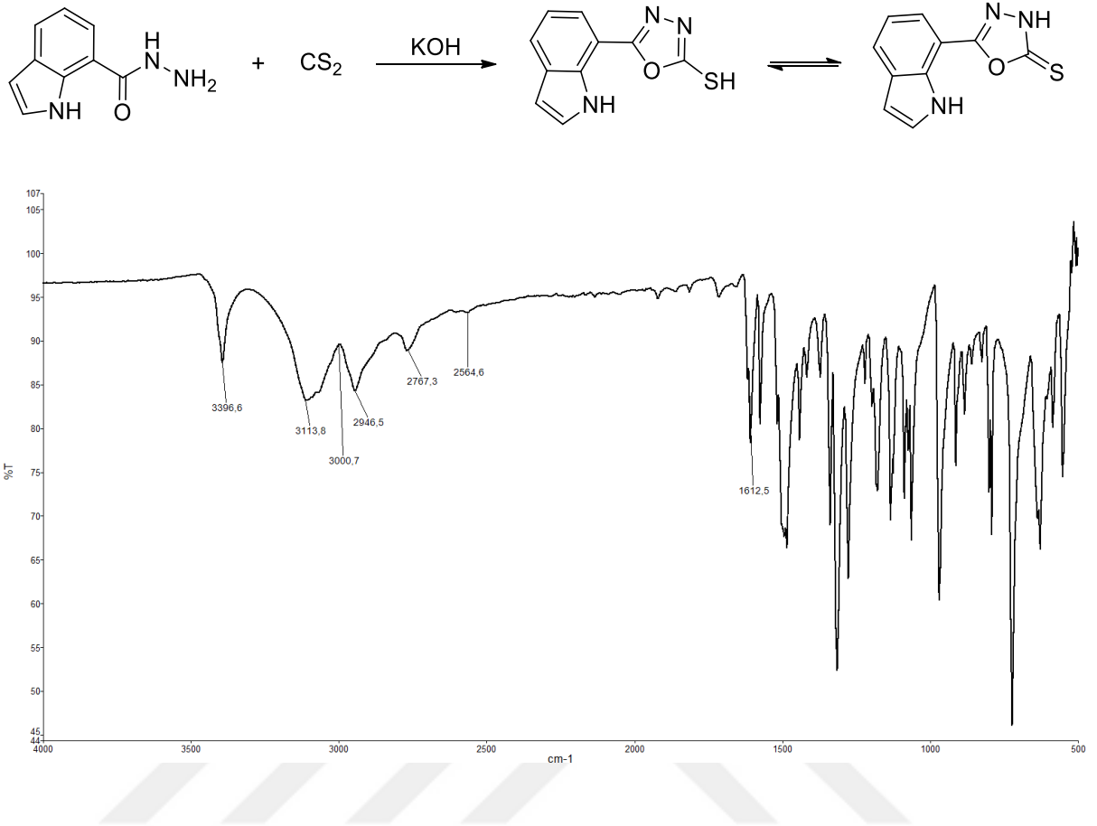
Şekil 3. 31. 2k'nın FT-IR spektrumu
