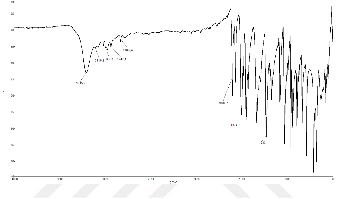
Şekil 3. 13. 2c'nin FT-IR spektrumu
