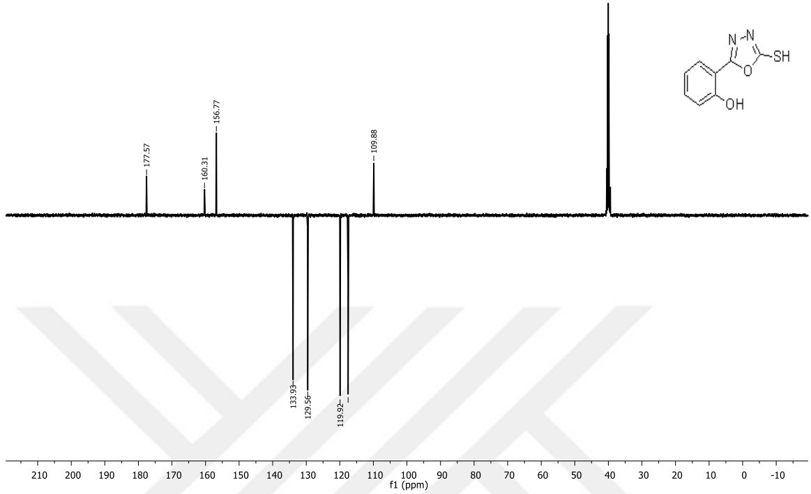
Şekil 3. 9. 2c'nin ^{13}\text{C} APT-NMR spektrumu
