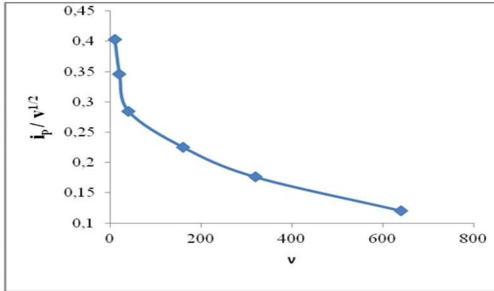
Şekil 5.6 \text{CuL}_2 kompleksinin GC elektrotta bazik pH'da (pH=8,00) DV deneylerinden elde edilen sonuçlar için tarama hızı ile akım fonksiyonunun değişimi
