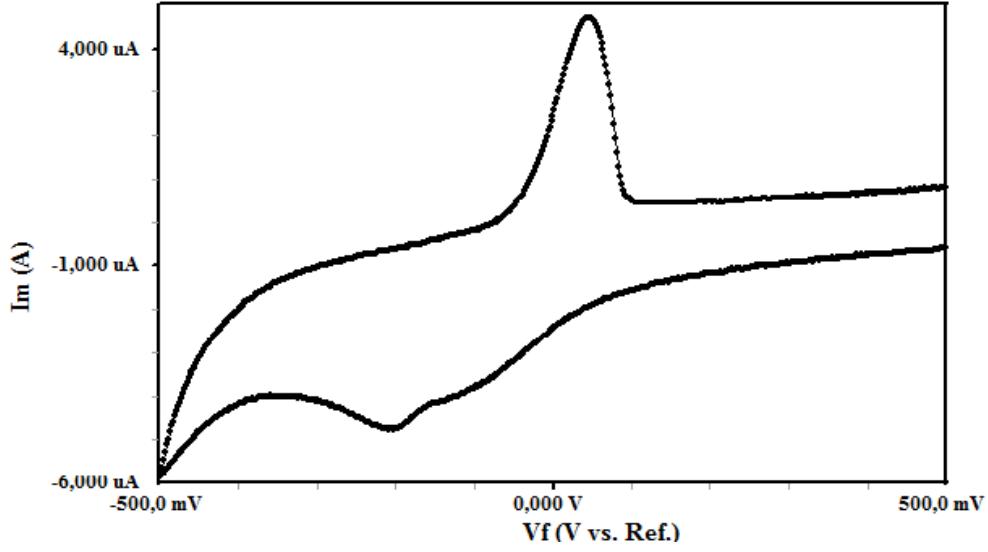
Şekil 4.12 \text{Ni}(\text{NO}_3)_2 tuzunun \text{pH}=2,12 'de 100 \text{ mV s}^{-1} tarama hızında +500 \text{ mV} ile -500 \text{ mV} arasında Gamry cihazında kaydedilen dönüşümlü voltamogramı
