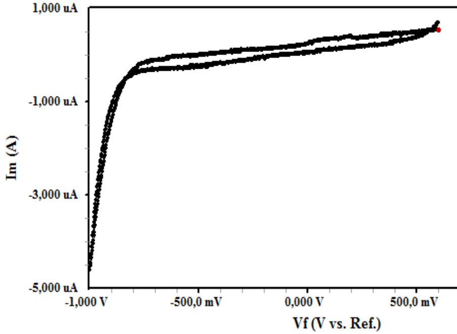
Şekil 4.2 +600 ile -1000 mV potansiyel aralığında pH=9,80’de 100mV s -1 tarama hızıyla Gamry cihazında kaydedilen tanık çözeltinin dönüşümlü voltamogramı
