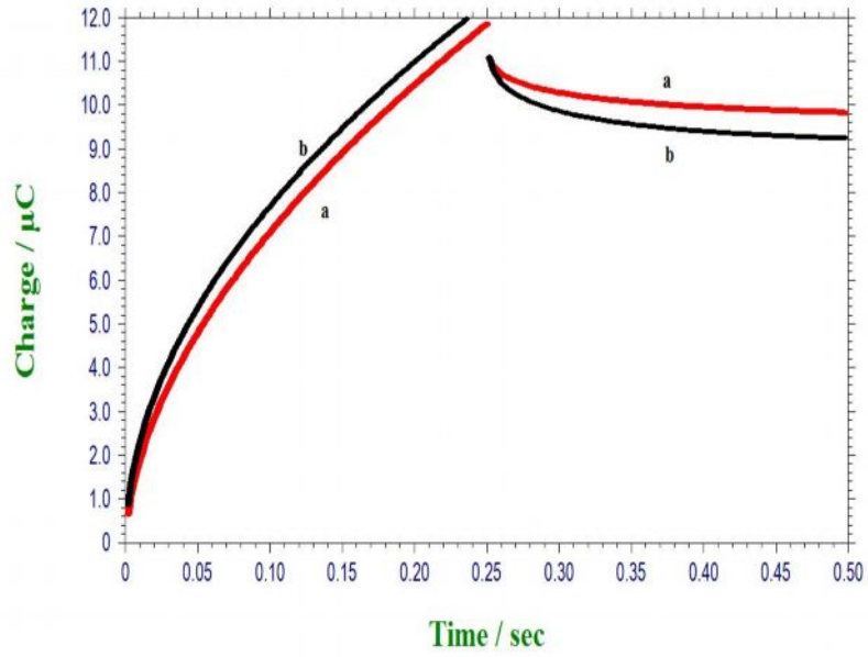
Şekil 4.20 Ligandın farklı pH'larında CHI cihazında kaydedilen kronokulometrik voltamogramı (a): pH=8,00; (b): pH=10,00.
