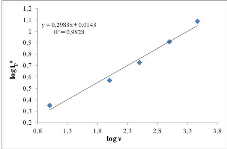
Şekil 5.12 NiL 2 kompleksinin GC elektrotta pH=10,00'de katodik pik için farklı tarama hızlarında alınan dönüşümlü voltamogramlarından elde edilen log i p 1 - log v grafiği
