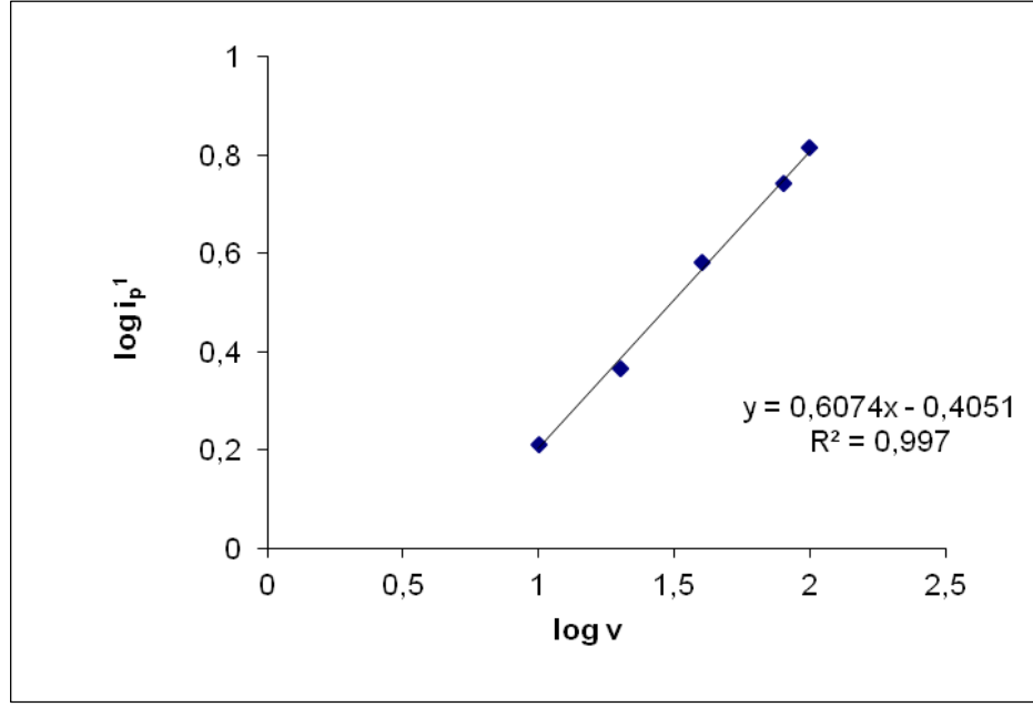
Şekil 5.5 \text{CuL}_2 kompleksinin GC elektrotta bazik pH'da (pH=8,00) farklı tarama hızlarında alınan dönüşümlü voltamogramlarından elde edilen \log i_p^1 - \log v grafiği
