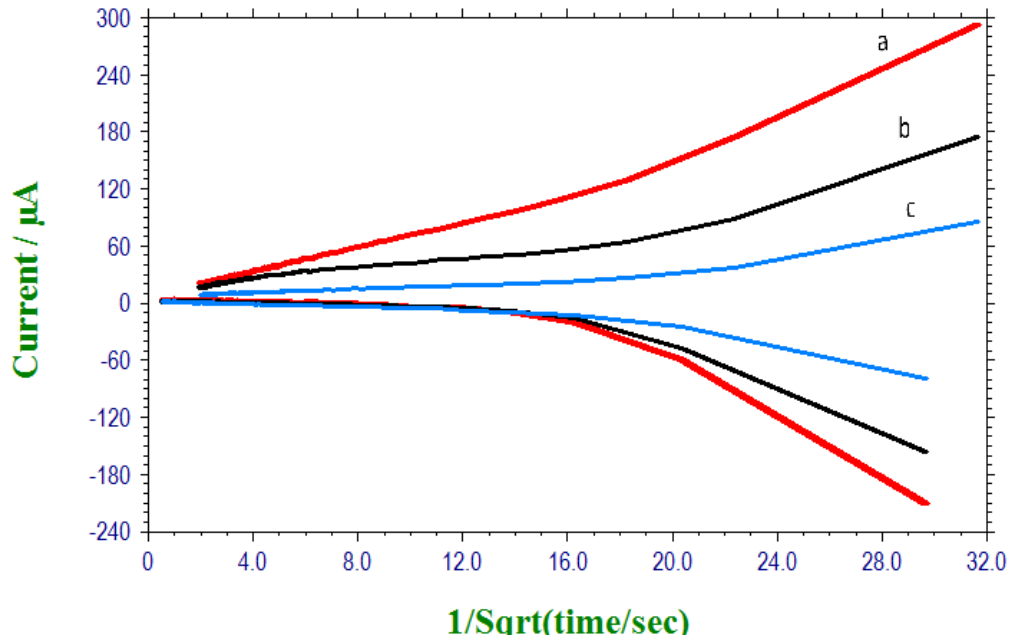
Şekil 4.15 Ligandın farklı pH'larda CHI cihazında kaydedilen kronoamperometri bulguları ile çizilen i - t^{-1/2} grafiği (a) pH=2,00; (b) pH=4,00; (c) pH=6,00.
