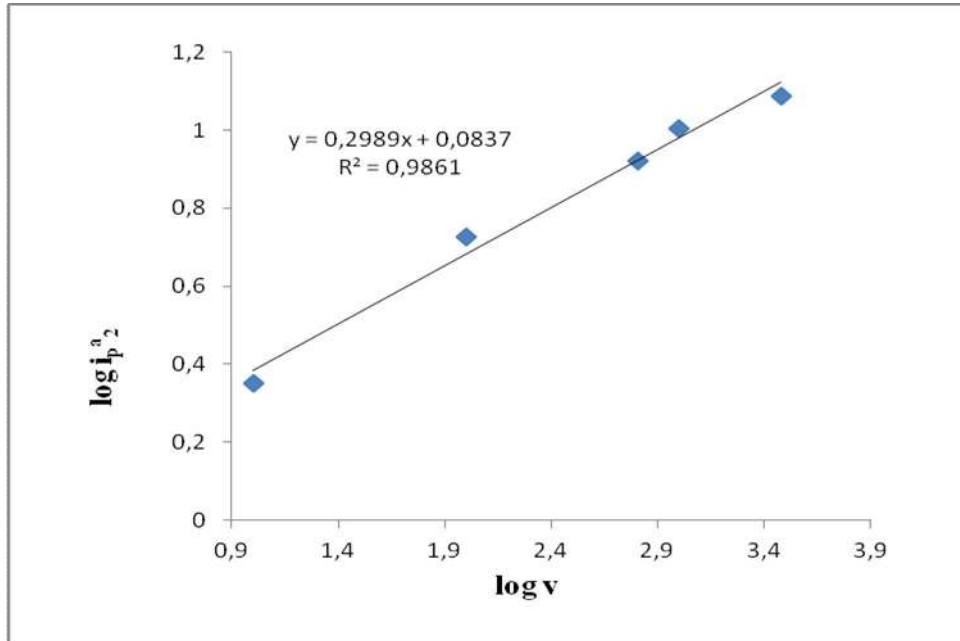
Şekil 5.10 NiL 2 kompleksinin GC elektrotta pH=2,80'de katodik pik için farklı tarama hızlarında alınan dönüşümlü voltamogramlarından elde edilen \log i_p^1 - \log v grafiği
