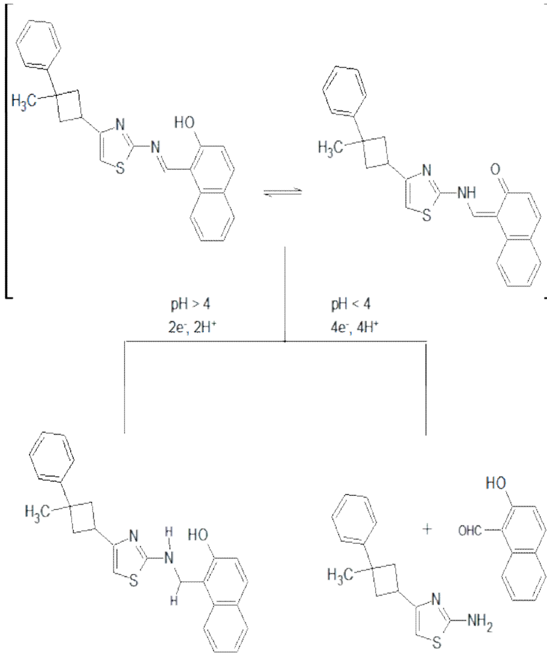
Şekil 5.13 LH'n asidik ve bazik ortamdaki elektrokimyasal indirgenme reaksiyon mekanizması
