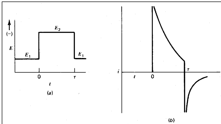
Şekil 2.8 (a) Krono tekniklerinde elektroda uygulanan potansiyel profili (b) Kronoamperometride oluşan akımın zamanla değişimi
