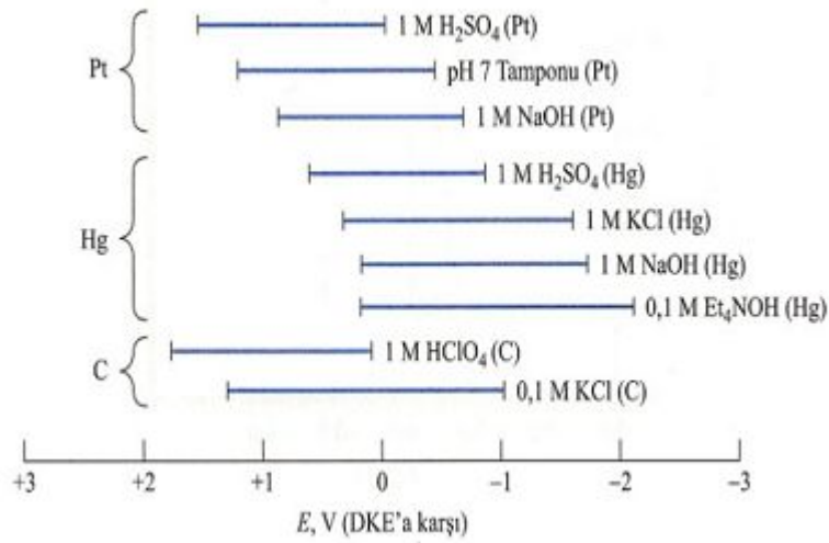
Şekil 2.3 Üç tip elektrot için çeşitli destek elektrolitlerin potansiyel aralıkları
