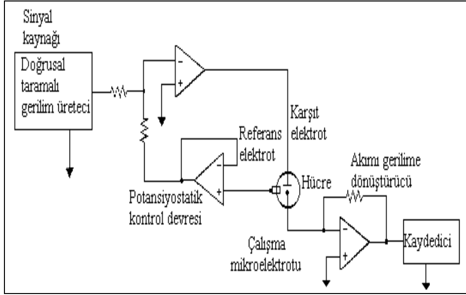
Şekil 2.2 Doğrusal taramalı voltametrik ölçümler yapmak için kullanılan bir cihazın bileşenleri.
