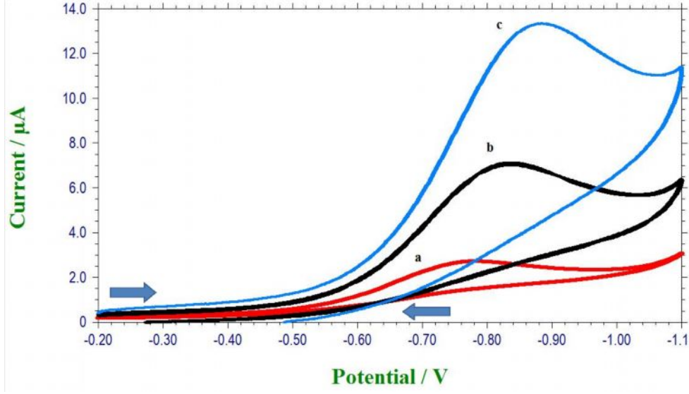
Şekil 4.3 Ligandın pH=4,00’de farklı tarama hızlarında CHI cihazında kaydedilen dönüşümlü voltamogramı v: mVs -1 (a):10; (b): 100; (c):1000.
