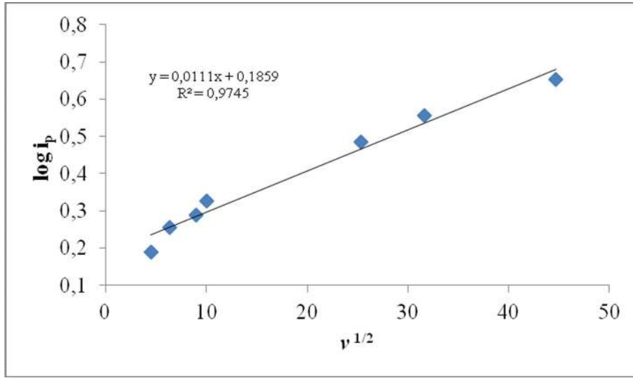
Şekil 5.3 CuL 2 kompleksinin GC elektrotta asidik pH’da (pH=2,00) farklı tarama hızlarında kaydedilen dönüşümlü voltamogramlarından elde edilen \log v - v^{1/2} grafiği
