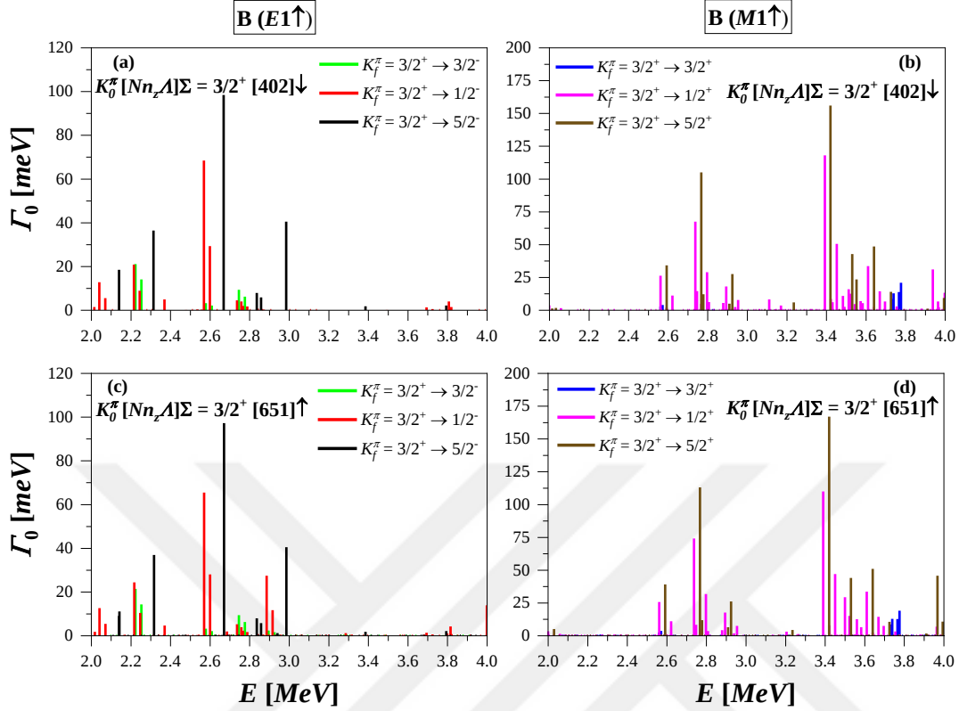
Şekil 3.2. 153 Sm çekirdeği için teorik olarak elde edilen düşük enerjili dipol uyarılmalarına ait radyasyon genişliklerinin 2-4 MeV enerji aralığındaki dağılımı (a) 153 Sm çekirdeğinde 3/2[402] taban durum konfigürasyonu için TGI-QPNM ile hesaplanan \Gamma_0(E1\uparrow) radyasyon genişliklerinin enerji spektrumundaki dağılımı (b) 153 Sm çekirdeğinde 3/2[402] taban durum konfigürasyonu için RI-QPNM ile hesaplanan \Gamma_0(M1\uparrow) radyasyon genişliklerinin enerji spektrumundaki dağılımı. (c) 151 Sm çekirdeğinde 3/2[651] taban durum konfigürasyonu için TGI-QPNM ile hesaplanan \Gamma_0(E1\uparrow) radyasyon genişliklerinin enerji spektrumundaki dağılımı (d) 153 Sm çekirdeğinde 3/2[651] taban durum konfigürasyonu için RI-QPNM ile hesaplanan \Gamma_0(M1\uparrow) radyasyon genişliklerinin enerji spektrumundaki dağılımı.
