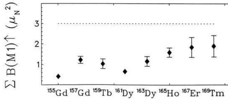
Şekil 1.3. Bazı tek kütle numaralı deforme çekirdeklerde düşük enerji bölgesinde deneysel olarak belirlenmiş toplam indirgenmiş M1 geçiş ihtimalleri. Bu değerler belirlenirken deneyde gözlenen tüm düşük enerjili geçişlerin M1 karakterli oldukları kabul edilmiştir [36].
