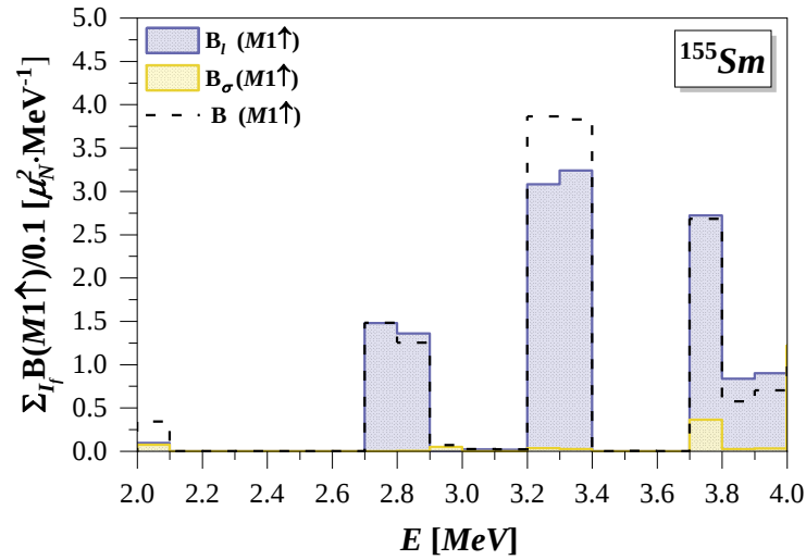
Şekil 3.7. ^{155}\text{Sm} çekirdeğinde 2-4 MeV enerji aralığındaki spin ve orbital B(M1 \uparrow) spektrumları. M1 operatörünün spin ve orbital kısımlarından gelen katkılar sırasıyla sarı ve mavi renk ile gösterilmiştir.
