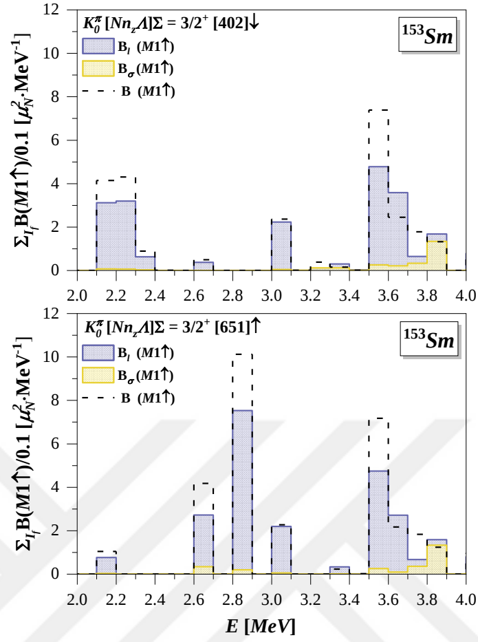
Şekil 3.6. ^{153}\text{Sm} çekirdeğinde 2-4 MeV enerji aralığındaki spin ve orbital B(M1 \uparrow) spektrumları. M1 operatörünün spin ve orbital kısımlarından gelen katkılar sırasıyla sarı ve mavi renk ile gösterilmiştir.
