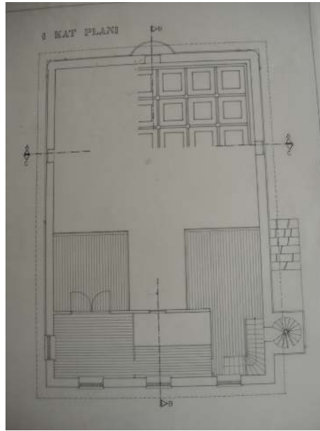
Şekil 3.5 Bandırmalı tekkesi 1. kat planı, MSGSÜ.
