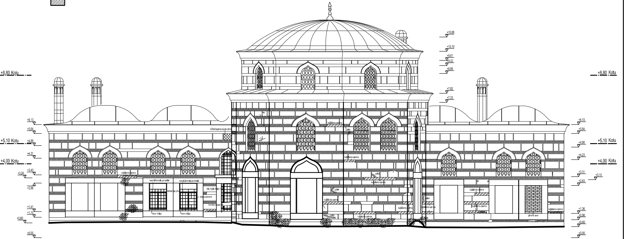
GÜNEY CEPHESİ ÖLÇEK :1/50
