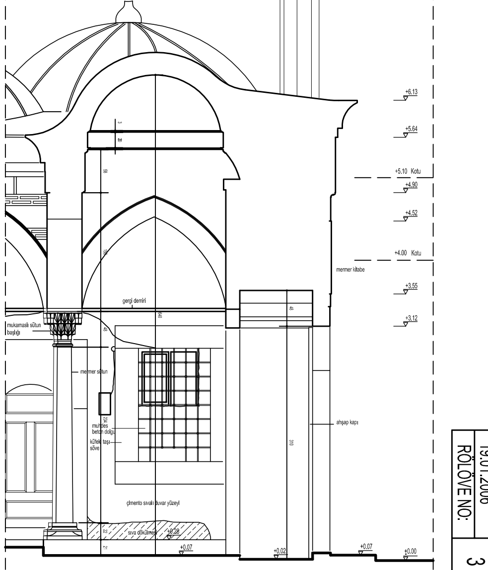
GİRİŞ KAPISI KESİTİ ÖLÇEK : 1/20
