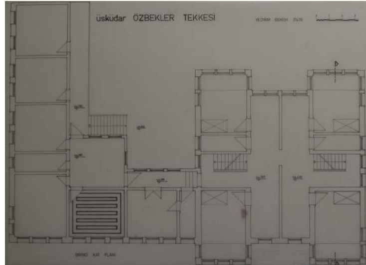
Şekil 3.19 Özbekler Tekkesi harem ve selamlık birinci kat planı, Bekem, MSGSÜ.
