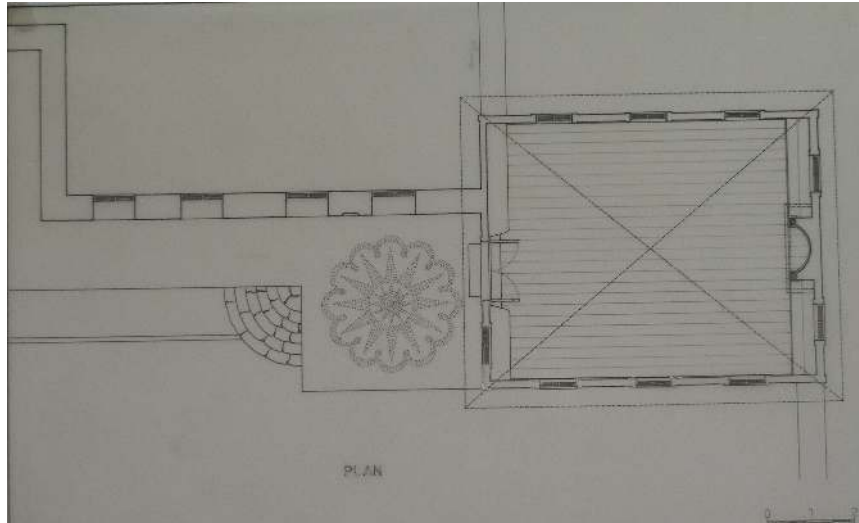
Şekil 3.17 Özbekler Tekkesi mescit planı, Bekem, MSGSÜ.
