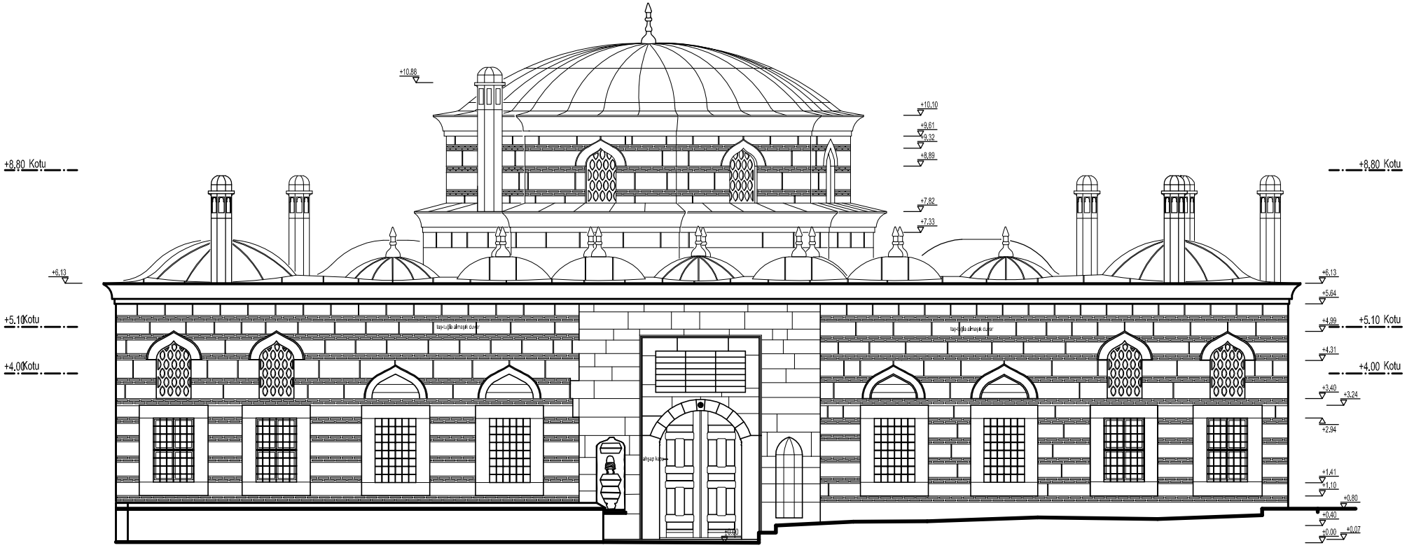
KUZEY CEPHESİ ÖLÇEK :1/50
