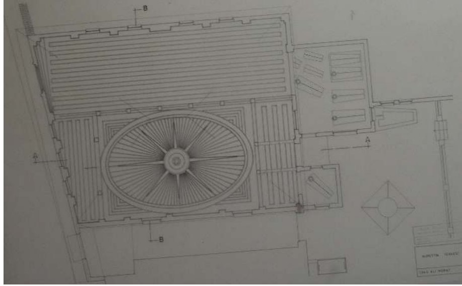
Şekil 3.15 Nureddin Cerrahi tekkesi tavan planı, Murat, 1976, MSGSÜ.
