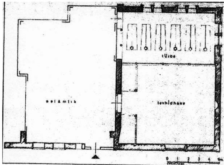
Şekil 3.21 Sertarikzade Tekkesi planı, DBİA, 1994, c.7.
