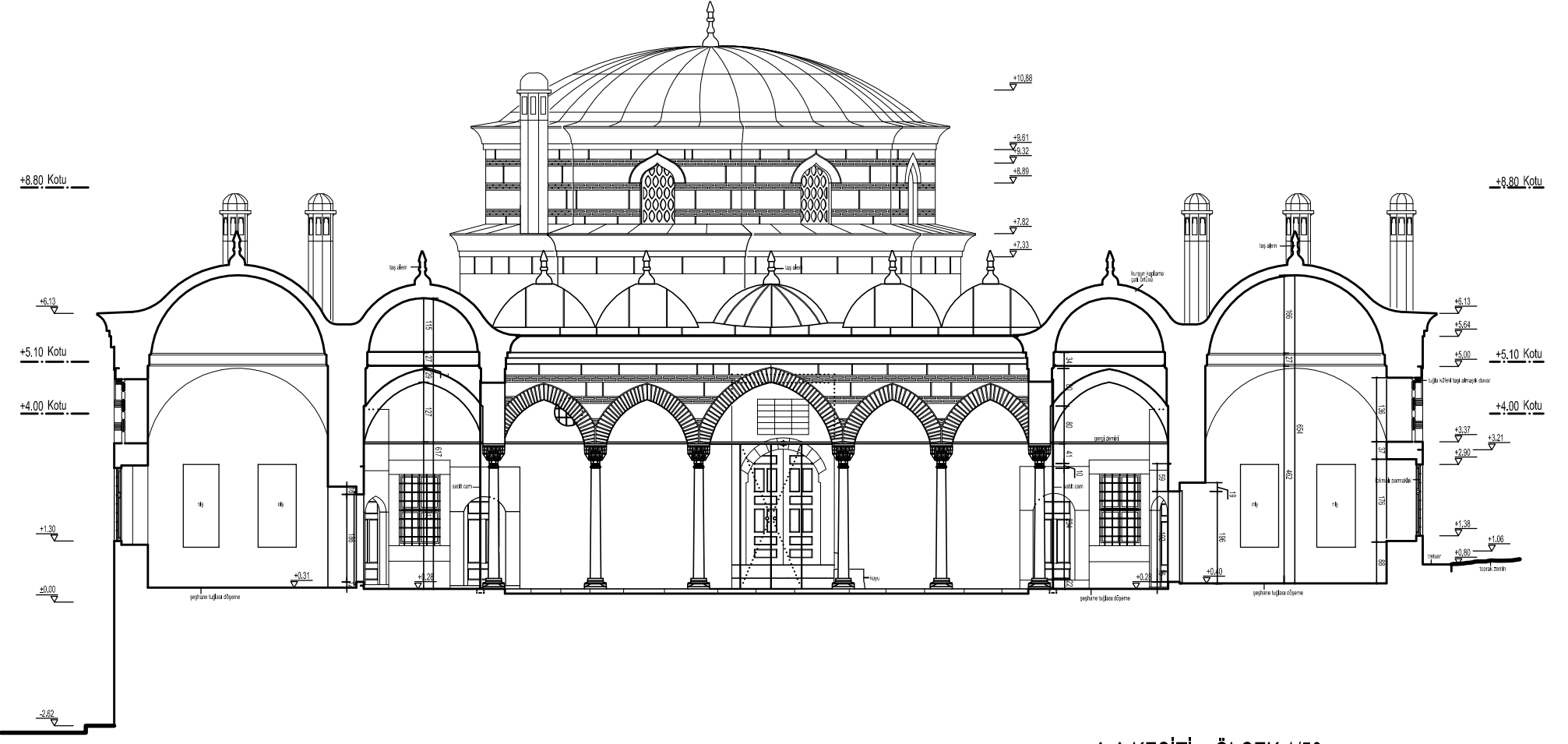
A-A KESİTİ ÖLÇEK:1/50
