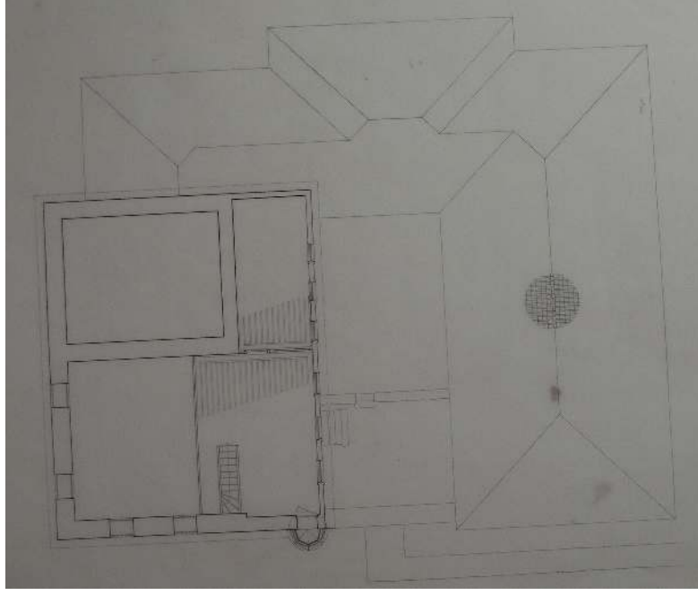
Şekil 3.29 Tahirağa Tekkesi çatı planı, Özer, MSGSÜ, 1983.
