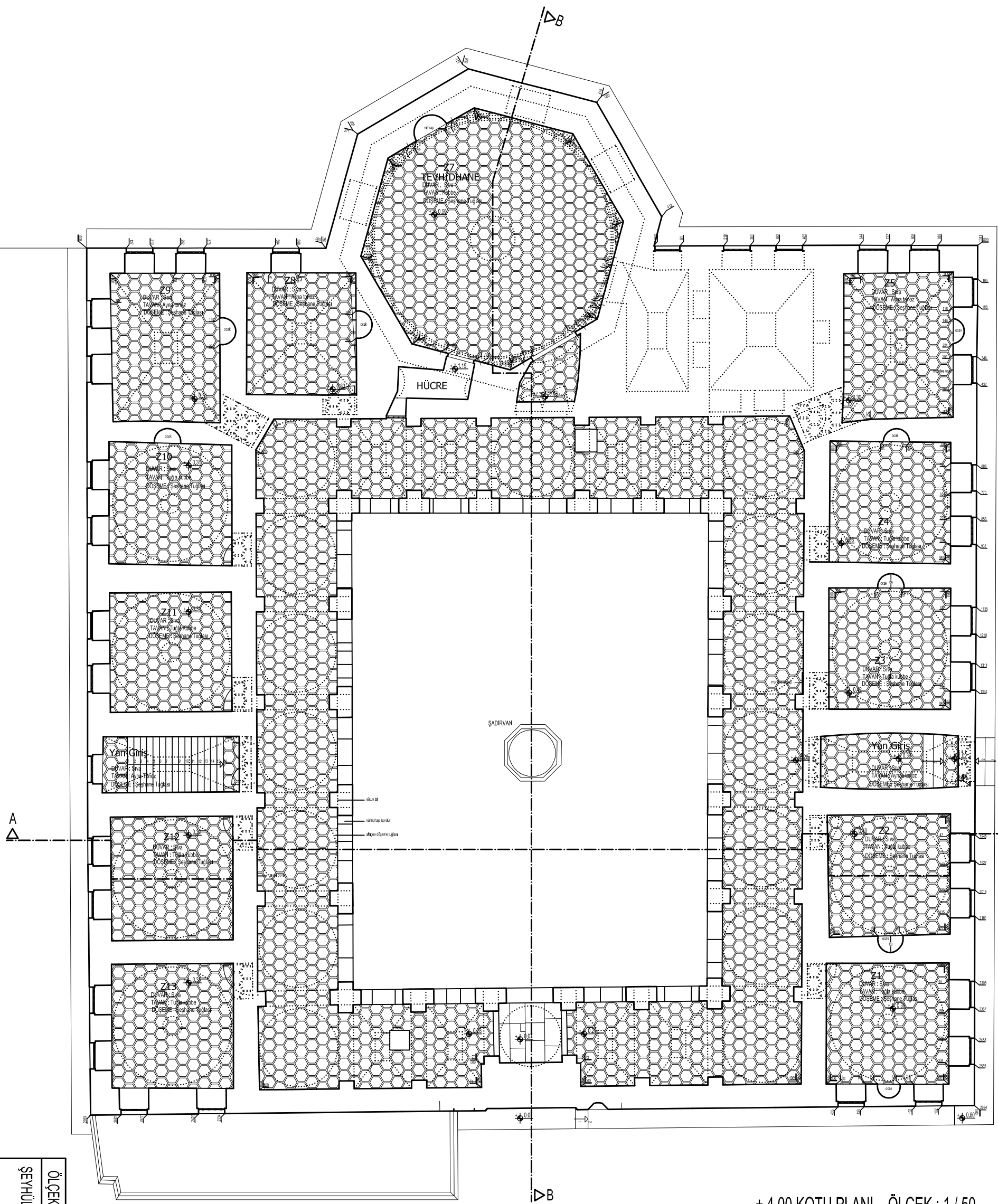
+ 4.00 KOTU PLANI ÖLÇEK : 1 / 50
