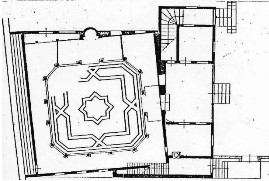
Şekil 3.6 Hasırcızade Tekkesi zemin kat planı, Başkır, 1990, İTÜ
