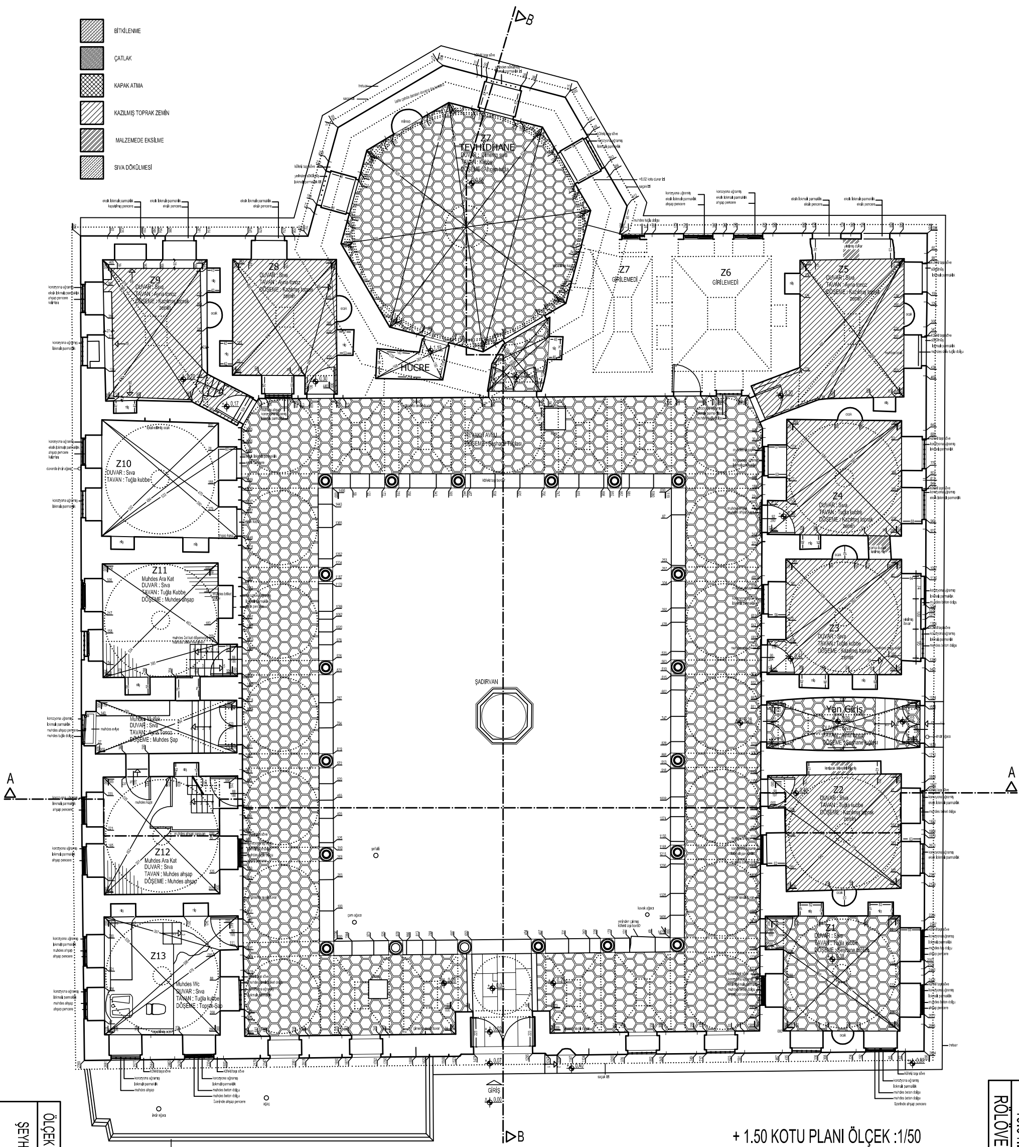
Ek 3.3 Şeyhülislâm Tekkesi, + 1.50 Kotu Planı - Rölöve
