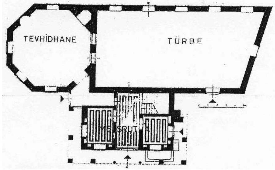
Şekil 3.24 Şeyh Atâ Tekkesi planı, İşli, 1998, YTÜ.
