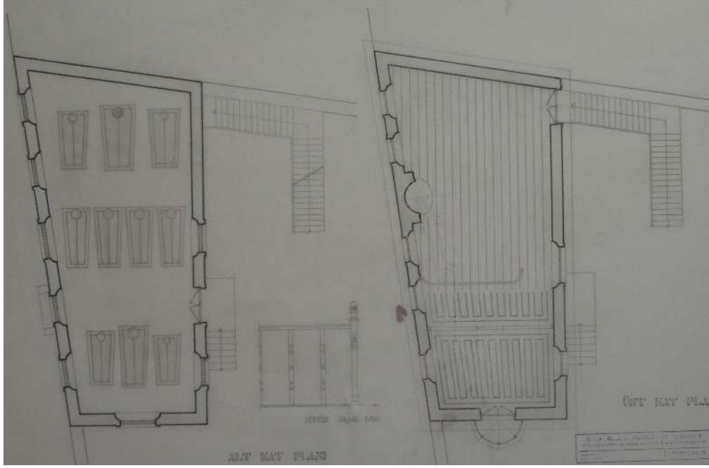
Şekil 3.31 Üsküdar Mevlevihanesi zemin ve birinci kat planları, Tüzün, Oruç, MSGSÜ, 1975.
