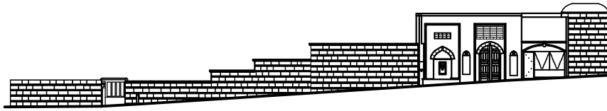
DIŞ AVLU KUZAY CEPHESİ ÖLÇEK : 1 / 200
