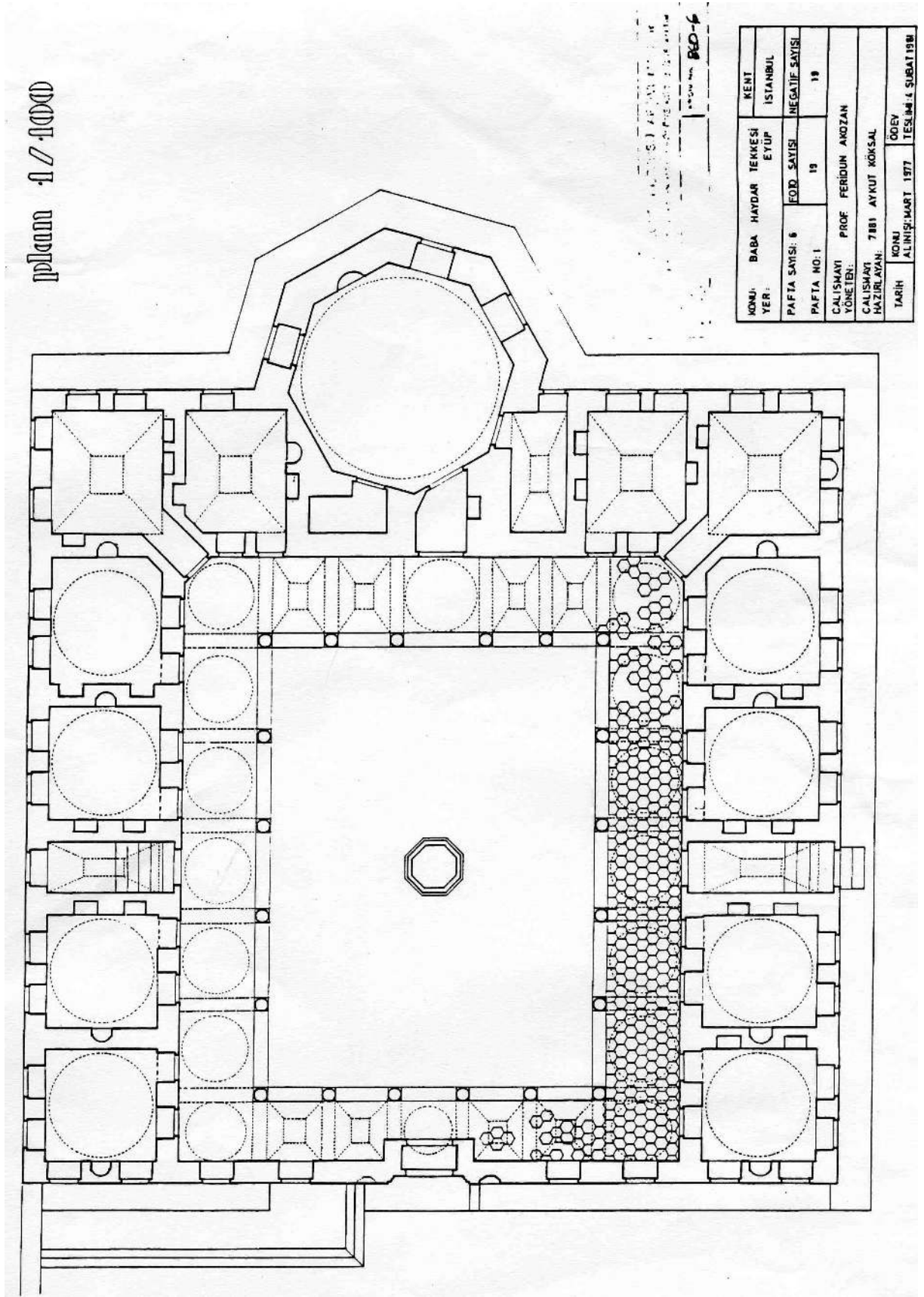
Şekil 5.6 Şeyhülislam Mustafa Efendi Tekkesi Rölövesi, Köksal 1981.
