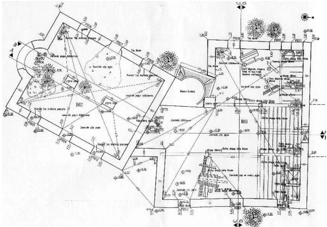
Şekil 3.9 İzzet Paşa Tekkesi bodrum planı, Bay, 2004, İTÜ.
