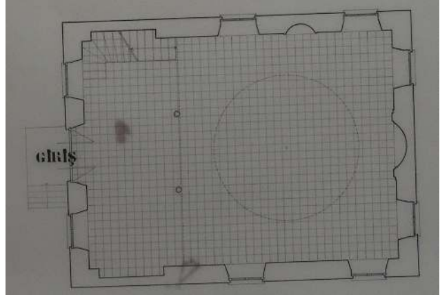
Şekil 3.23 Şazeli tekkesi planı, Türkkan, Güler, MSGSÜ.
