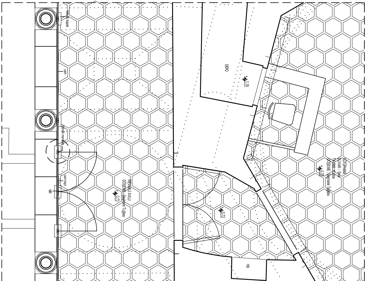
+ 1.50 KOTU PLANI ÖLÇEK :1/20
