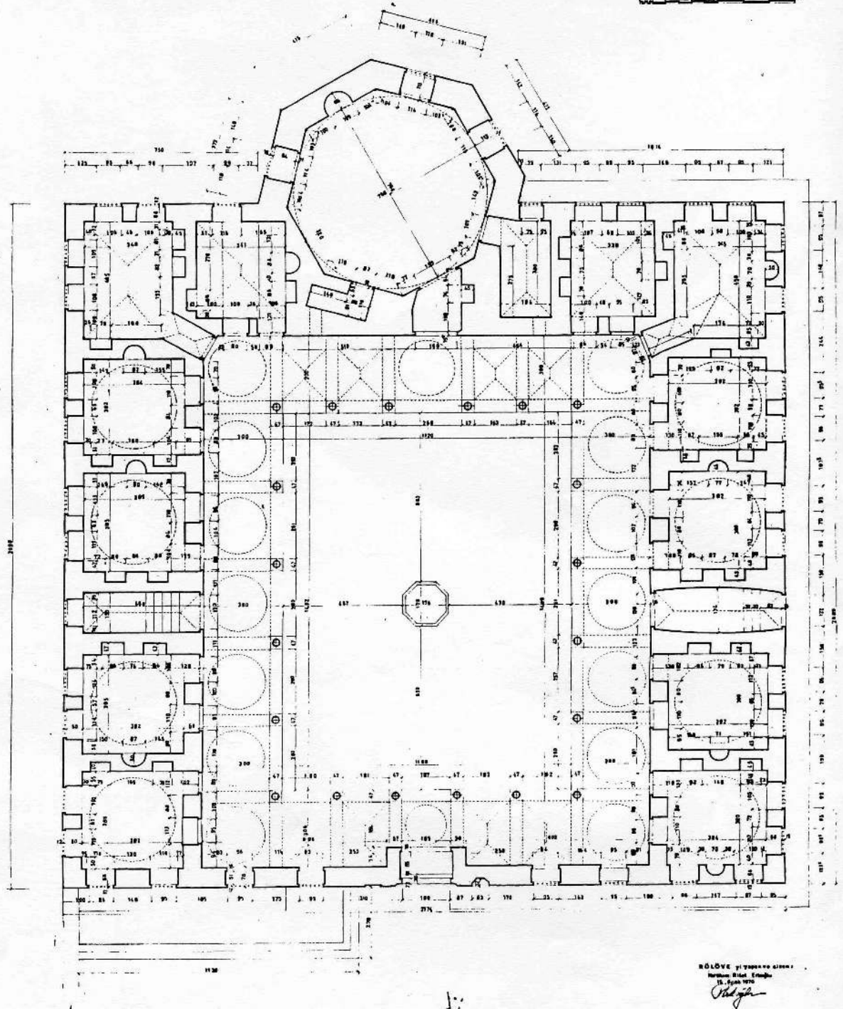
Şekil 5.5 Şeyhülislam Mustafa Efendi Tekkesi Rölövesi, Erkoğlu 1970.
