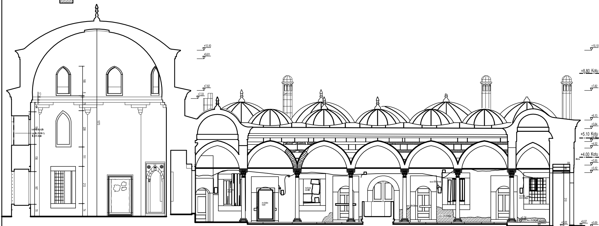
B-B KESİTİ ÖLÇEK :1/50
