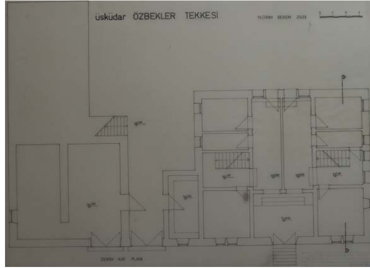
Şekil 3.18 Özbekler Tekkesi harem ve selamlık zemin kat planı, Bekem, MSGSÜ.
