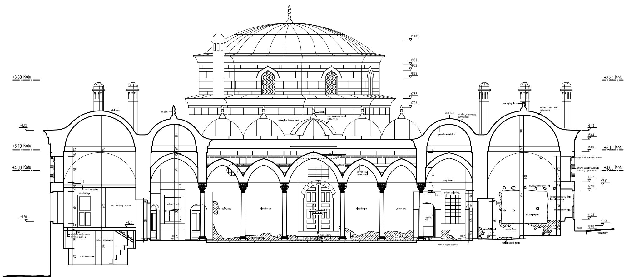
A-A KESİTİ ÖLÇEK :1/50
