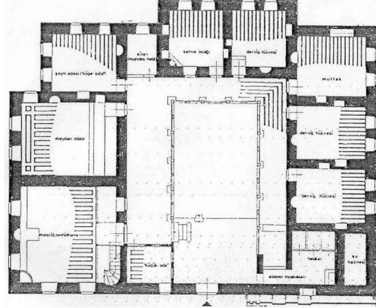
Şekil 3.28 Tahirağa Tekkesi planı, İSTA.
