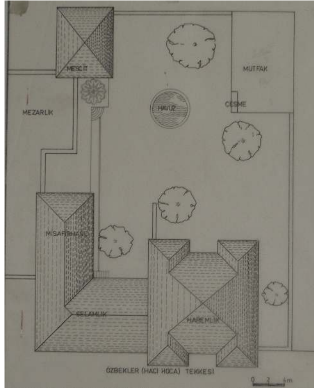
Şekil 3.16 Özbekler Tekkesi vaziyet planı, Bekem, MSGSÜ.
