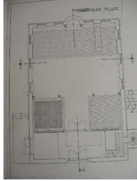
Şekil 3.4 Bandırmalı tekkesi zemin kat planı, MSGSÜ.
