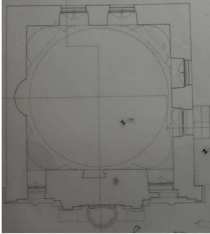
Şekil 3.11 Kalenderhane Tekkesi planı, Küstü, 2005, MSGSÜ.
