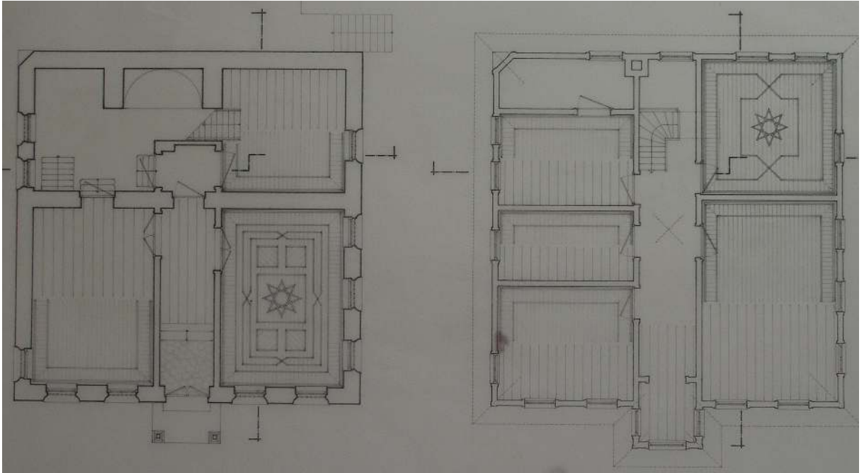
Şekil 3.32 Üsküdar Mevlevihanesi şeyh evi zemin ve birinci kat planları, Tüzün, Oruç, MSGSÜ, 1975.
