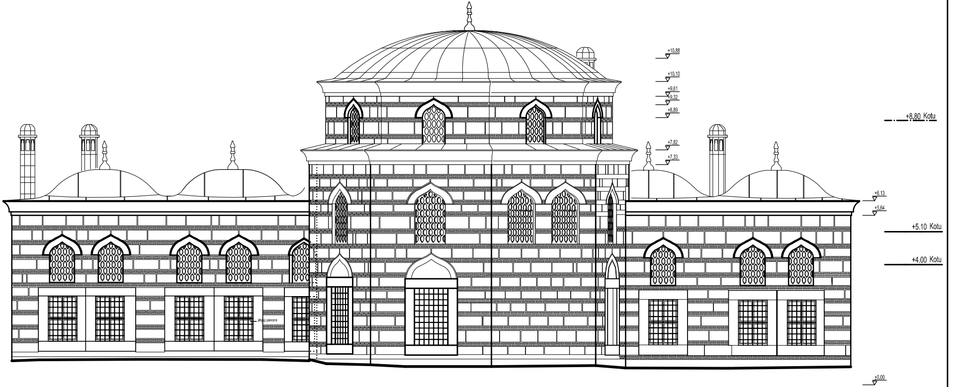
GÜNEY CEPHESİ ÖLÇEK:1/50
