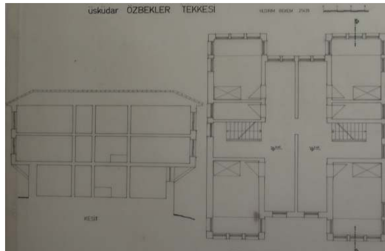
Şekil 3.20 Özbekler Tekkesi harem ikinci kat planı-kesit, Bekem, MSGSÜ.
