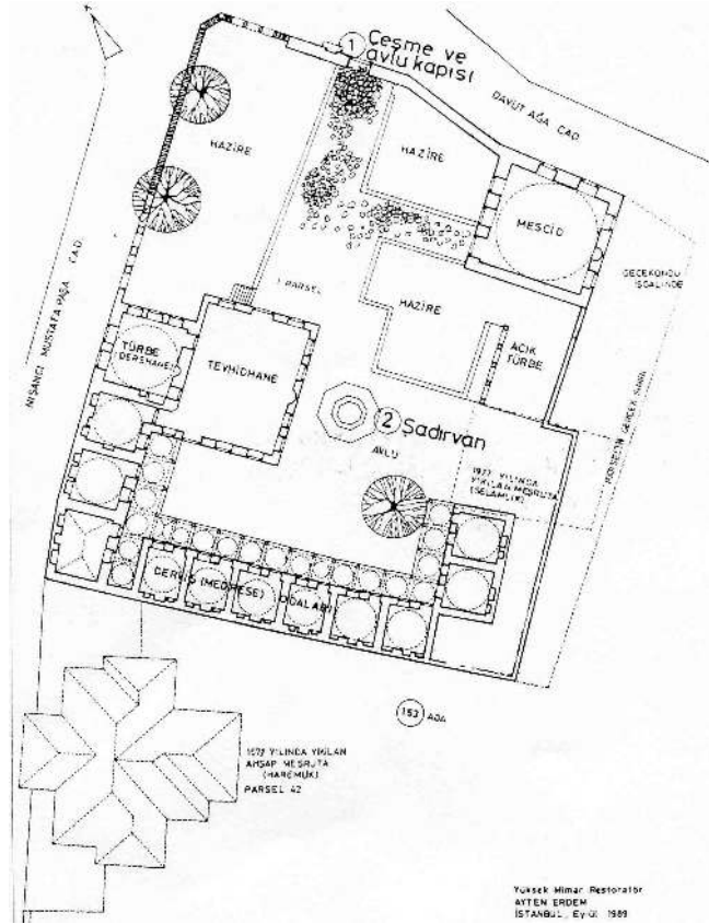
Şekil 3.27 Şeyh Murat Tekkesi vaziyet planı, Erdem, 1989, II.Eyüp Sultan Sempozyumu.
