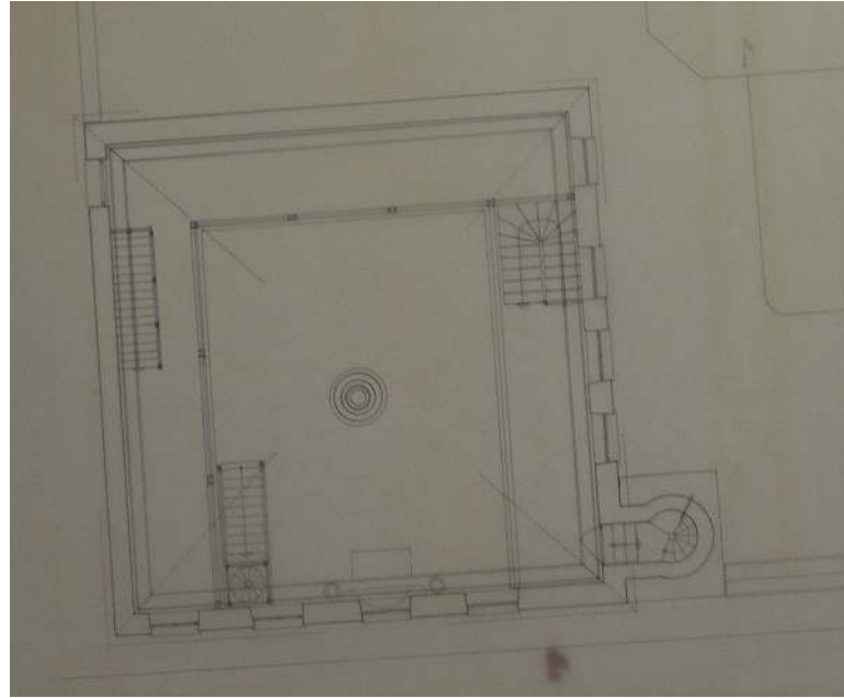
Şekil 3.26 Şeyh Fenai Efendi Tekkesi mahfil planı, Bozkurt, Seymen, MSGSÜ.
