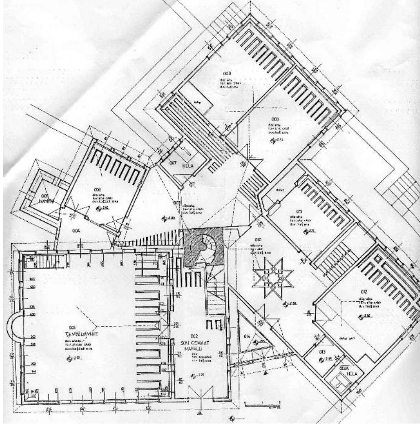
Şekil 3.12 Kaşgari Tekkesi planı, Demirel.
