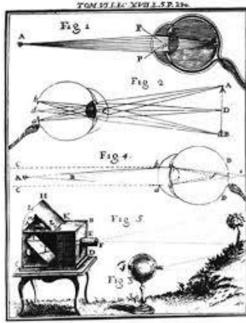
Görsel 8: İnsan Gözü ve Karanlık Kutu
