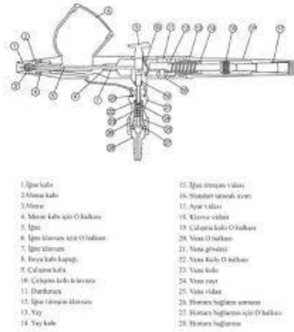
Görsel 11: TG Model Havalı Püskürtme (Airbrush) Mekanizması.
