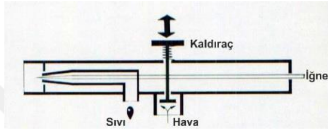
Görsel 10: Havalı Püskürtme Aletinin Çizimi
