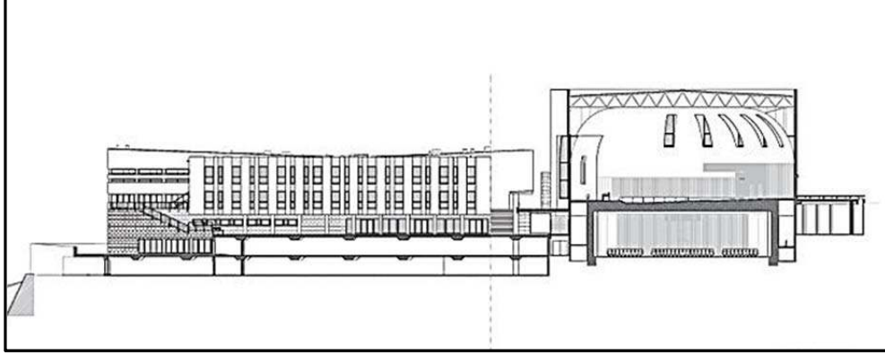
řekil 3.98. Boa Nova Kilisesi Kesiti (Url-33)
