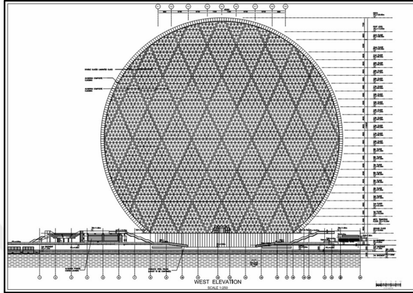
Şekil 3.38. Yapının Batı Görünüşü (Url-16)
