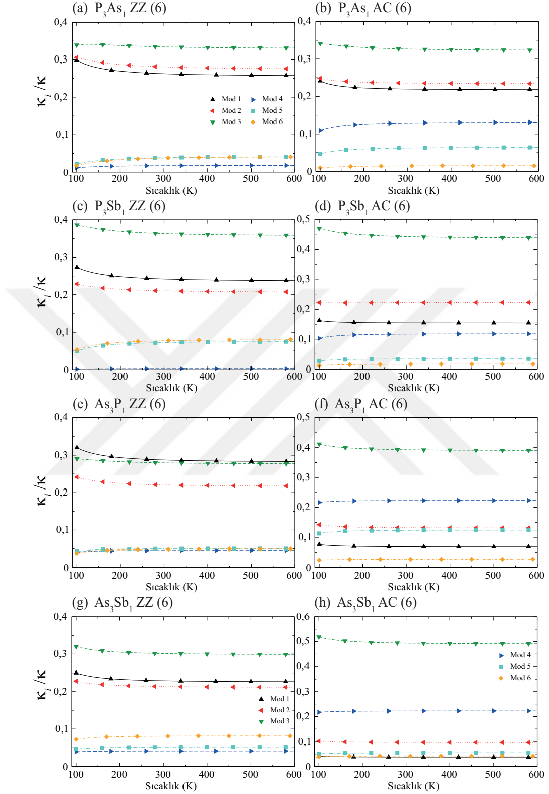
Şekil 6.16: %25 katkılı ikili bileşiklerin akustik ve düşük frekanslı optik modlarının normalize edilmiş olarak ZZ ve AC yönlerinde termal iletkenliğe katkıları.
