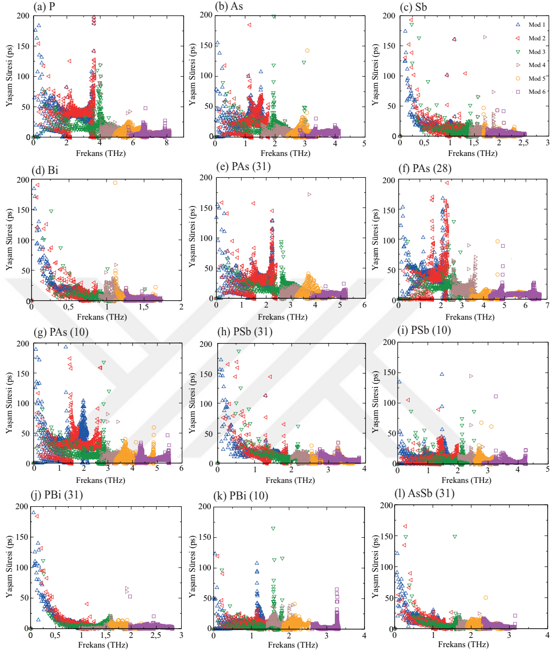
Şekil 6.13: T = 300\text{ K} için (a)-(d) katkısız yapıların, (e)-(r) %50 katkılı bileşiklerin ve (s)-(v) %25 katkılı bileşiklerin frekansın fonksiyonu olarak fonon yaşam süreleri.
