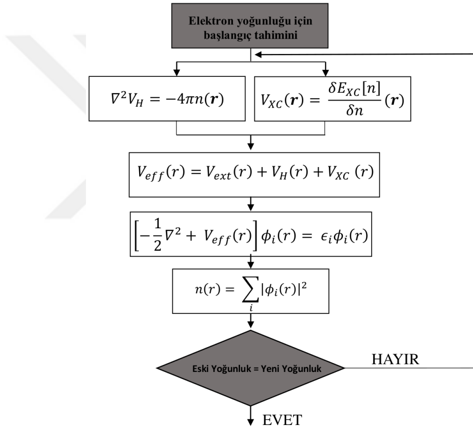
Şekil 3.1: Kohn-Sham denkleminin iteratif çözüm şeması.
