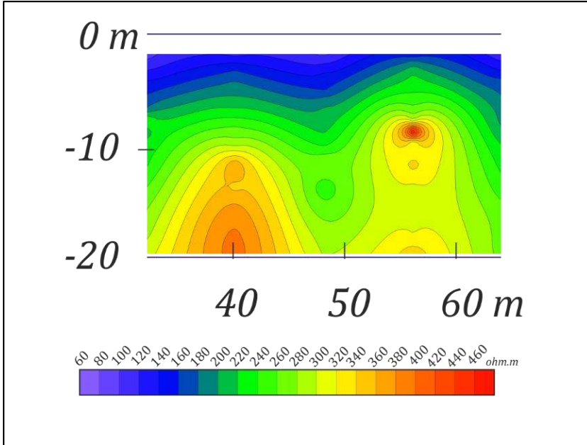
Şekil 4.30. HAT 2’de gerçekleştirilen DES ölçüm sonuçlarının SURFER ile oluşturulmuş kesiti
