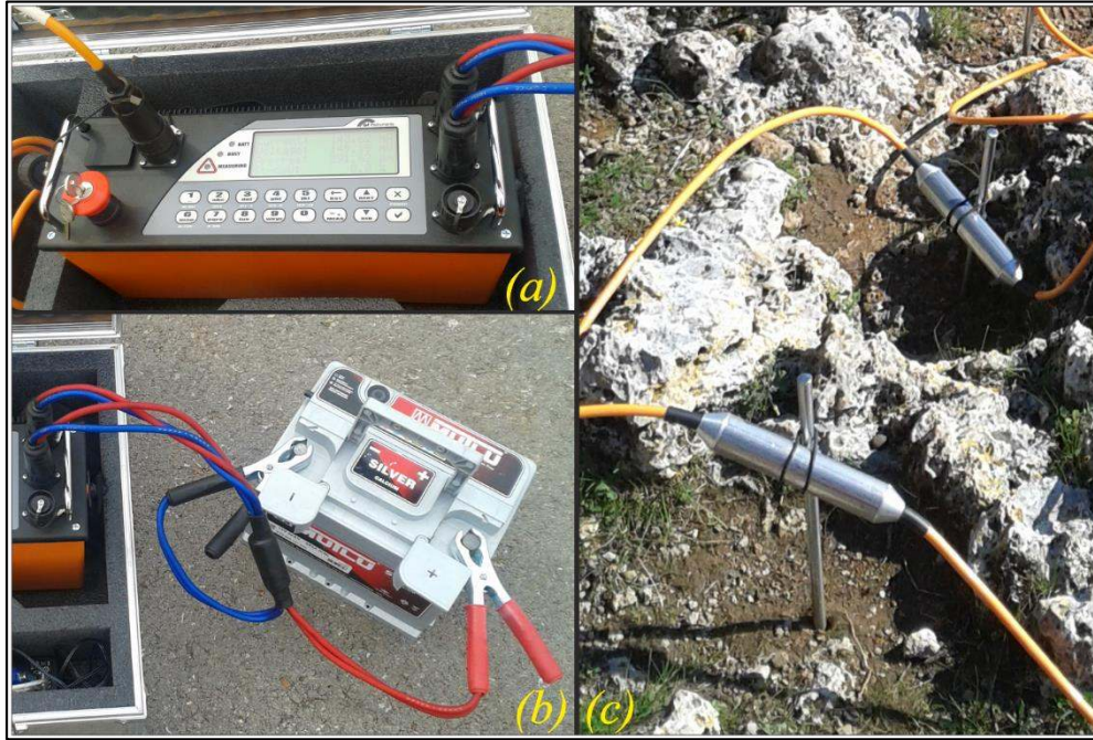
Şekil 3.1. (a) ARES çok kanallı rezistivite cihazı, (b) rezistivite cihazının akü bağlantısı, (c) akıllı kabloların elektrot bağlantısı
