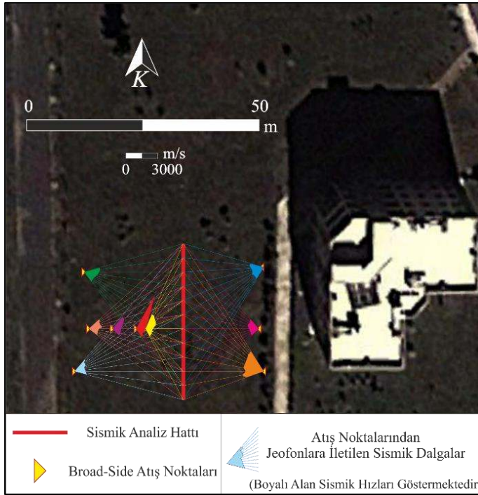
Şekil 4.18. Kampüs alanı 1 numaralı çalışma bölgesinde gerçekleştirilen Broad-Side analizinden elde edilen sismik hızların ve sismik dalgaların harita üzerinde gösterilmesi
