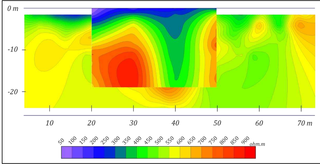
Şekil 4.42. Kampüs alanı 2 numaralı çalışma bölgesinde gerçekleştirilen Wenner-Alfa ve DES ölçüm sonuçlarının SURFER ile oluşturulmuş kesitlerinin karşılaştırılması
