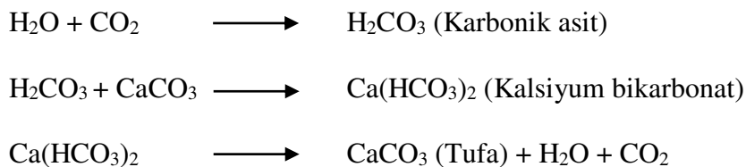
Şekil 2.10. Karst oluşumunu gösteren şema
