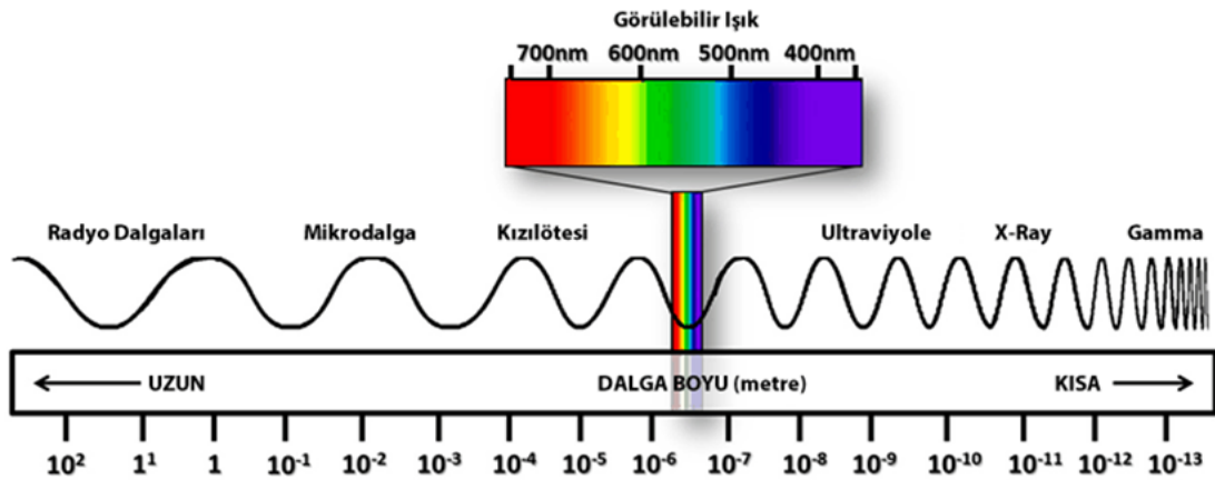
Şekil 2.1. Elektromanyetik Spektrum [44].
