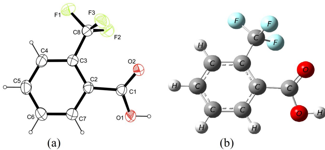
Şekil 4.1.a) Atom sayı şemasını gösteren tek kristal moleküler yapı, b) 2-TFMB için temel durumdaki B3LYP/6-31++G (d,p) metodu ile optimize teorik moleküler yapı şeması [76].
