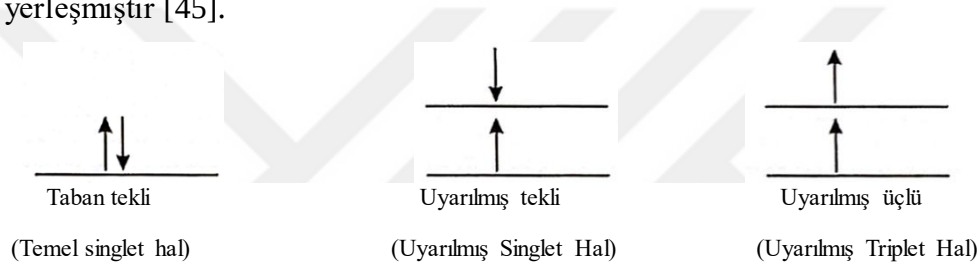
Şekil 2.2. Uyarılmış Tekli ve üçlü durumlar [45].
