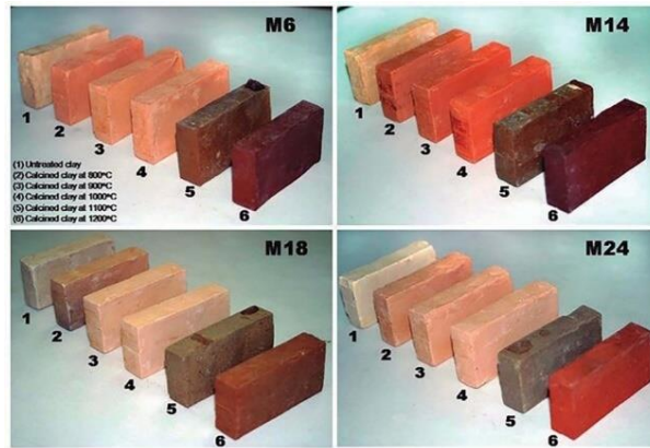
Görsel 2.22. Farklı Derecelerde Pişirilen Dört Farklı Çamurda Görülen Renk Değişimleri (http-227)
