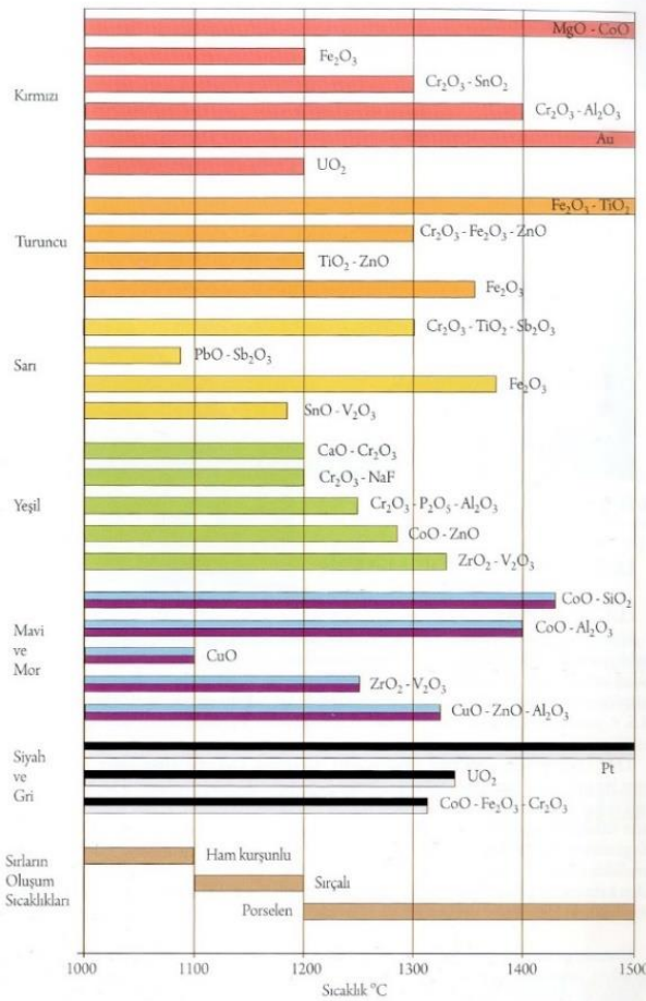
Görsel 2.27. Sırlı Boyaların Kullanım Sıcaklık Aralıkları (Mete, 2020, s. 321)
