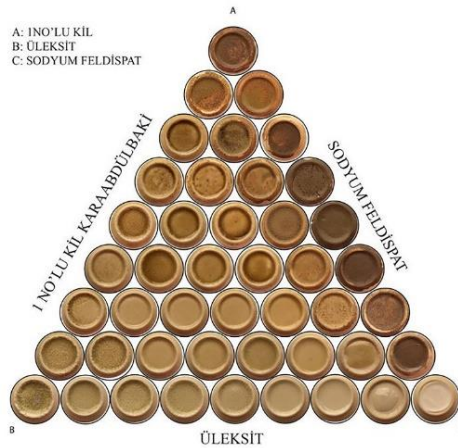
Görsel 2.36. Kocaeli İli Yöre Killeri ile Oluşturulan Üçlü Diyagramlar ve 1200°C Sıcaklıkta Pişirilmiş Deney Sonuçları (Sülün, 2021, s. 48)
