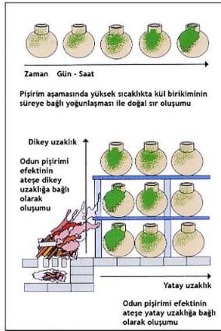
Görsel 2.24. Fırında Uzaklığa ve Süreye Bağlı Olarak Bünyelerin Üzerinde Oluşan Kül Birikimi (Özyurt, 2008, s. 64)
