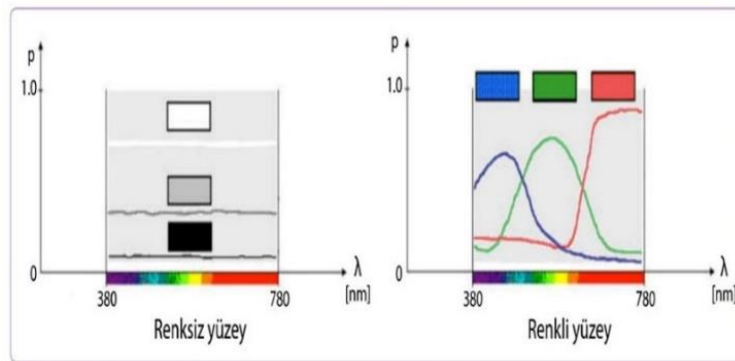
Görsel 1.14. Renksiz ve Renkli Yüzeylerin Yansıtma Çarpanları Eğrisi (http-19)
