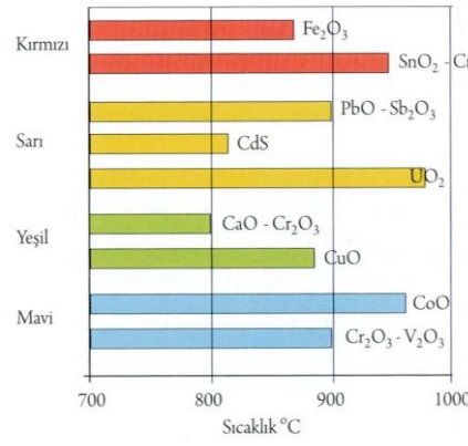
Görsel 2.26. Sırlı Boyaların Kullanım Sıcaklık Aralıkları (Mete, 2020, s. 320)
