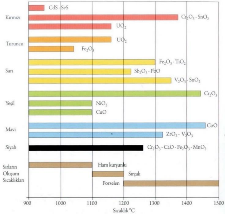
Görsel 2.25. Sırıçi Boyalarının Kullanım Sıcaklık Aralıkları (Mete, 2020, s. 320)
