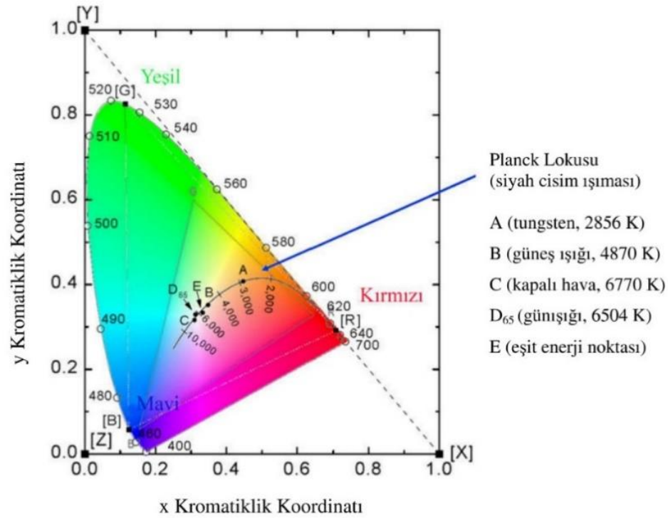
Görsel 1.8. CIE Kromatiklik Diyagramı (http-14)
