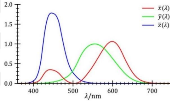
Görsel 1.12. CIE'nin Tayfsal Üçrenksel Bileşenleri (http-17)
