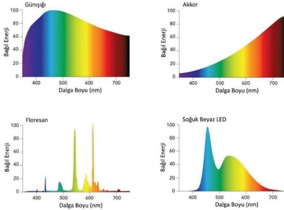
Görsel 1.7. Farklı Işıkların Tayf Eğrileri (http-13)
