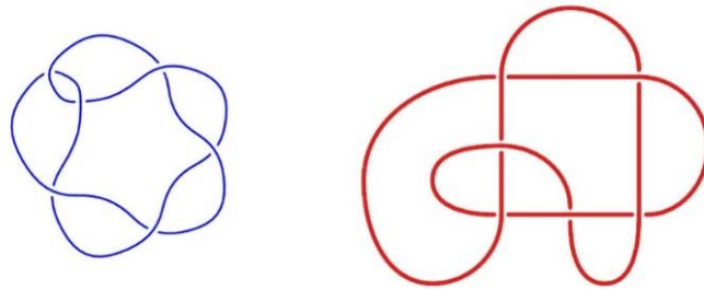
Görsel 4.1. 6-1 Düğümü'nün İki Farklı Görünüm Diyagramı (http-312)
