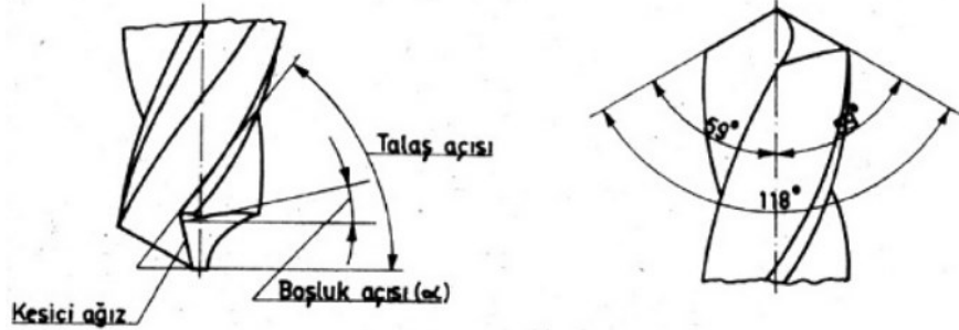
3.13. Kesici takım uc açılarının gösterimi [39]
