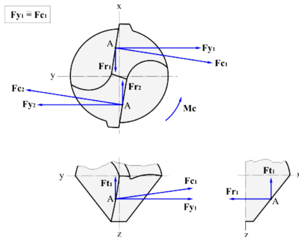
Şekil 3.4. Matkap ucuna etkileyen kuvvetler [22]
