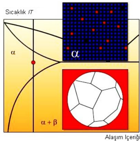
Şekil 2.3. Çözeltiliye alma işlemi sonucunda tek faz halindeki katı çözelti [21]
