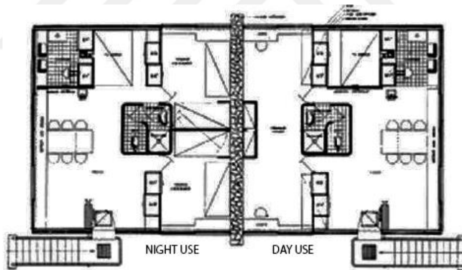
Figure 3.1. Maisons Loucheur, Le Corbusier, 1928-1929 (Živković, Keković & Kondić, 2014)
