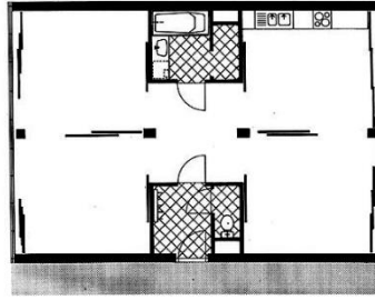
Figure 2.10. Grieshofgasse, Vienna ("Wohnbau Grieshofgasse", 1996)
