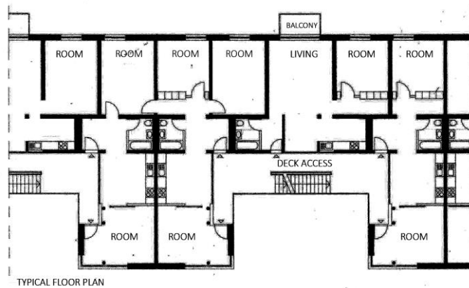
Figure 2.3. Überbauung Hellmutstrasse by ADP Architektur und Planung (A.D.P. Walter Ramseier, 1991)
