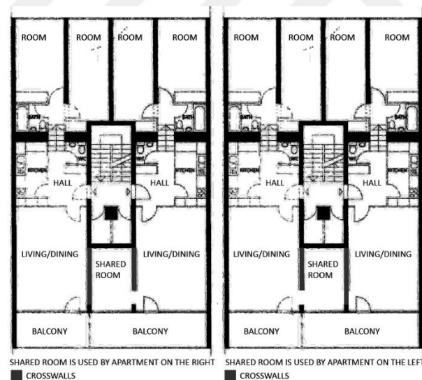
Figure 2.7. Asemwald by O. Jäger, U. Müller, H. Papst, H. Wirth (Jager & Müller, 1964, p. 504).
