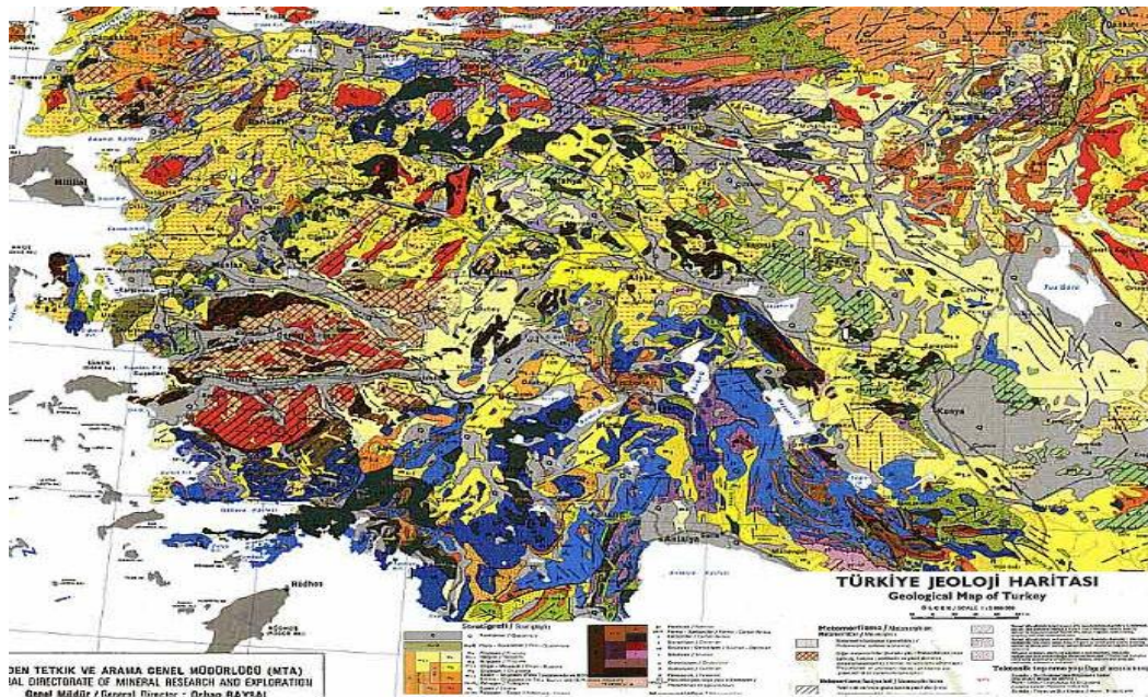
Şekil 2.1. Ege Bölgesi' nin jeoloji haritası (MTA,2002).
