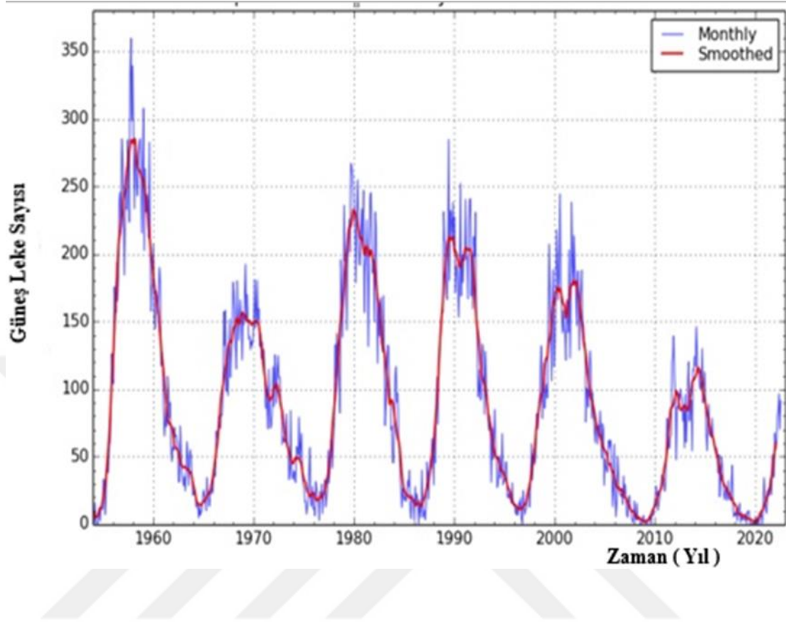
Şekil 2.15. Son altı döngünün verileriyle oluşturulmuş uzun dönemli Güneş leke aktivitesi. Son altı döngü için aylık ortalama Güneş lekesi sayısı (mavi) ve 11 adımda düzeltilmiş Güneş lekesi sayısı (kırmızı) 23 .
