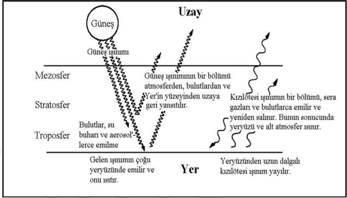
Şekil 2.19. Sera etkisinin şematik gösterimi (WHO, 1996'ya göre Türkes, 2000; Türkes vd. 2000) 31 .
