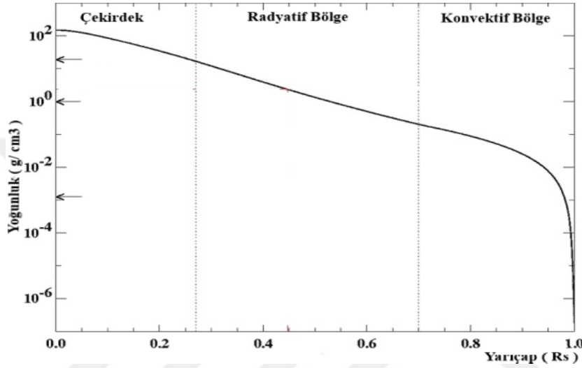
Şekil 2.3. Güneş'in merkezinden yüzeyine doğru yarıçap-yoğunluk değişimi 9
