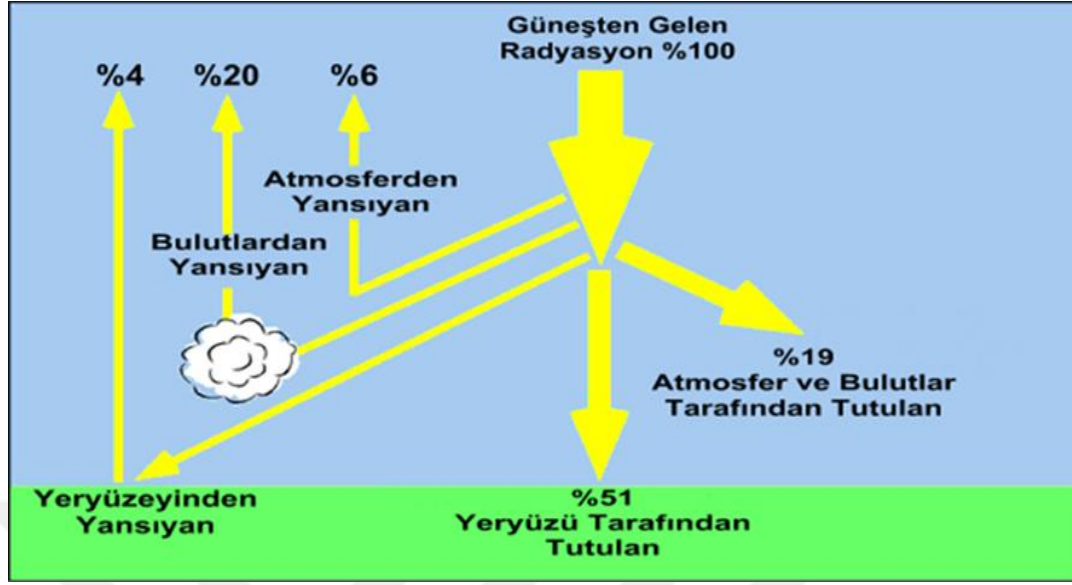
Şekil 2.20. Güneş'ten Gelen Radyasyonun Tutulması ve Yansımaları 34 .
