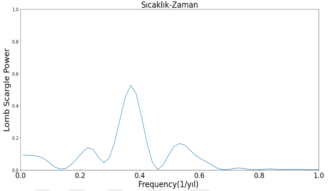
Şekil 3.7. Veriler üzerinde yapılan Fourier Analizi sonucu elde edilen grafikler. (a) F_{10.7} Radyo akısının güç spektrumu, (b)Sunspot (Güneş leke sayısı) sayısı güç spektrumu, (c)Sıcaklık değerinin zamana bağlı güç spektrumu.
