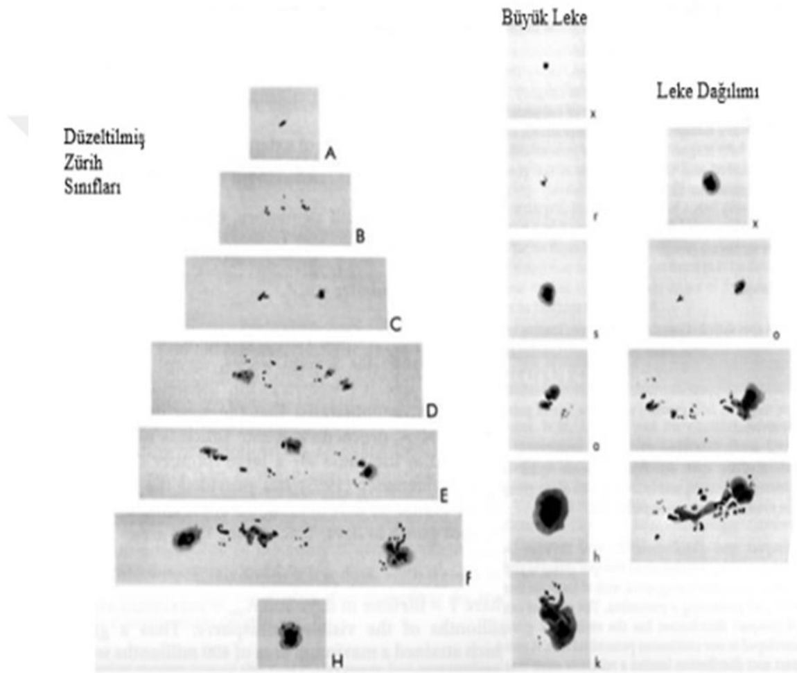
řekil 2.12. Modifiye edilmiř Z rich leke sınıflandırması 18 (McIntos Sınıflandırması; McIntos 1990) .
