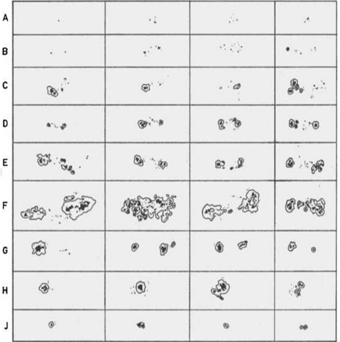
Şekil 2.11. Zürich leke grubu sınıflandırması (Bray vd. 1964).
