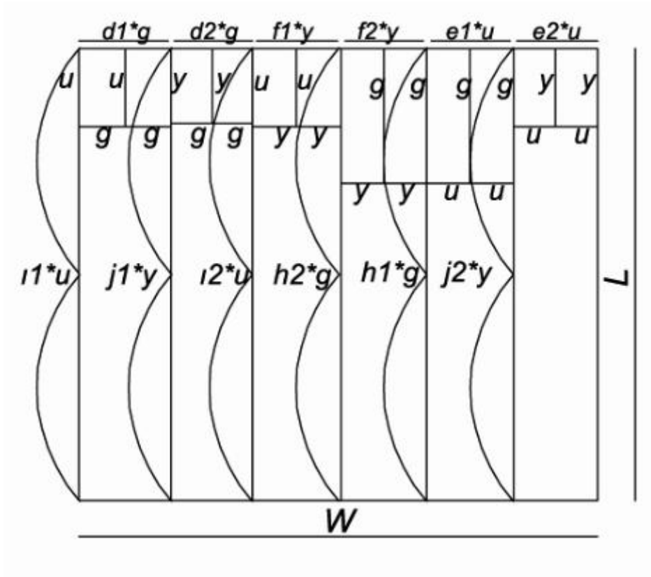
Şekil 6. Aynı türden katlar oluşturarak konteynırın genişliđi boyunca yapılan yükleme
