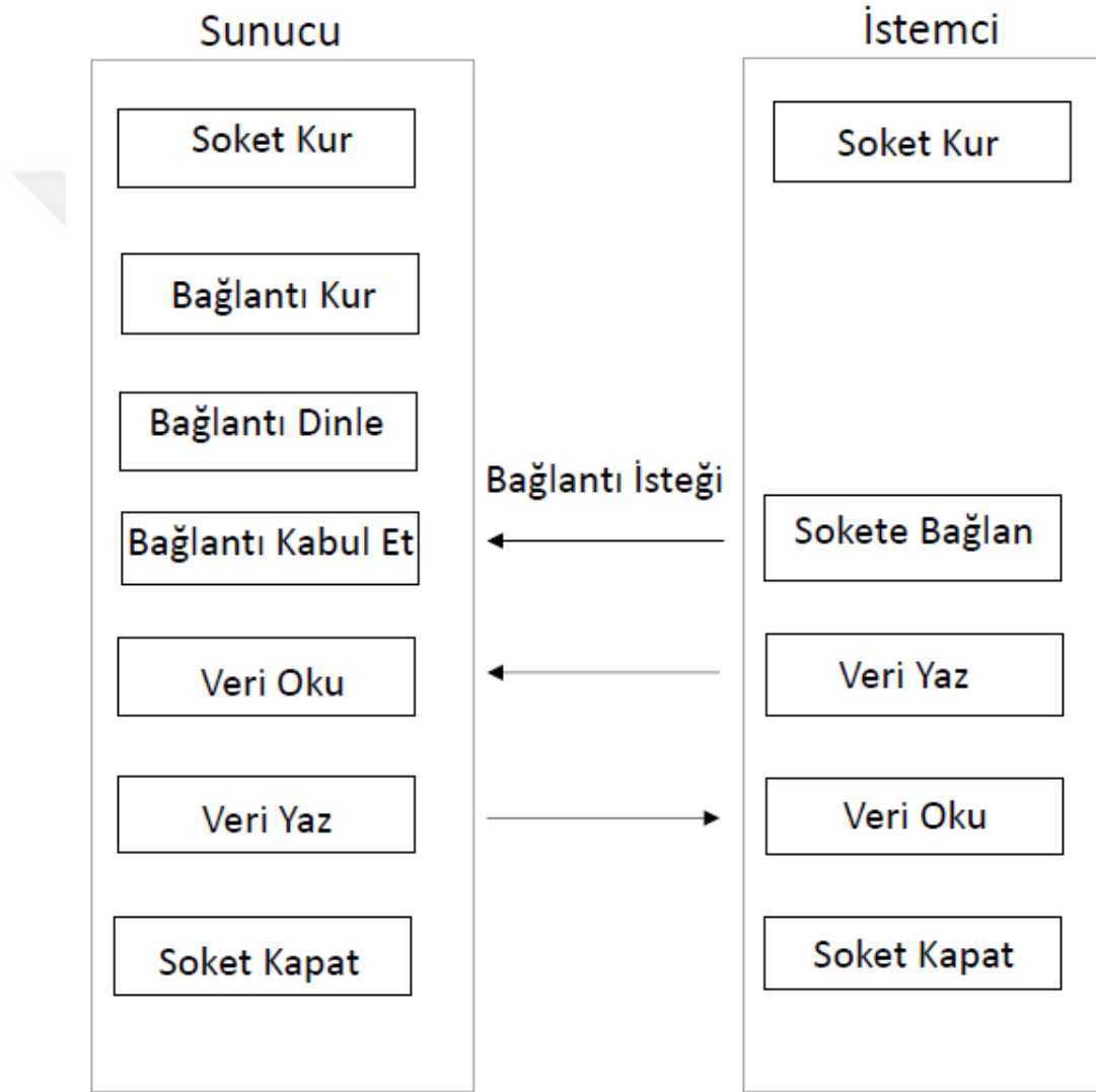
Şekil 3.13. İstemci-sunucu modeli için sıralı diyagram
