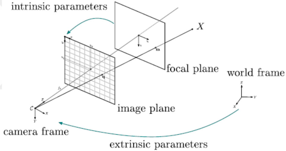
Şekil 2.6. İğne deliği kamerasının genel bir modeli [55]
