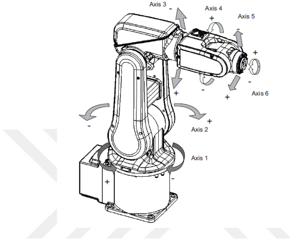
Şekil 2.9. ABB 120 robot mekanik yapı [67]
