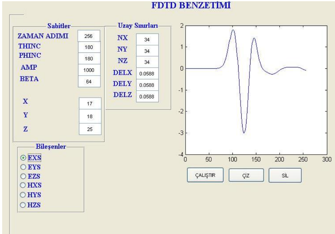
Şekil 3.2 FDTD EXS Sonuç Grafiği
