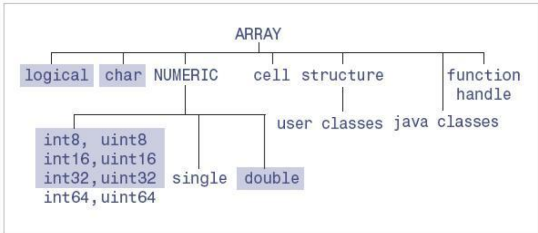
Şekil 3.4 MATLAB TZ’nin Tarafından Desteklenen Veri Tipleri (Gölge Olanlar) [18]
