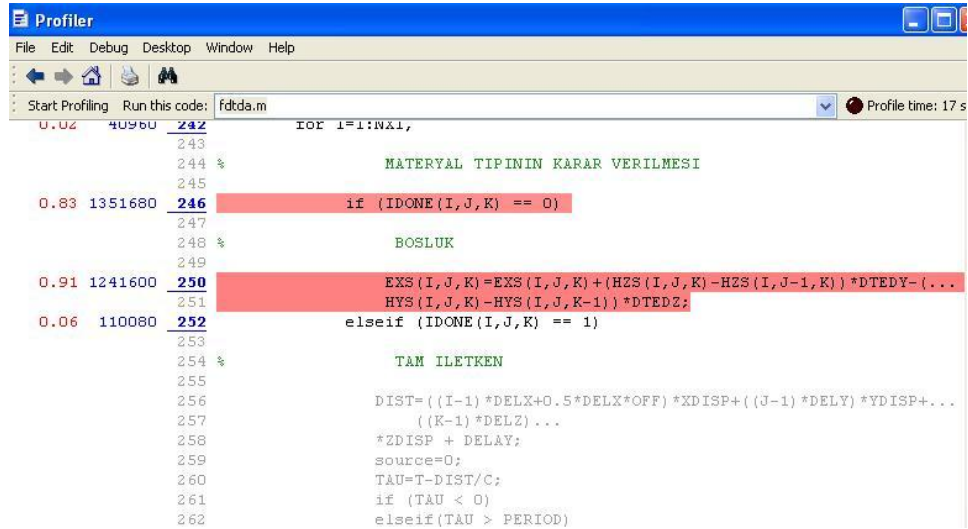
Şekil 3.1 EXS Boşluk Alan Güncellemesi İle İlgili FOR Döngüsü
