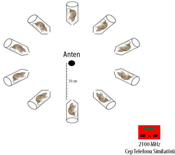
Şekil 3.2. Elektromanyetik radyasyon maruziyeti için kullanılan sistem
