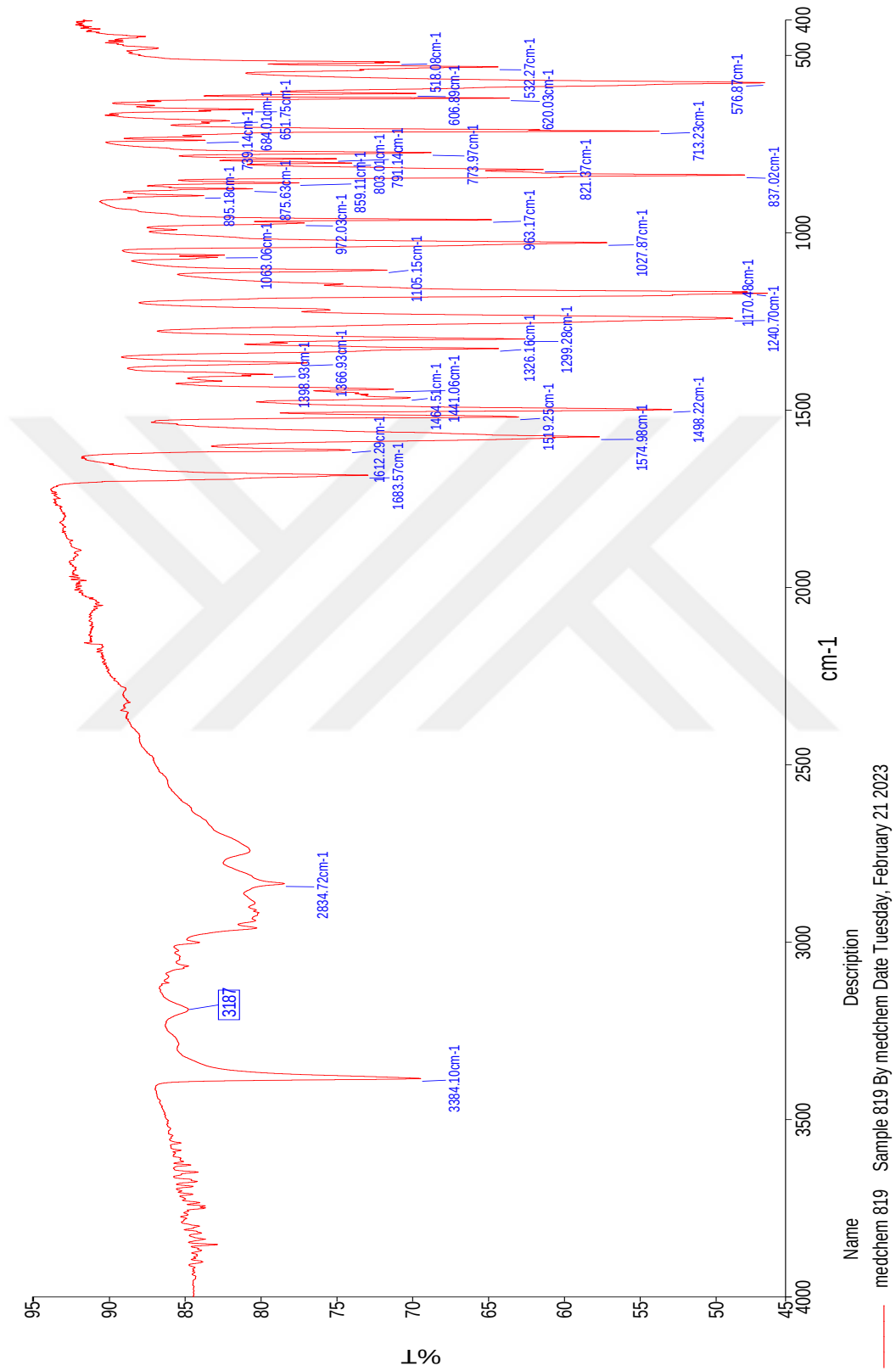
Şekil 4.57. 5j bileşiğinin IR spektrumu
