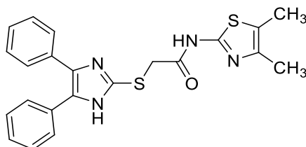
Şekil 4.61. N -(4,5-Dimetiltiyazol-2-il)-2-((4,5-difenil-1 H -imidazol-2-il)tiyo)asetamit (5k) bileşiği
