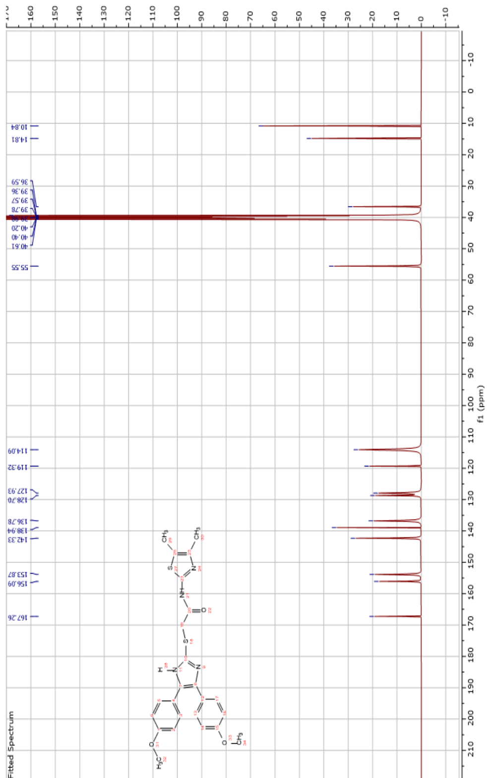
Şekil 4.69. 5I bileşiğinin 13 C-NMR spektrumu
