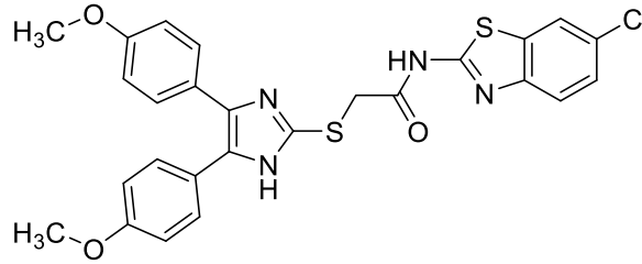
Şekil 4.46. 2-((4,5-Bis(4-metoksifenil)-1H-imidazol-2-il)tiyo)-N-(6-klorobenzo[d]tiyazol-2-il)asetamit (5h) bileşiği
