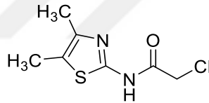
Şekil 4.10. 2-Kloro-N-(4,5-dimetiltiyazol-2-il)asetamit molekülü (4b)
