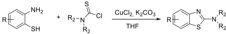
Şekil 1.42. Xu ve diğerlerinin benzotiyazol sentez şeması
