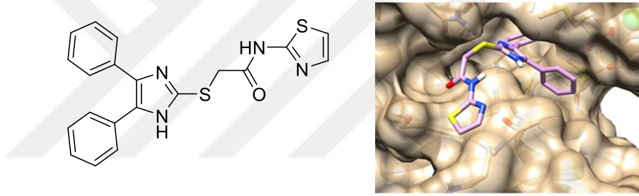
Şekil 1.23. Colderen ve diğerlerinin etkili buldukları Ca^{+2} duyarlaştırıcı bileşik ve bileşiğin modellemesi
