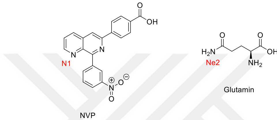
Şekil 1.62. NVP kodlu PDE4 selektif inhibitörü ve PDE4 enziminde bulunan glutamin rezidüsü arasındaki etkileşim yerleri
