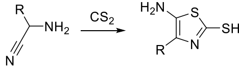
Şekil 1.35. Cook- Heilbron tiyazol sentez şeması
