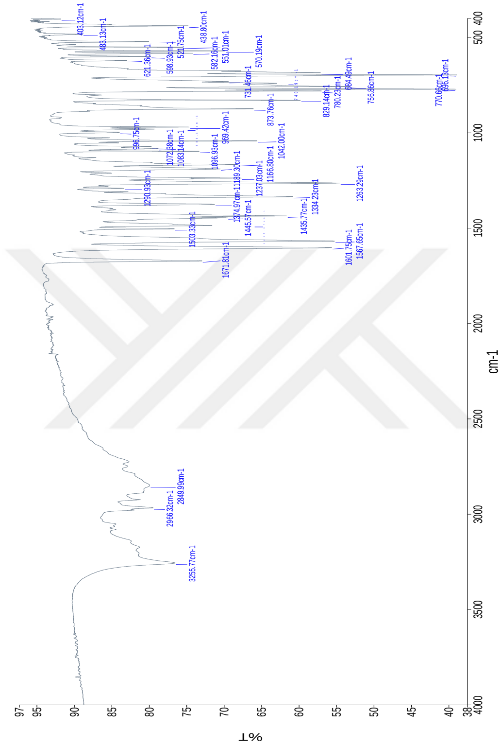
Şekil 4.27. 5d bileşiğinin IR spektrumu
