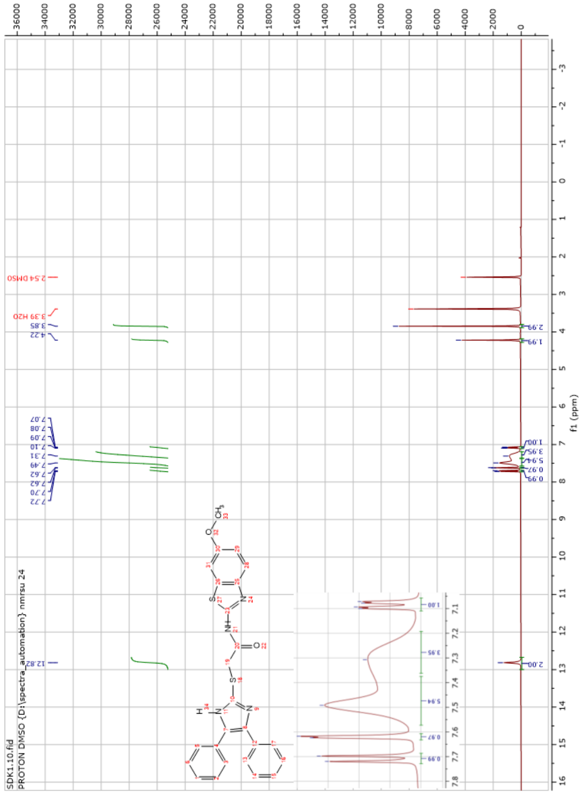
Şekil 4.13. 5a bileşiğinin 1 H-NMR spektrumu
