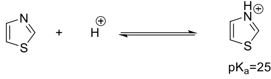
Şekil 1.27. Tiyazol halkasının protonlanması
