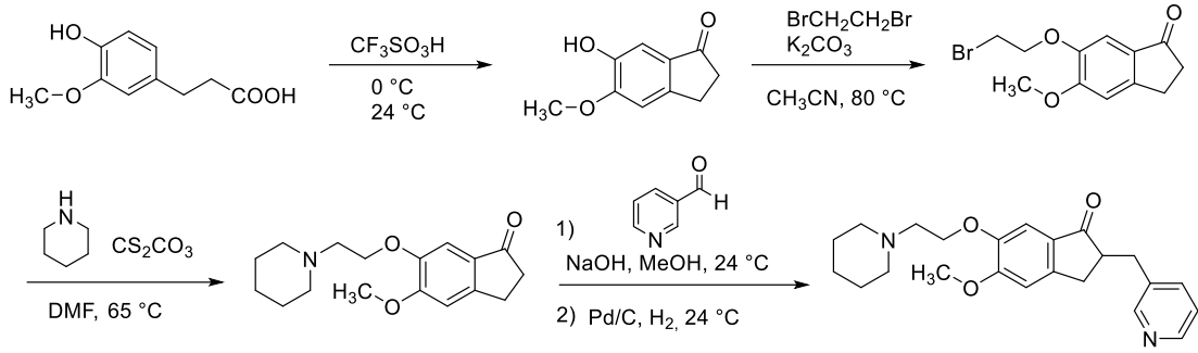
Şekil 1.65. 12C bileşiğinin sentez şeması
