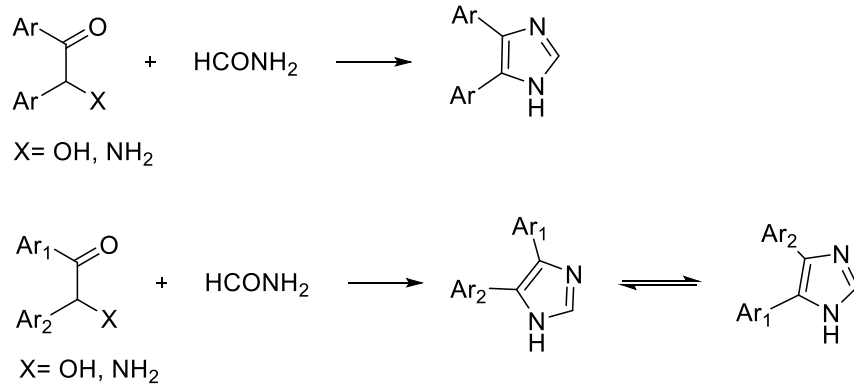
Şekil 1.10. Brederick ve Theilig sentezi
