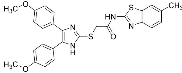
Şekil 4.41. 2-((4,5-Bis(4-metoksifenil)-1H-imidazol-2-il)tiyo)-N-(6-metilbenzo[d]tiyazol-2-il)asetamit (5g) bileşiği
