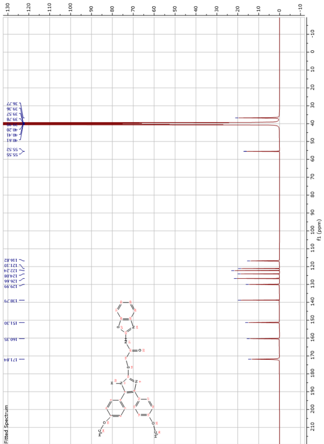
Şekil 4.34. 5e bileşiğinin ^{13}\text{C} -NMR spektrumu
