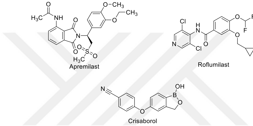
Şekil 1.60. FDA onaylı PDE4 inhibitörlerinin yapıları
