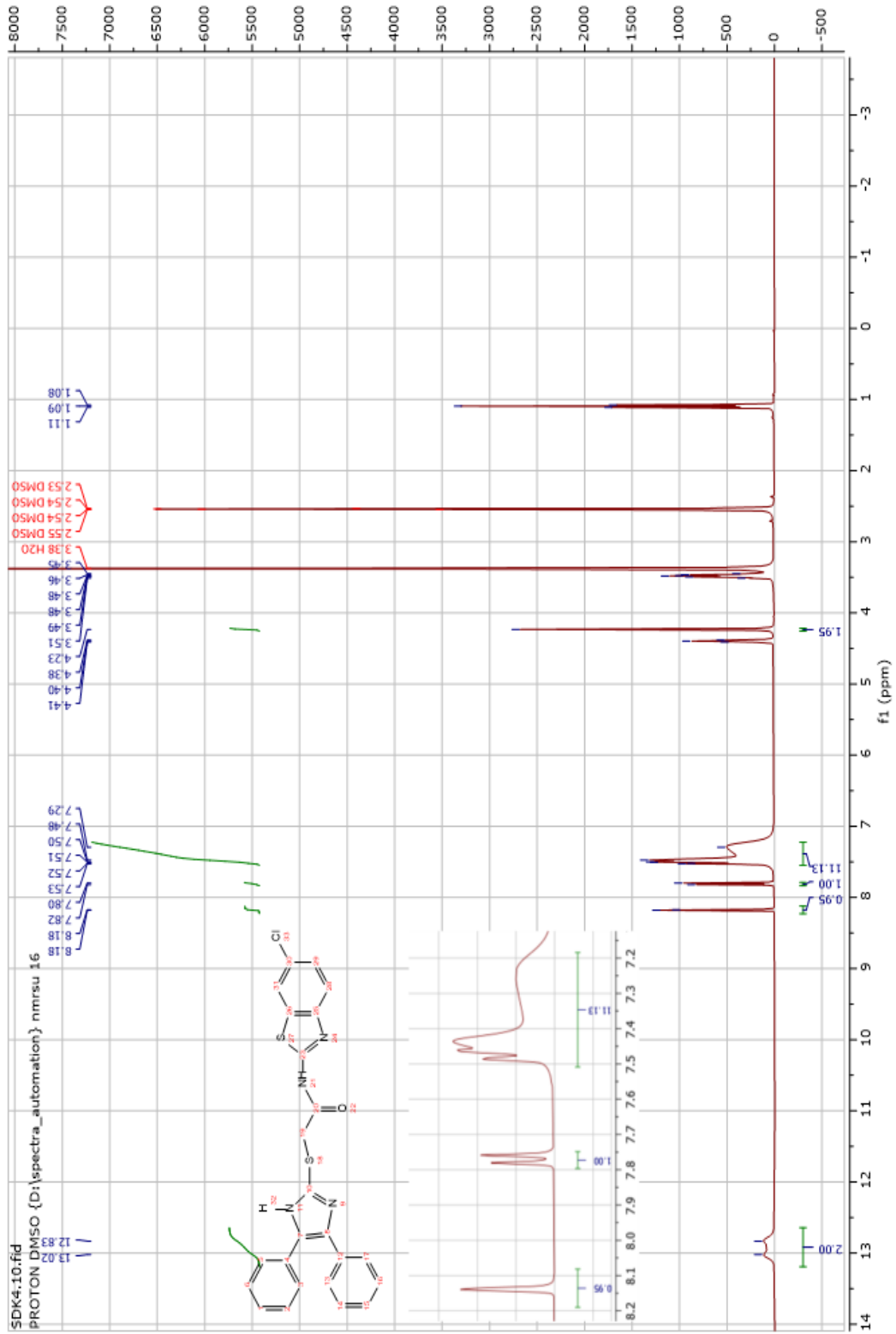
Şekil 4.28. 5d bileşiğinin ^1\text{H} NMR spektrumu
