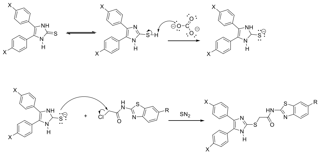
Şekil 4.76. Metot D1'de gerçekleşen sentez mekanizması
