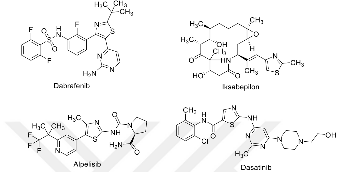
Şekil 1.43. FDA tarafından onaylanmış antikanser etkili tiyazol halkası taşıyan bazı bileşikler
