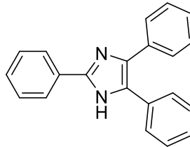
Şekil 1.4. 2,4,5-Trifenilimidazol (Lofin) yapısı
