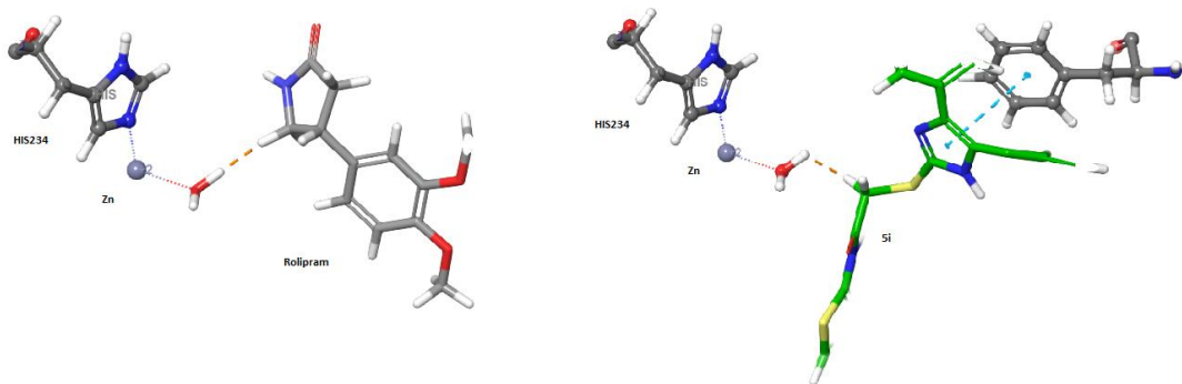
Şekil 4.78. Rolipram (solda) ve 5i (sağda) bileşiklerinin HOH1008 ile etkileşimini gösteren pozlar
