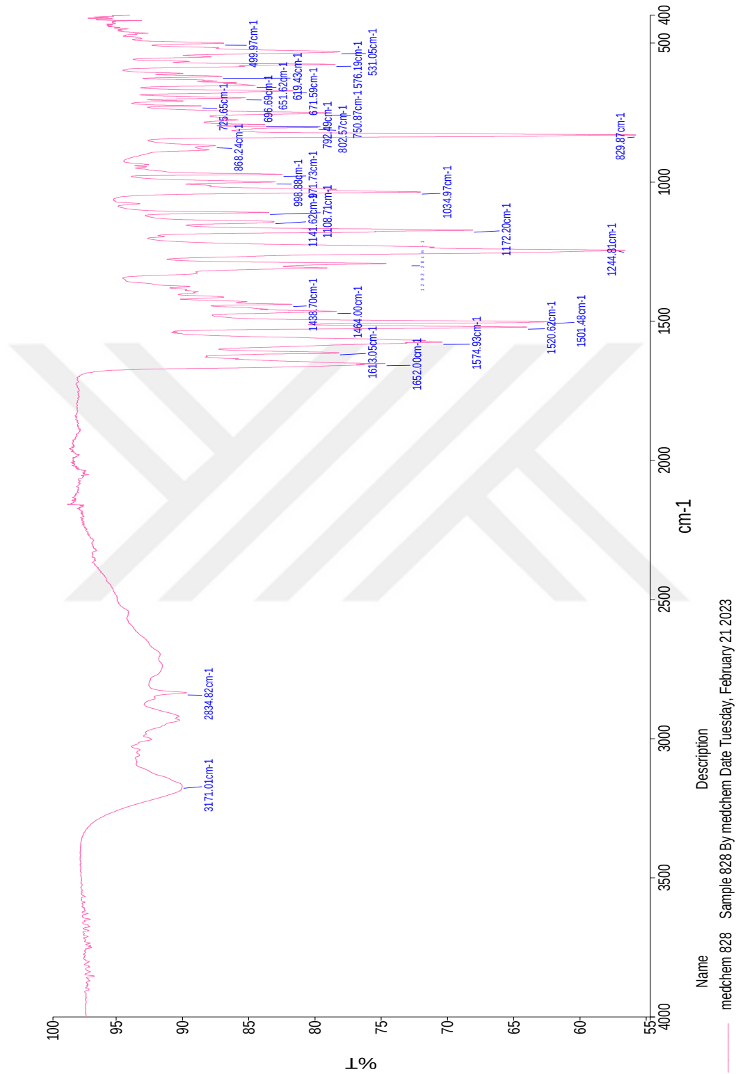
Şekil 4.67. 5I bileşiğinin IR spektrumu
