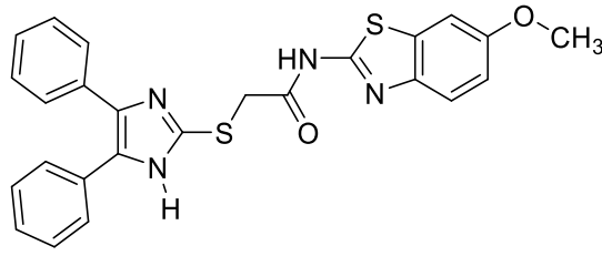
Şekil 4.11. 2-((4,5-Difenil-1H-imidazol-2-il)tiyo)-N-(6-metoksibenzo[d]tiyazol-2-il)asetamid ( 5a ) bileşiği
