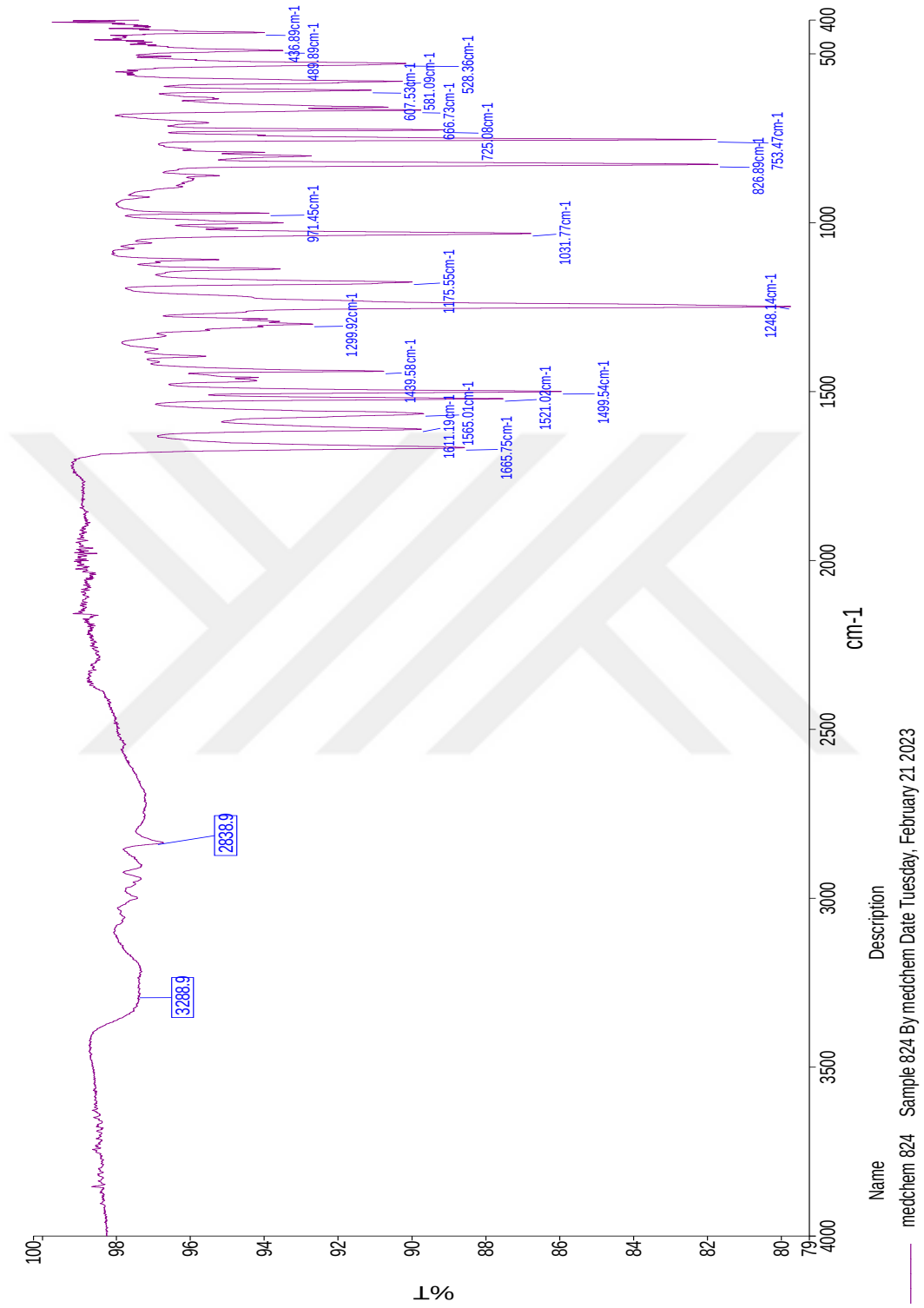
Şekil 4.32. 5e bileşiğinin IR spektrumu
