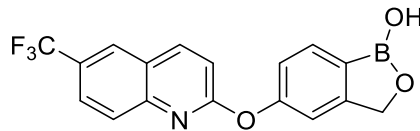
Şekil 1.69. 72 Kodlu bileşiğin yapısı
