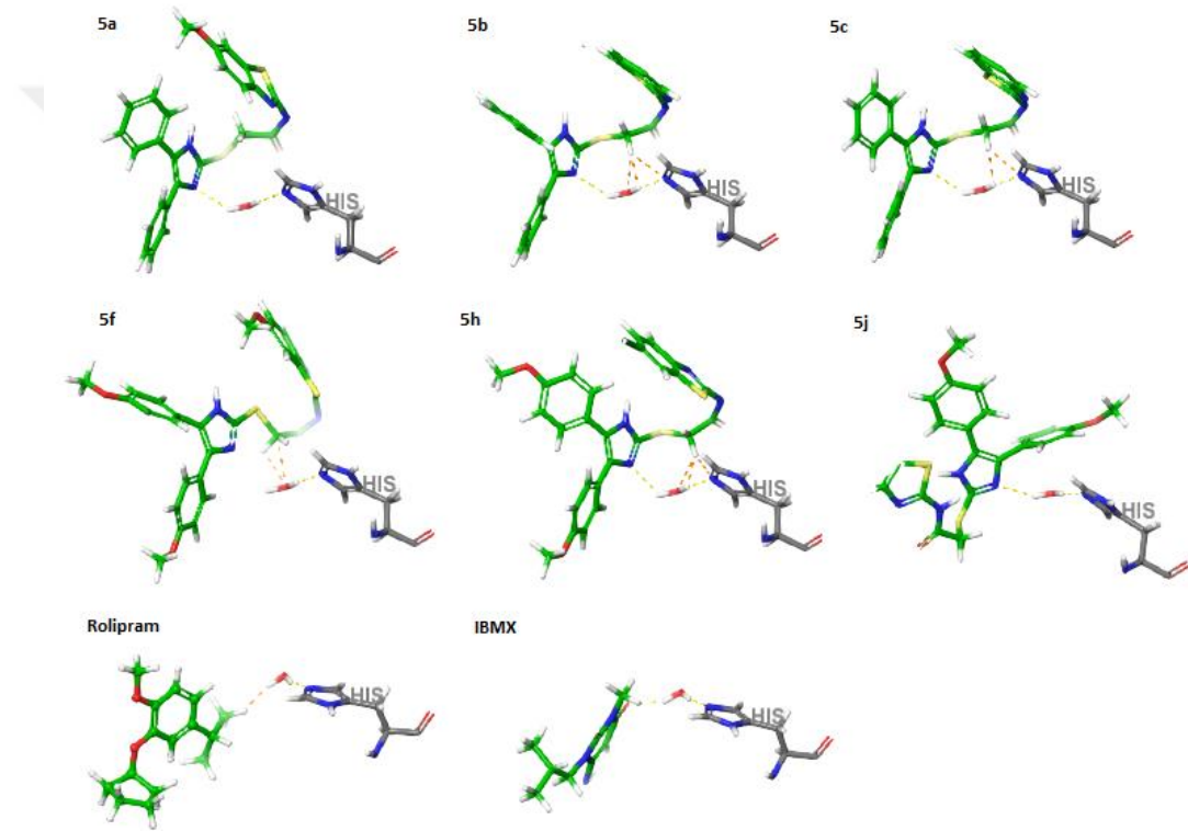
Şekil 4.86. 5a , 5b , 5c , 5f , 5h , 5j , Rolipram ve IBMX bileşiklerinin HOH 1008 ile etkileşimlerine ait pozlar
