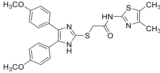
Şekil 4.66. 2-((4,5-Bis(4-metoksifenil)-1H-imidazol-2-il)tiyo)-N-(4,5-dimetiltiyazol-2-il)asetamit (5I) bileşiği
