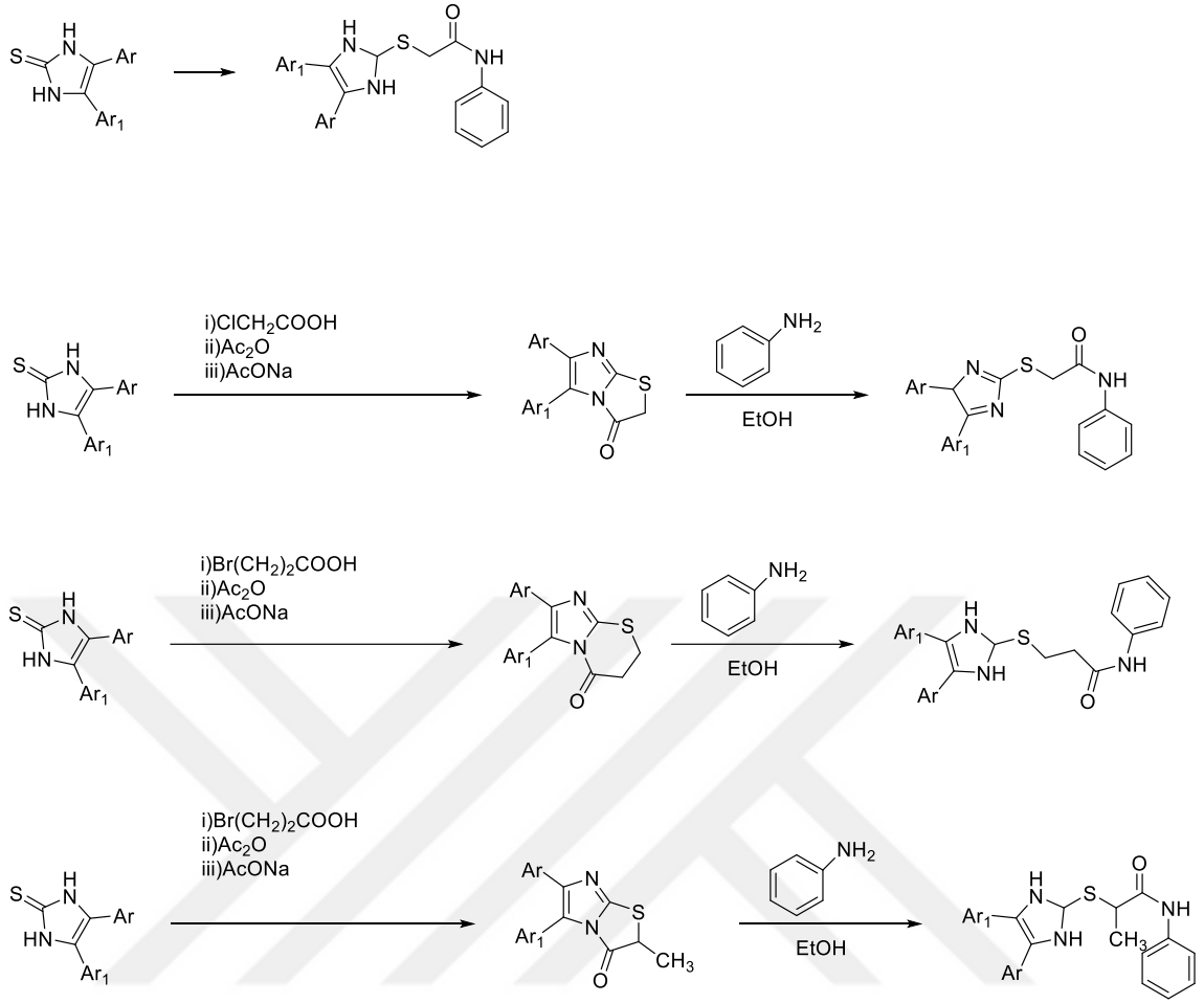
Şekil 1.16. Salama ve diğerleri tarafından oluşturulan 4,5-diaril-1H-imidazolil-2-tiyon türevlerine ait sentez şeması
