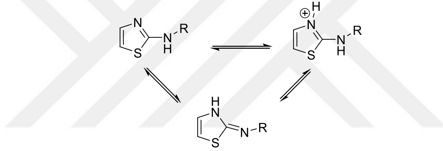
Şekil 1.28. 2-Aminotiyazol halkasının tautomerik yapısı
