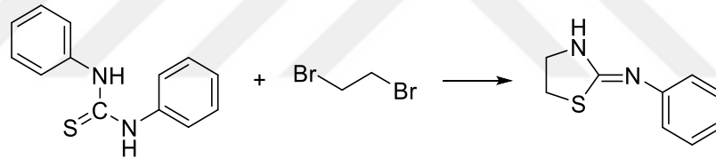
Şekil 1.30. Tiyazol halkasının ilk sentez şeması
