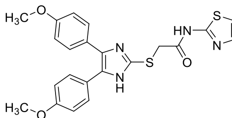
Şekil 4.56. 2-((4,5-Bis(4-metoksifenil)-1H-imidazol-2-il)tiyo)-N-(tiyazol-2-il)asetamit (5j) bileşiği
