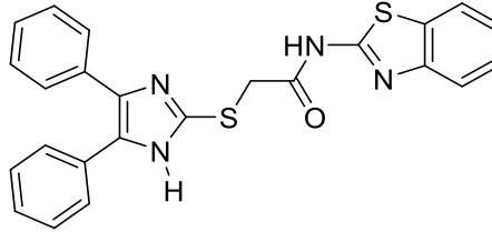
Şekil 4.21. N -(Benzo[d]tiyazol-2-il)-2-((4,5-difenil-1 H -imidazol-2-il)tiyo)asetamit (5c) bileşiği
