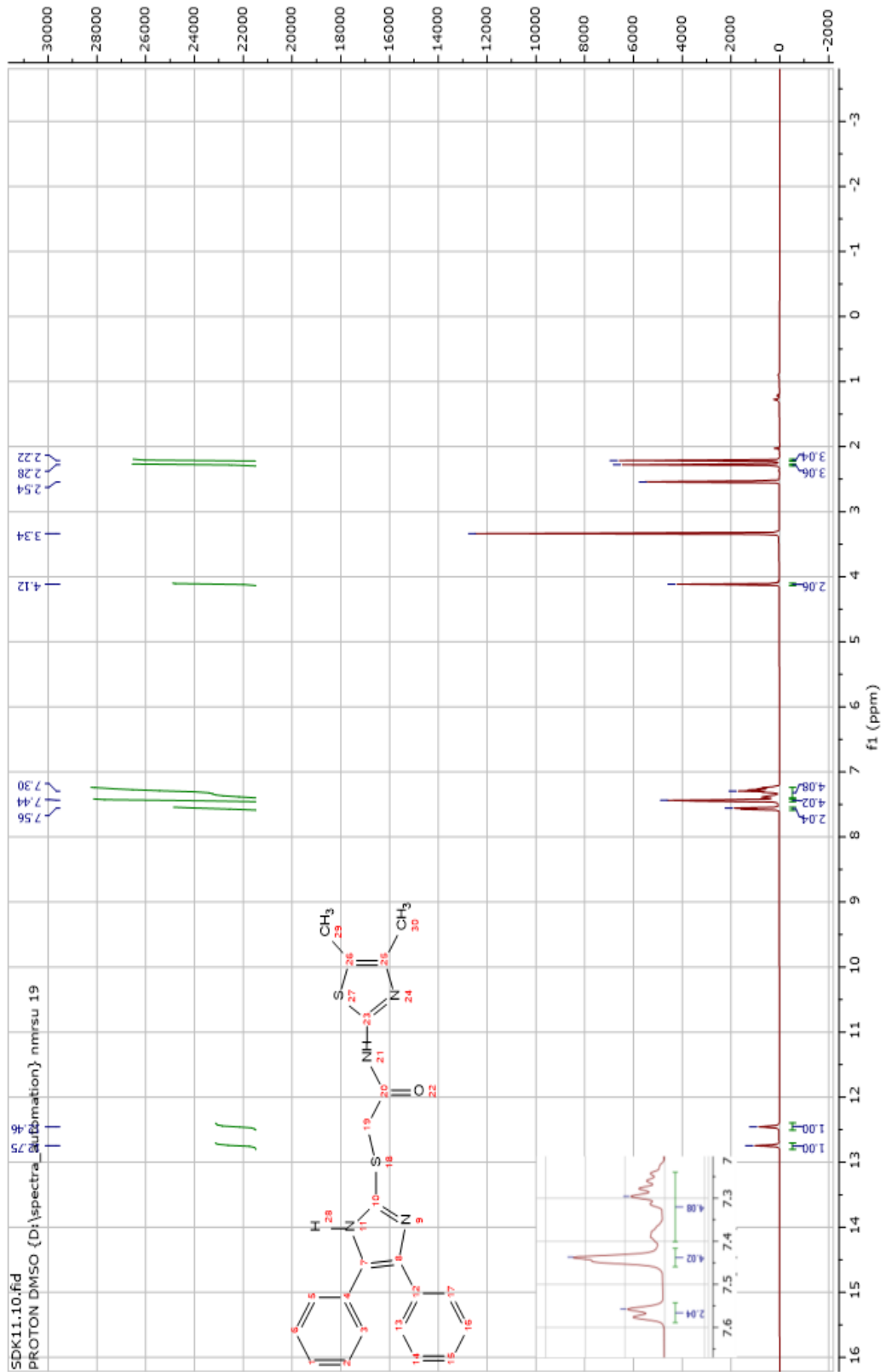
Şekil 4.63. 5k bileşiğinin ^1\text{H} -NMR spektrumu
