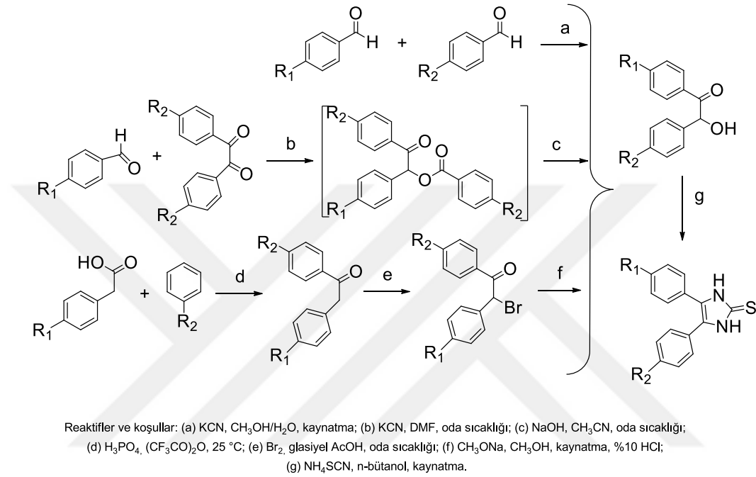
Şekil 1.14. Assadieskandar ve diğerleri tarafından oluşturulan 4,5-diaril-1H-imidazolil-2-tiyon türevlerine ait sentez şeması
