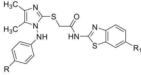
Şekil 1.53. Yurttaş ve diğerlerinin sentezlediği C6 ve HepG2 hücre hatlarında etkili bileşik
