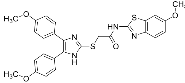
Şekil 4.36. 2-((4,5-Bis(4-metoksifenil)-1H-imidazol-2-il)tiyo)-N-(6-metoksibenzo[d]tiyazol-2-il)asetamit (5f) bileşiği
