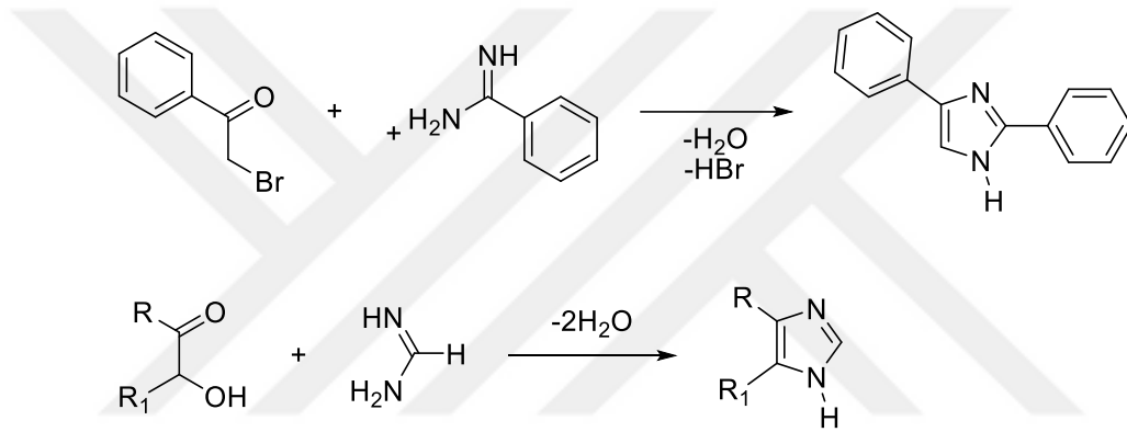
Şekil 1.13. Alfa haloketondan hareketle 4,5-diarilimidazol türevlerinin sentez şeması
