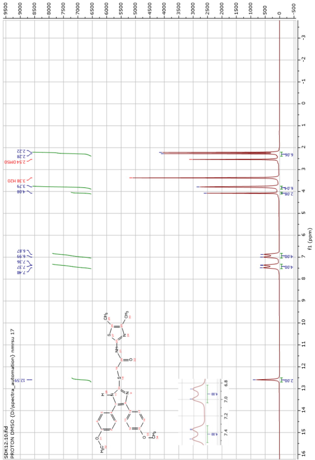
Şekil 4.68. 51 bileşiğinin ^1\text{H} -NMR spektrumu
