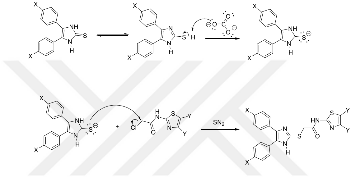
Şekil 4.77. Metot D2’de gerçekleşen sentez mekanizması
