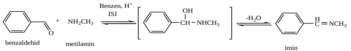
Şekil 1.3. Aromatik yapılu imin reaksiyon denklemleri
