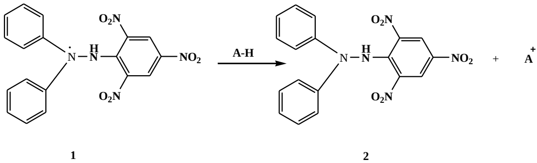
Şekil 1.10. DPPH serbest radikal ile antioksidan reaksiyonu. 1: DPPH serbest radikali, 2: DPPH indirgenmiş formu
