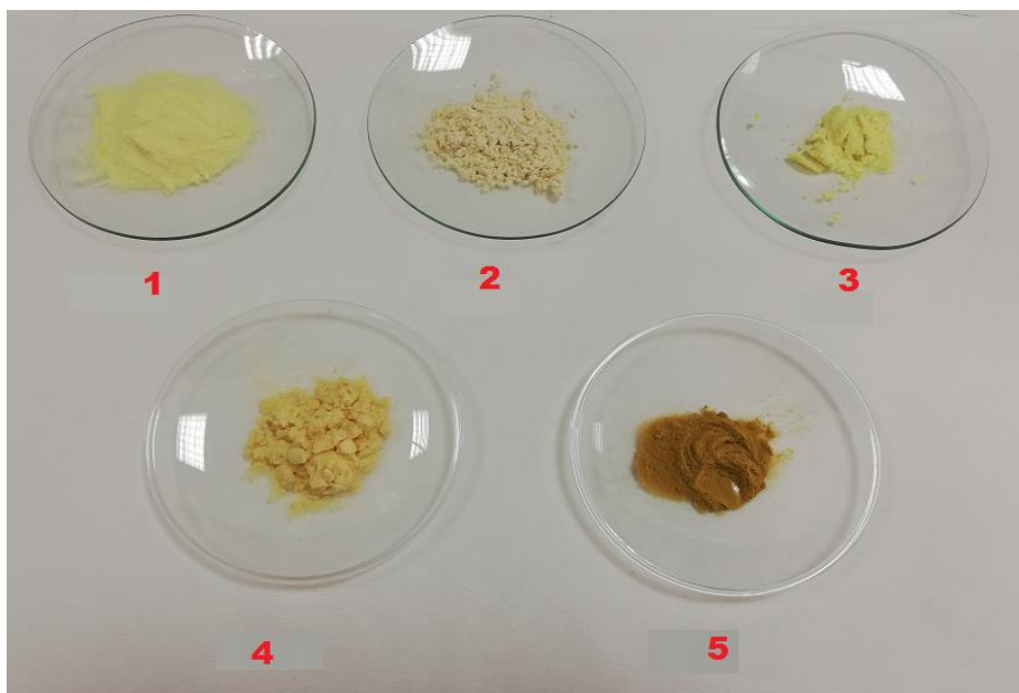
Şekil 4.2. Bileşik 1-5 katı toz görünimleri
