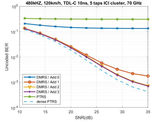
(d) Uncoded BER for 120 km/h.
