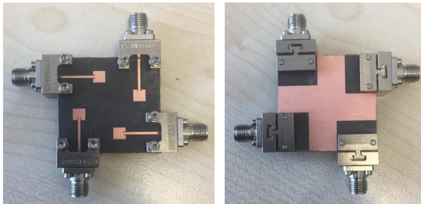
Resim 8.1. Üretilen MIMO antenin (a) ön, (b) arka yüzleri
