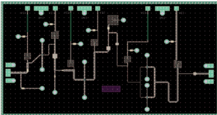
Şekil 6.5. Üç aşamalı MMIC LNA'nın şematiği
