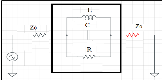
Şekil 4.13. Halter DGS'nin RLC eşdeğer devresi
