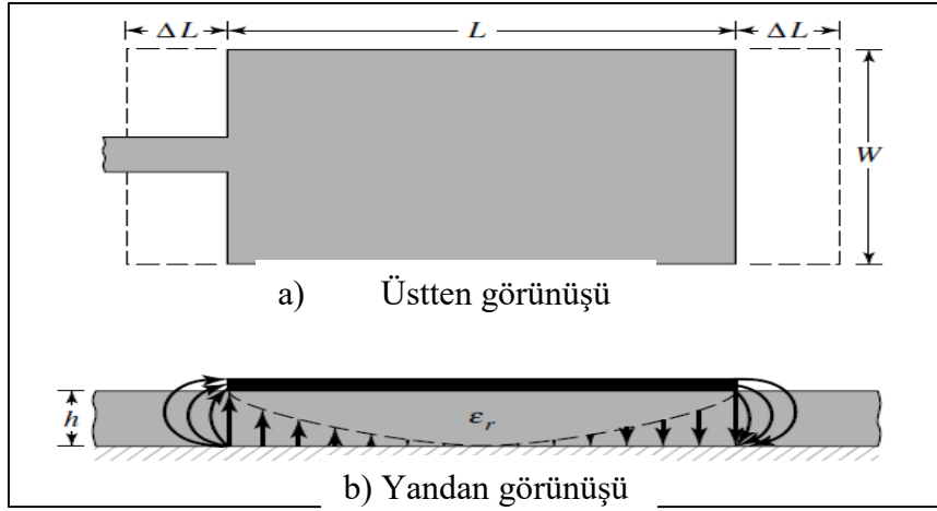
Şekil 2.9. Dikdörtgen mikroşerit yapının etkin ve fiziksel uzunlukları
