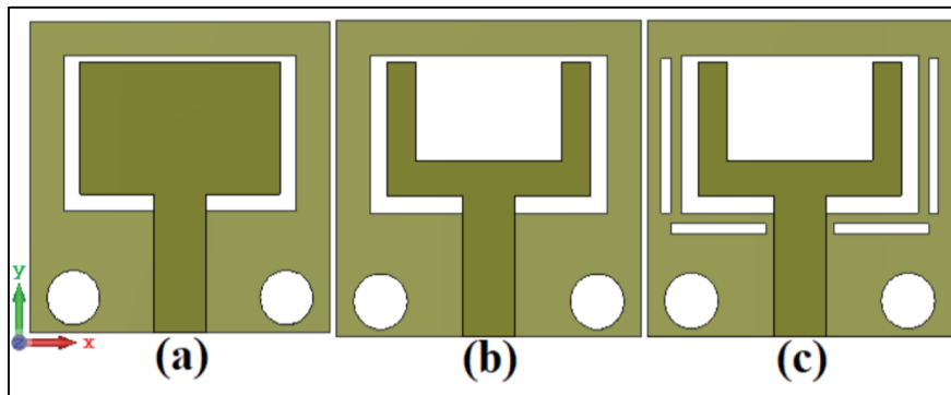
Şekil 5.1. (a) Dikdörtgen yama anten, (b) U-şekilli yama anten (c) Önerilen anten
