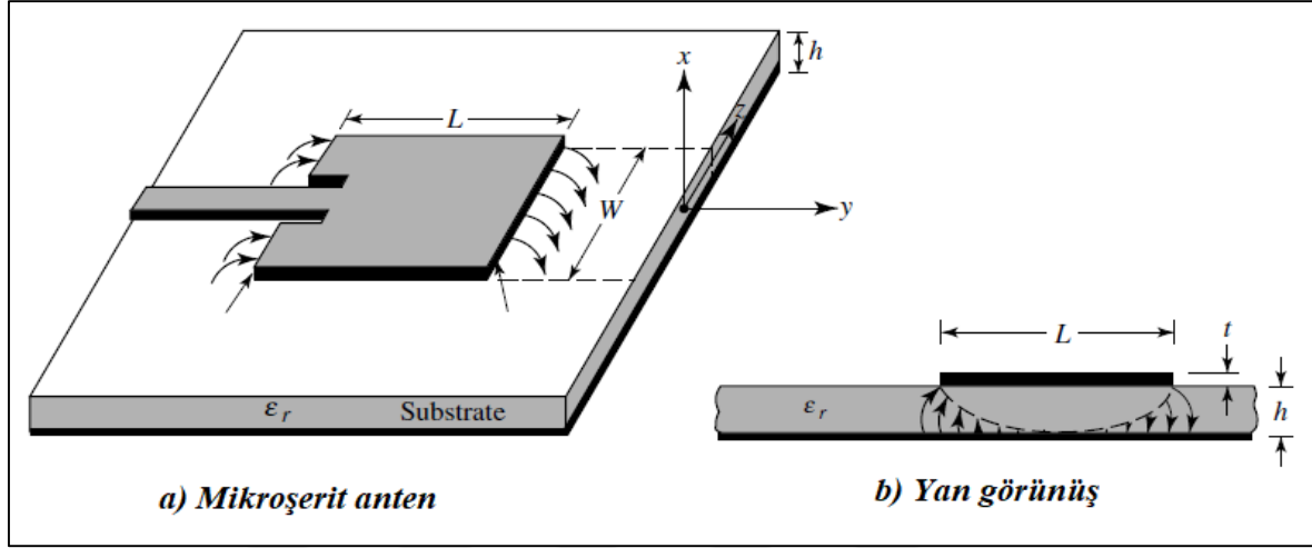
Şekil 2.4. Mikroşerit anten üstten ve yandan görünüşü
