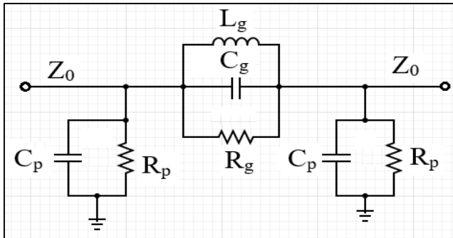
Şekil 4.14. Halter DGS'nin pi tipi eşdeğer devresi
