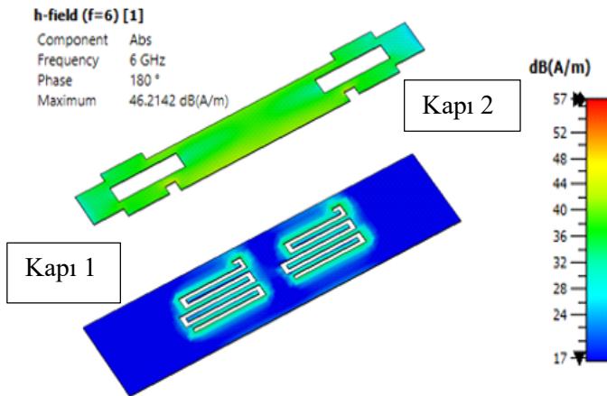
Şekil 7.13. İletim bandı (6 GHz) EM alan dağılımı
