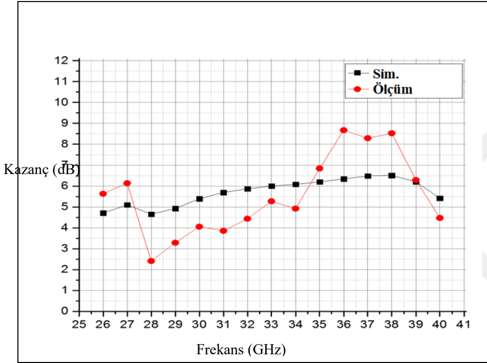
Şekil 5.8. Anten kazanç değerlerinin ölçüm ve simülasyon sonuçlarının karşılaştırılması
