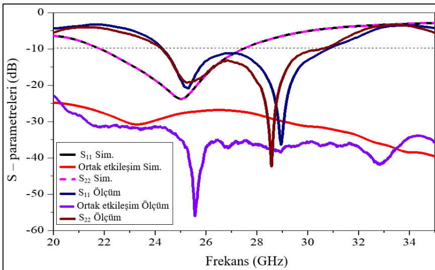
Şekil 8.6. Ölçüm ve simülasyon sonuçları
