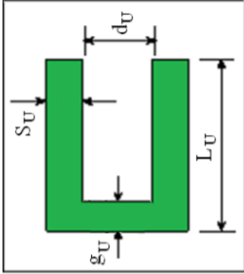
Şekil 4.7. U şekilli DGS
