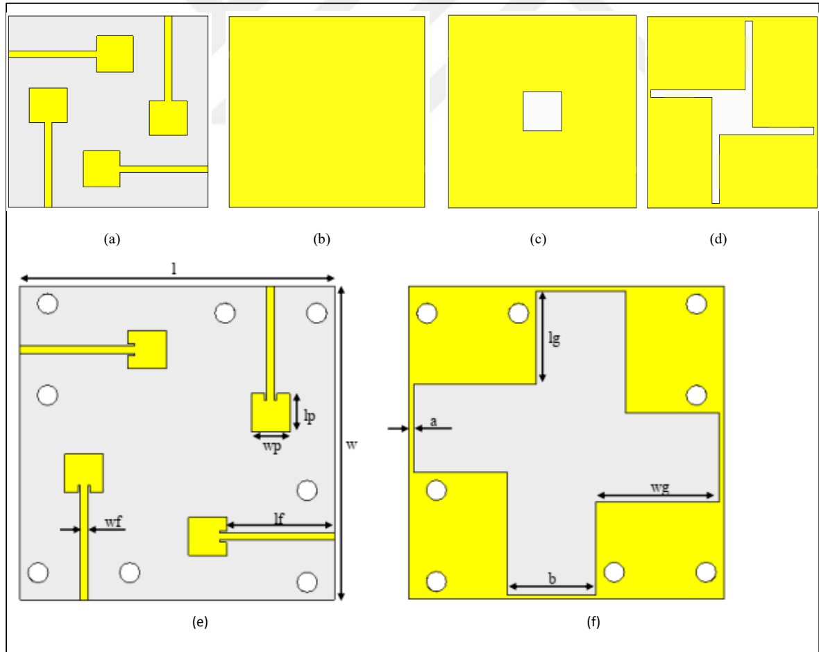
Şekil 8.1. Önerilen tasarım yapısı (a) üst görünüm, (b) step-1 alt görünüm, (c) step-2 alt görünüm (d) step-3 alt görünüm (e) final tasarımın üst görünümü (f) final tasarımın alt görünümü
