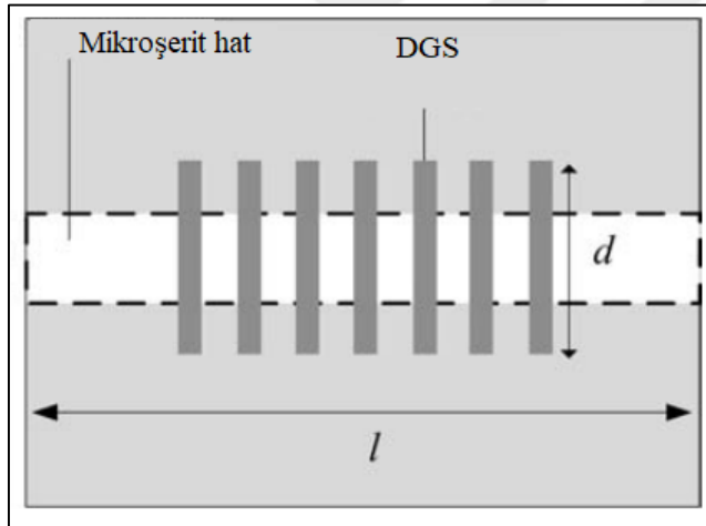
Şekil 4.10. Yedi hücreli periyodik DGS yapısı
