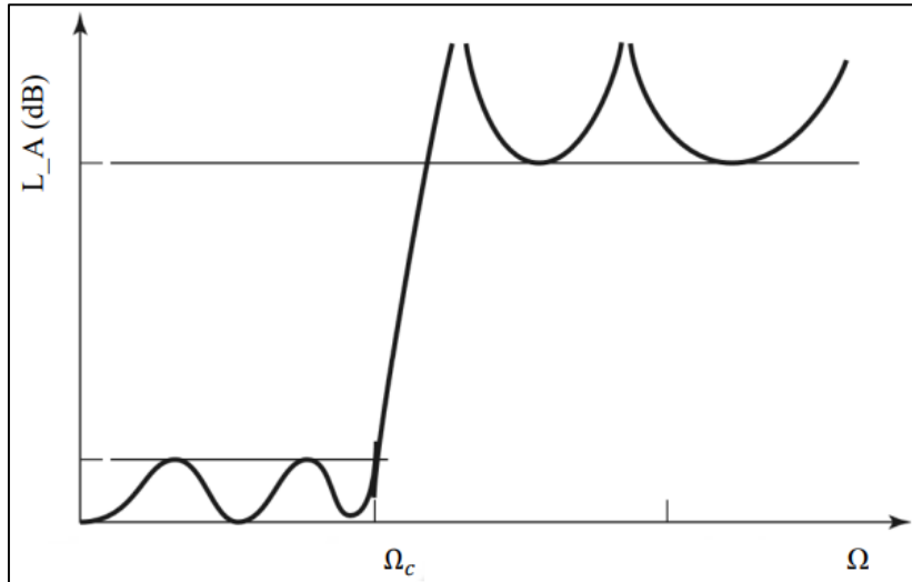
Şekil 3.11. Eliptik filtre frekans tepkisi [85]
