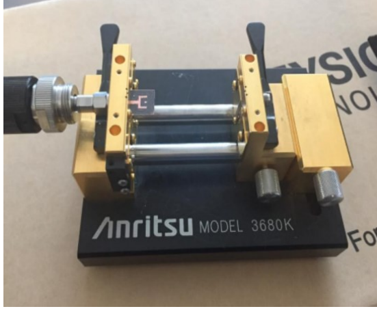
Resim 5.2. Test fixture cihazı
