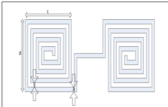
Şekil 4.5. Spiral şekilli DGS
