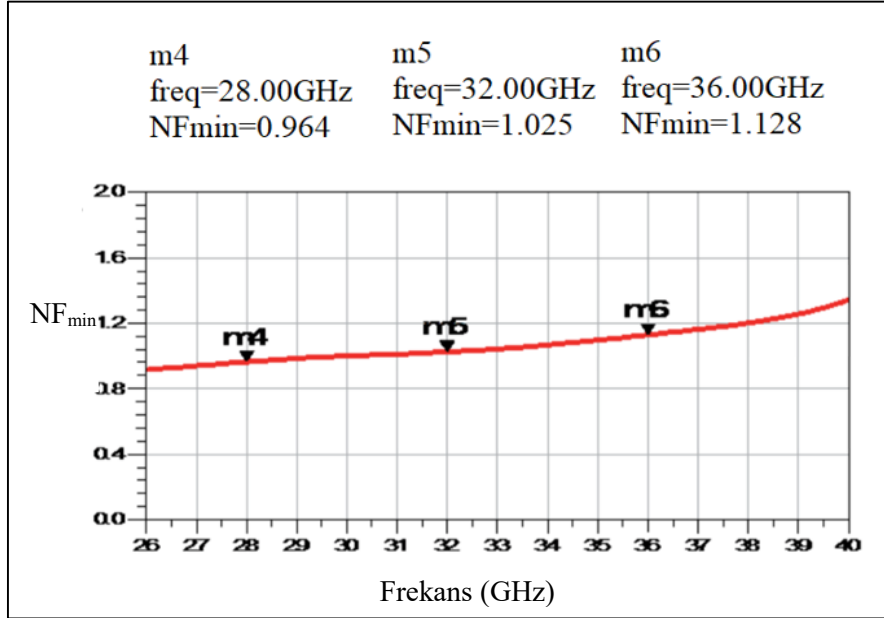
Şekil 6.7. MMIC LNA'nın gürültü katsayısı simülasyon sonuçları
