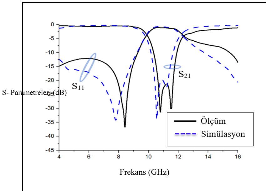
Şekil 7.6. Simülasyon ve ölçüm sonuçlarının karşılaştırılması (Aşama-2)
