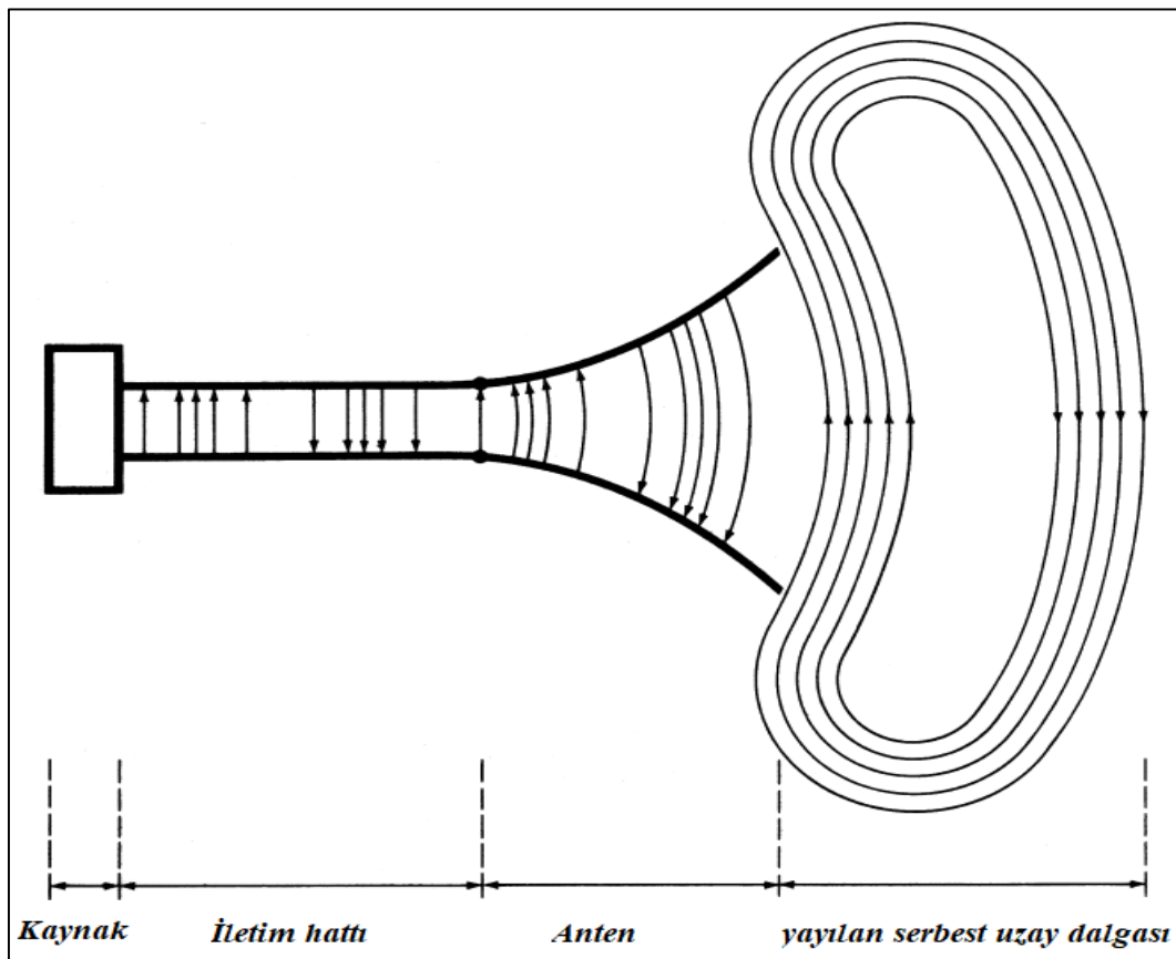
Şekil 2 1. Basit anten yapısı
