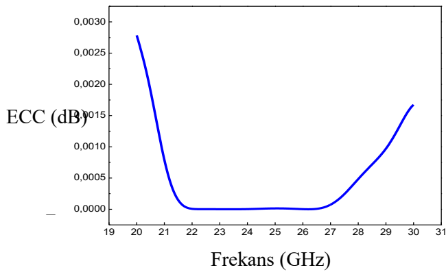
Şekil 8.11. MIMO anten ECC grafiği
