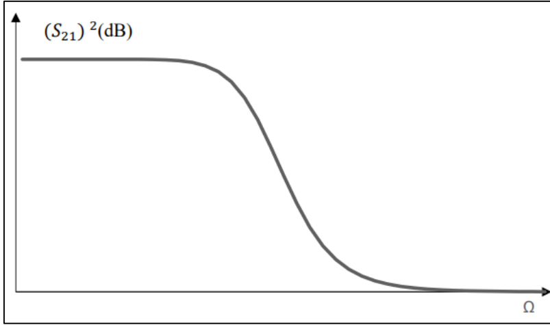
Şekil 3.7. Butterworth filtre frekans tepkisi
