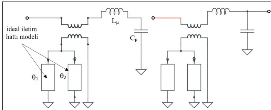
Şekil 4.11. Periyodik DGS'nin eşdeğer devresi
