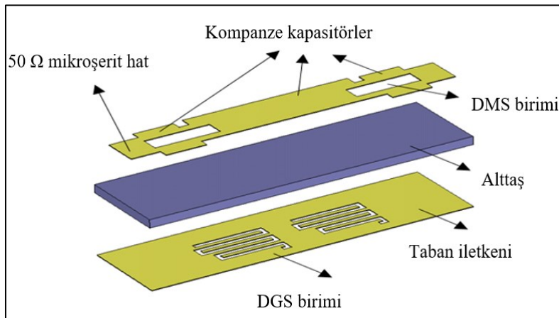
Şekil 7.8. Önerilen BSF tasarımın 3D görseli
