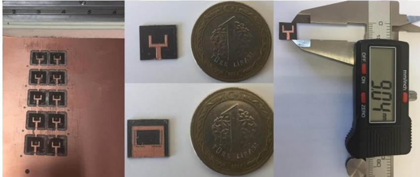
Resim 5.1. Üretilen tekli antenin görselleri
