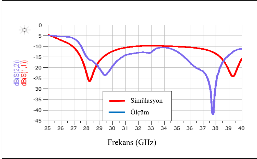
Şekil 5.6. Ölçüm ve simülasyon sonuçlarının karşılaştırılması
