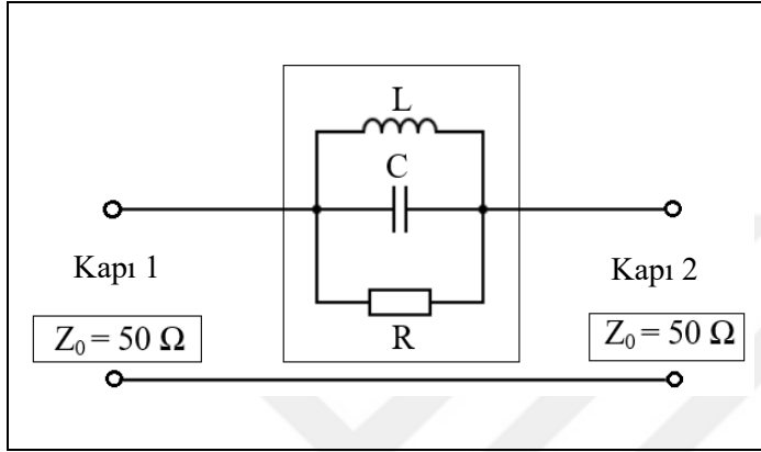
Şekil 7.2. Önerilen taban iletkeni kusurlu yapının eşdeğer devre modeli
