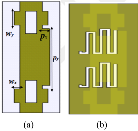
Şekil 7.7. Bant söndüren filtre tasarımının görselleri (a) besleme yüzeyi (b) topraklama yüzeyi
