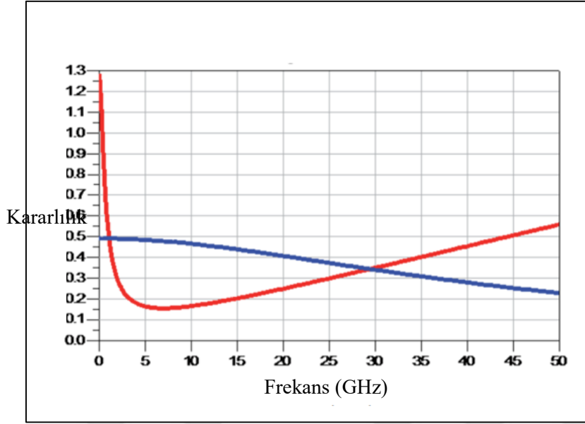
Şekil 6.2. 2 x 30 \mu\text{m} m-HEMT'nin kararlılık simülasyonu sonuçları
