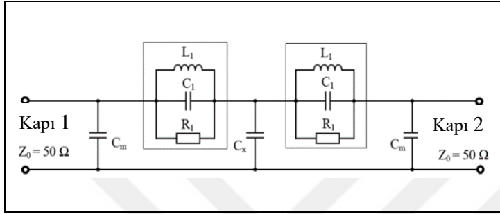
Şekil 7.10. Önerilen BSF eşdeğer devre modeli
