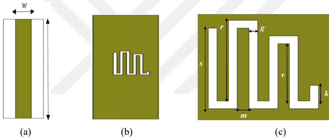
Şekil 7.1. Mikroşerit filtrenin geometrik yapısı (Aşama-1): (a) besleme yüzeyi (b) topraklama yüzeyi (c) önerilen taban iletkeni kusurlu yapı
