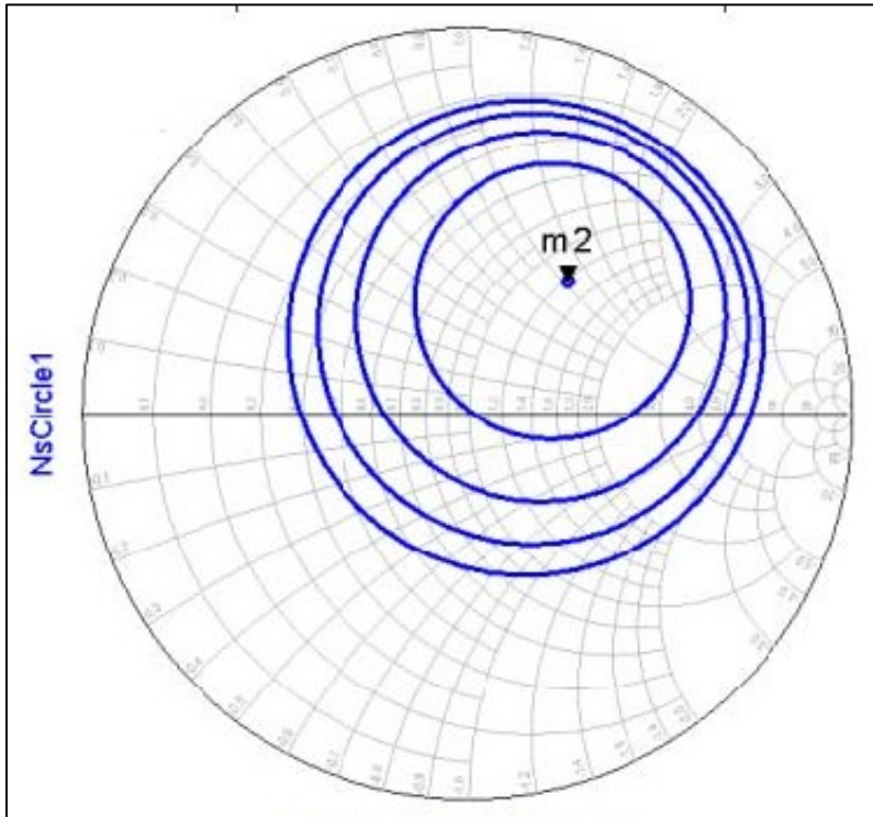
Şekil 6.1. 2 \times 30 \mu\text{m} m-HEMT gürültü çemberleri
