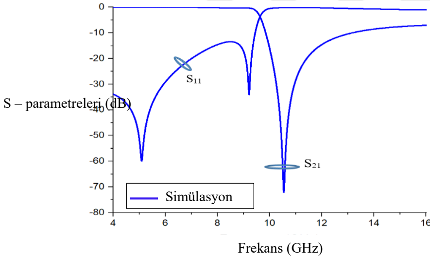
Şekil 7.11. Eşdeğer devre modelin S-parametre grafiği
