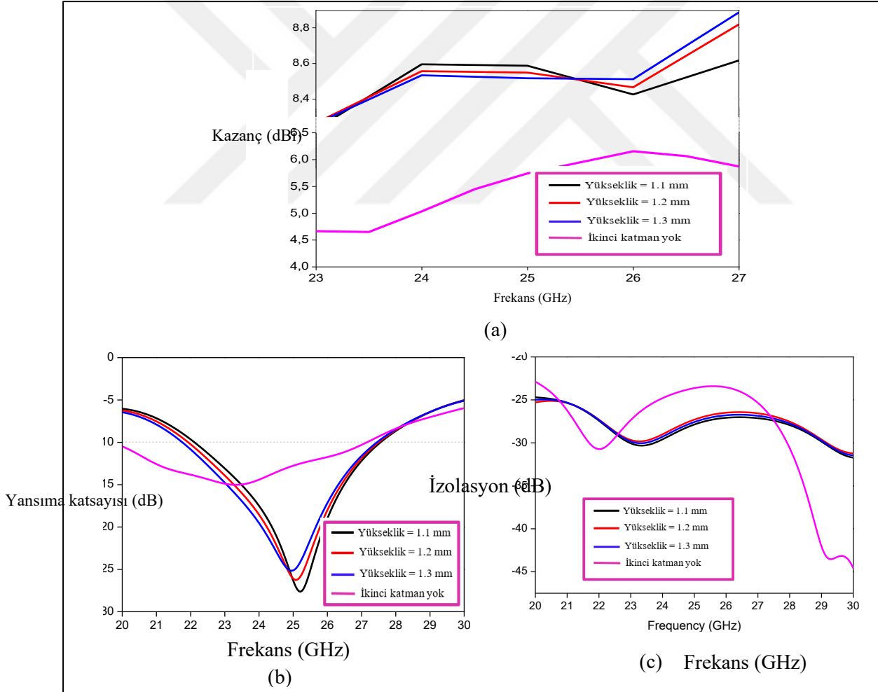
Şekil 8.5. Yüksekliğin (a) anten kazancına etkisi (b) bant genişliğine etkisi (c) izolasyona etkisi
