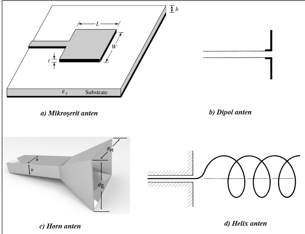
Şekil 2.3. Yaygın olarak kullanılan çeşitli anten yapıları
