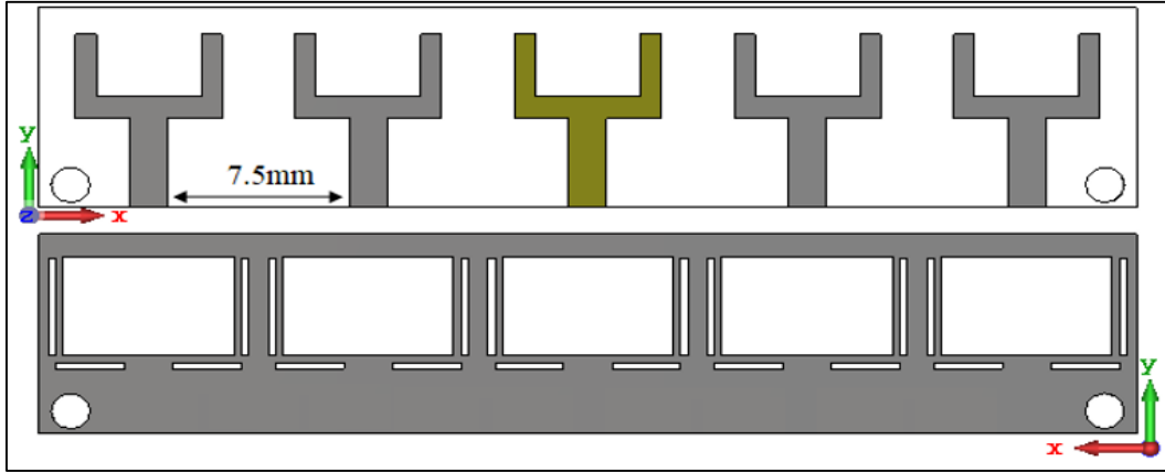
Şekil 5.9. Dizi anten tasarımı
