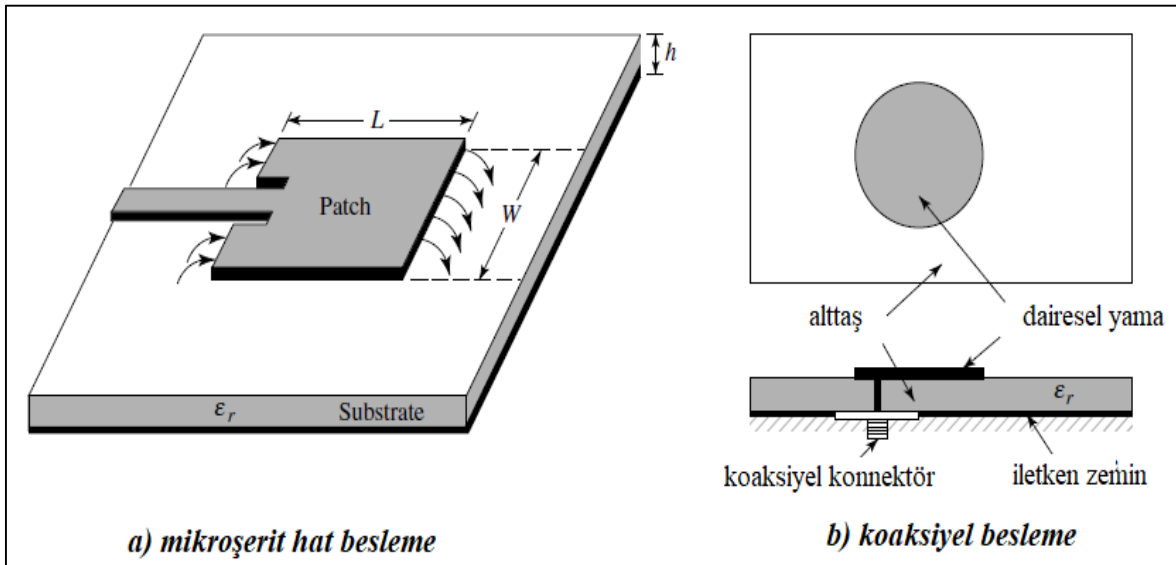
Şekil 2.6. Mikroşerit anten besleme türleri
