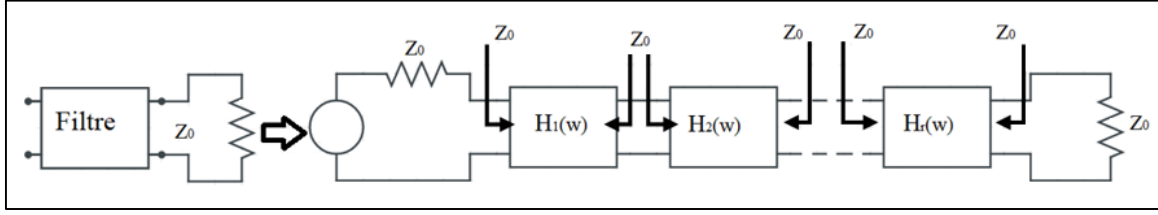
Şekil 3.4. GP ile filtre tasarımı [2]
