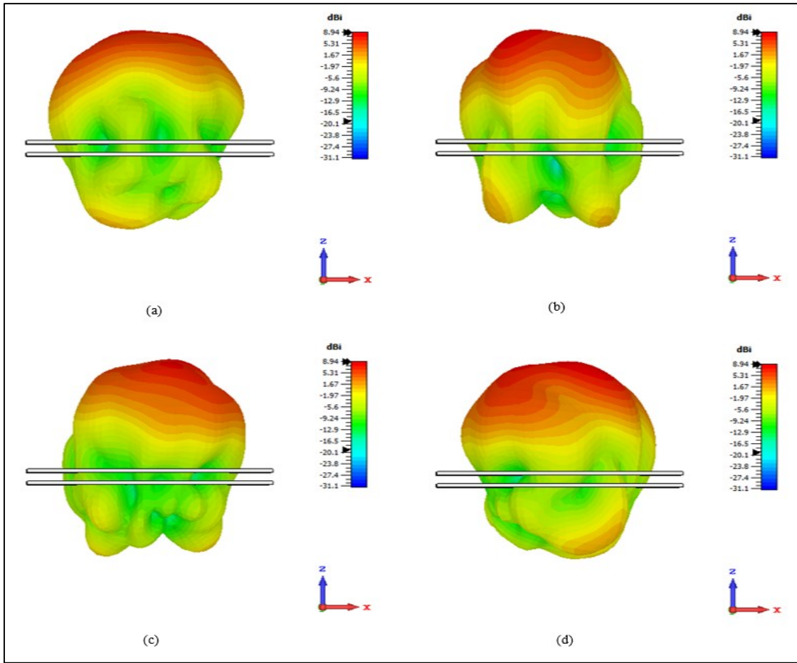
Şekil 8.7. 3D ışıma örüntüsünün simülasyon sonuçları
