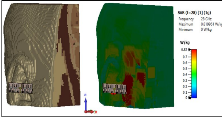
Şekil 5.13. Dizi anten SAR analizi
