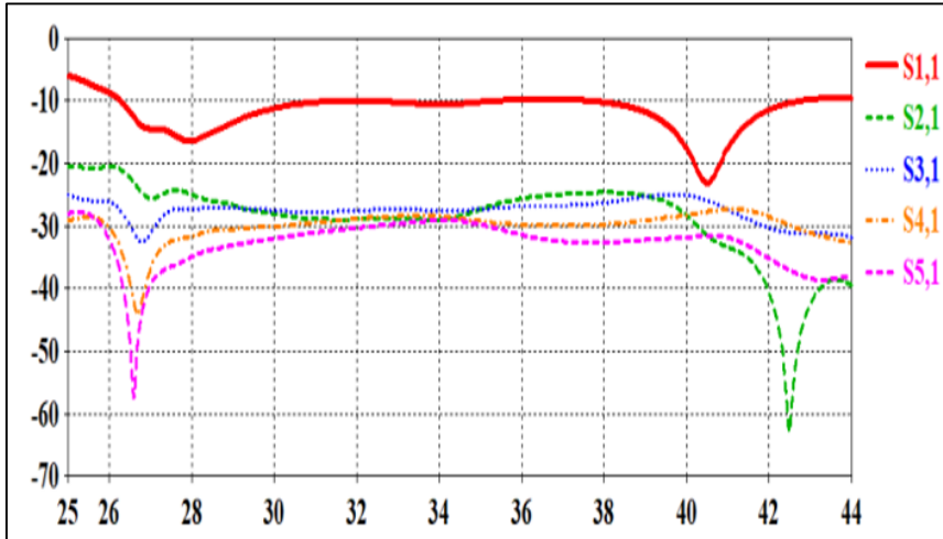
Şekil 5.10. Dizi anten ortak etkileşim tepkisi
