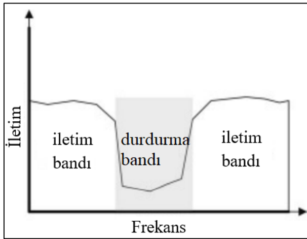
Şekil 4.1. EBG yapısının iletim karakteristiği
