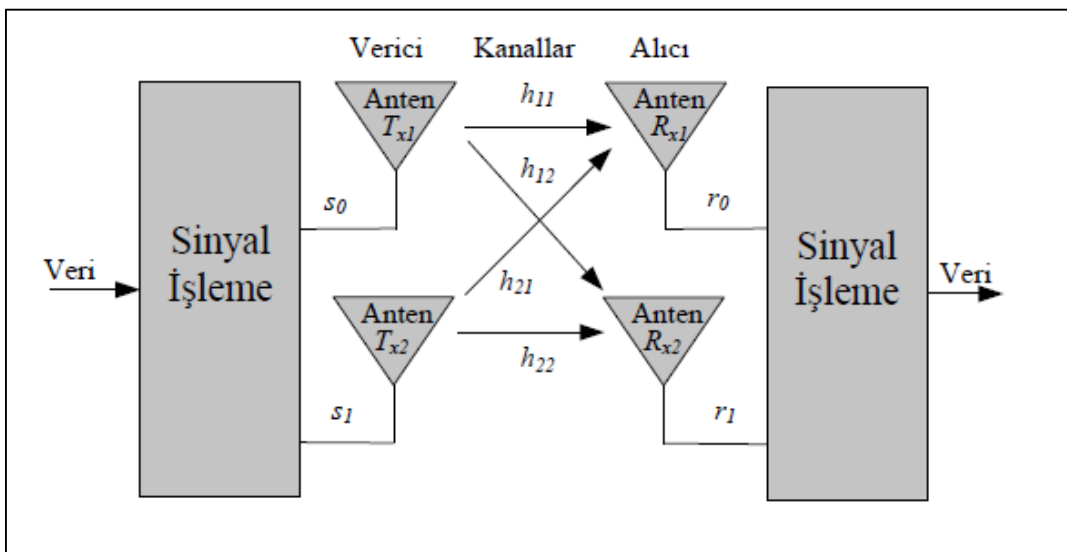
Şekil 2.12. 2 x 2 MIMO anten mimarisi
