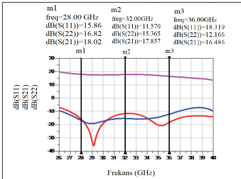
Şekil 6.6. MMIC LNA'nın S-Parametre simülasyon sonuçları
