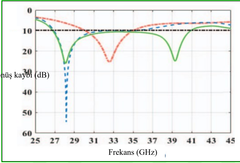
Şekil 5.2. Üç farklı anten modelinin geri dönüş kayıpları
