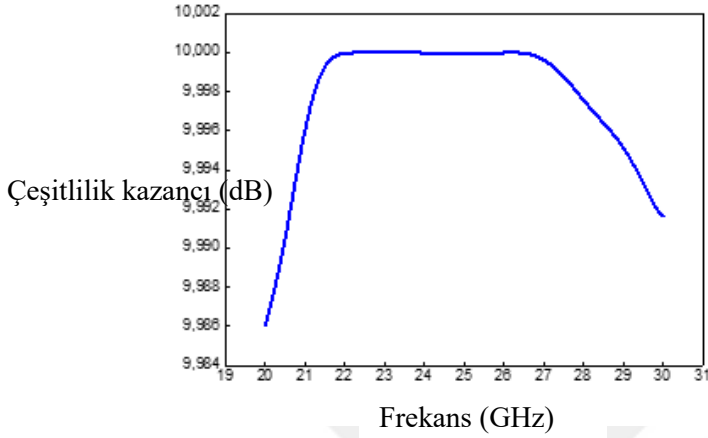
Şekil 8.12. MIMO anten DG grafiği
