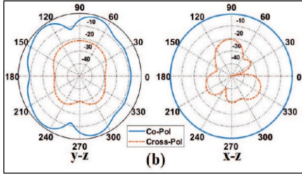
Şekil 5.5. Önerilen antenin 39 GHz'deki ışıma örüntüsü
