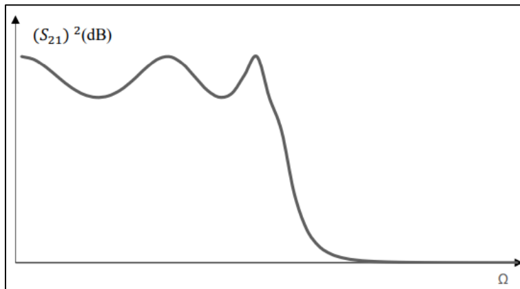
Şekil 3.9. Chebyshev filtre frekans tepkisi [85]
