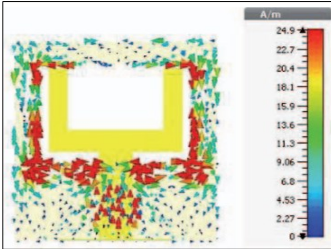
Şekil 5.4. Önerilen antenin 39 GHz'de yüzey akım dağılımları
