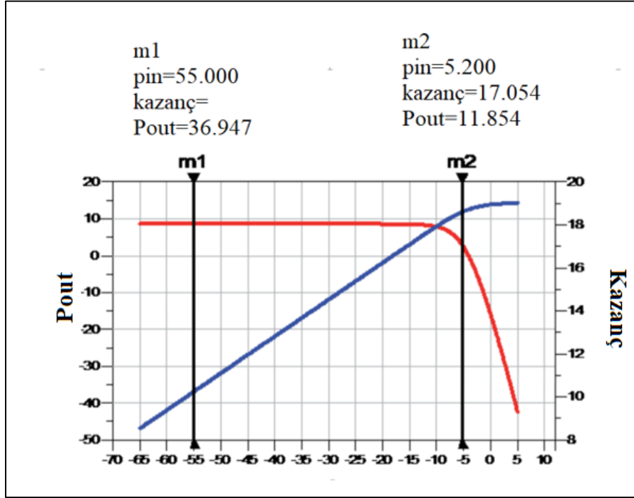
Şekil 6.9. MMIC LNA'nın doğrusallık simülasyonu sonucu
