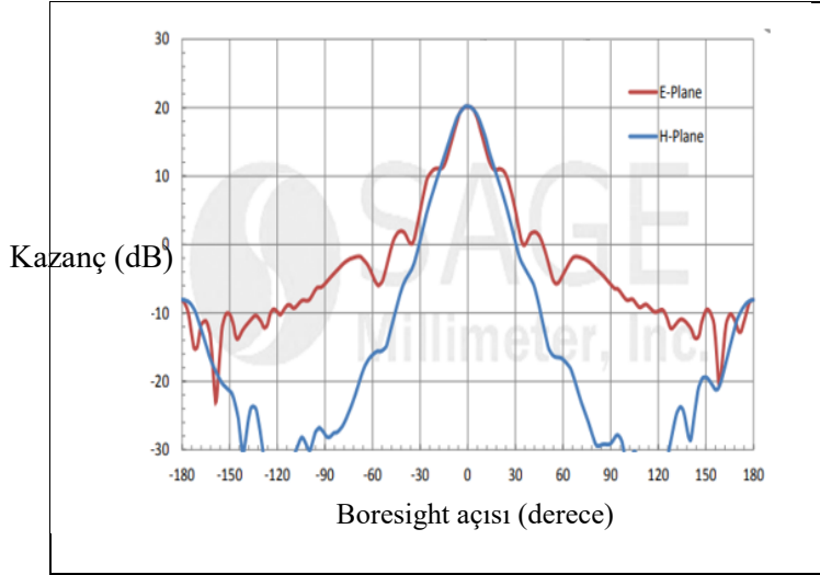
Şekil 5.7. Horn anten kazanç grafiği
