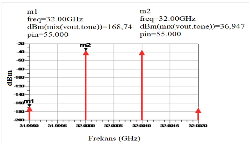
Şekil 6.8. MMIC LNA'nın doğrusallık simülasyonu sonucu
