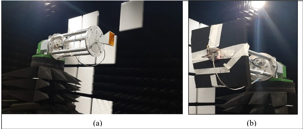
Şekil 8.9. Yankısız oda (a) referans horn anten (b) önerilen anten
