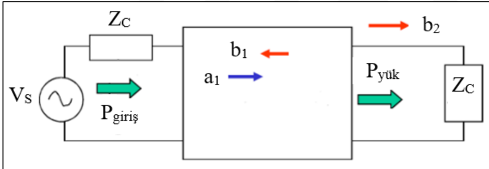
Şekil 3.6. AGK güç aktarım şeması
