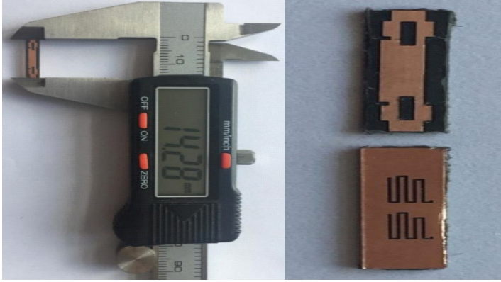
Resim 7.1. Üretilen bant söndüren filtre görselleri
