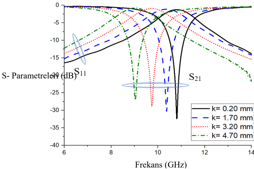
Şekil 7.4. Farklı "k" değerleri için elde edilen S-parametreleri
