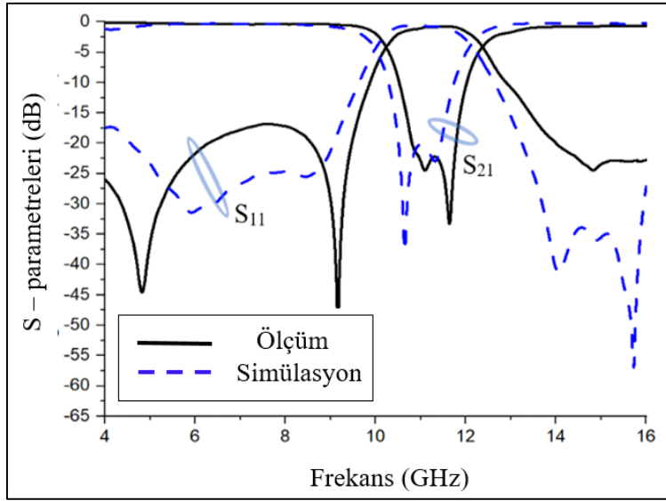
Şekil 7.14. Önerilen BSF'nin ölçüm ve simülasyon sonuçlarının karşılaştırılması
