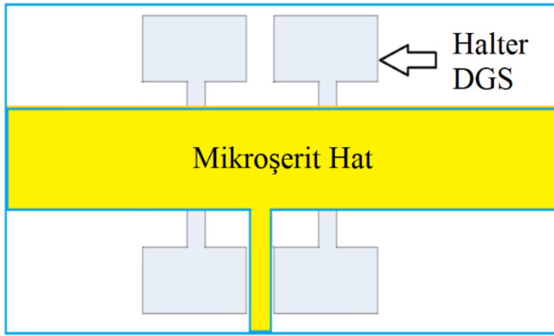
Şekil 4.15. Çift Halter DGS yapısı ile filtre tasarımı
