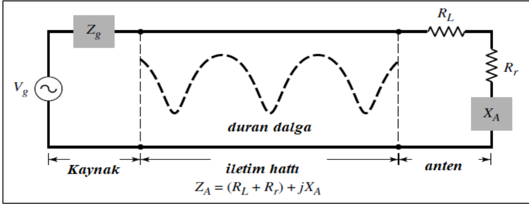
Şekil 2.2. Anten yapısının Thevenin eşdeğer devresi
