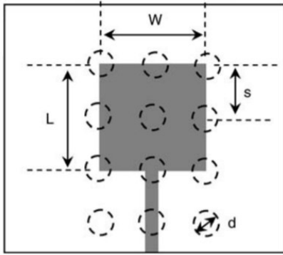
Şekil 4.16. Dairesel DGS uygulanan anten
