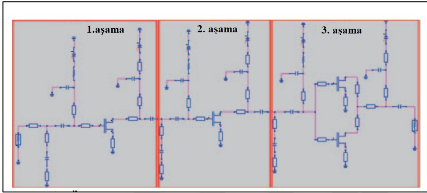
Şekil 6.4. Üç aşamalı MMIC LNA'nın şematiği
