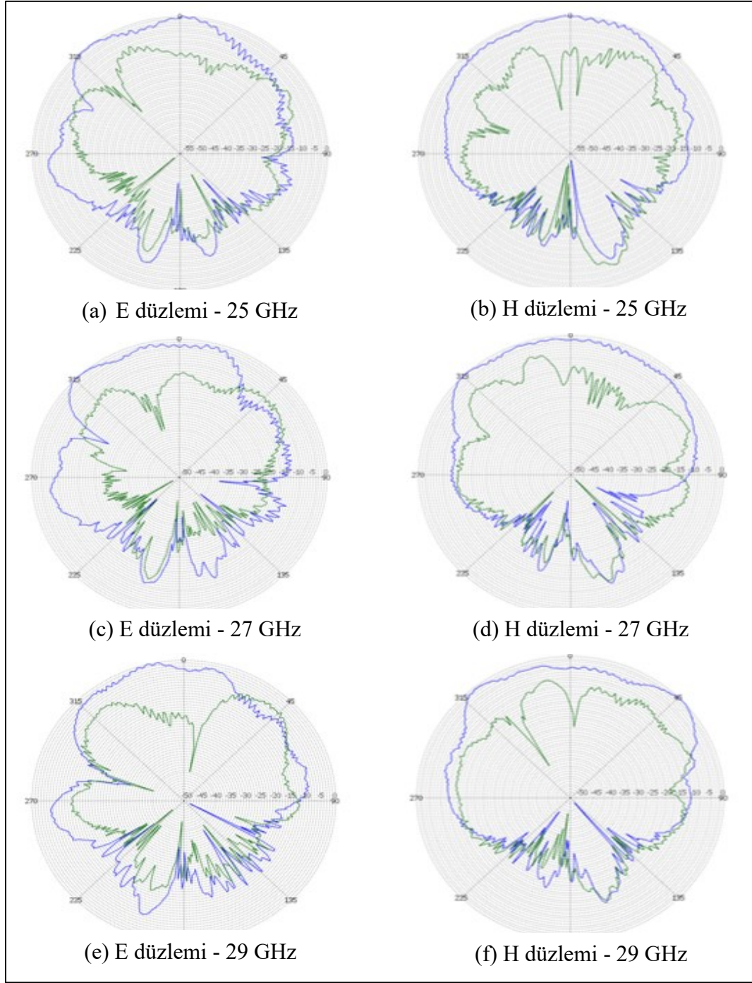
Şekil 8.8. 3D ışıma örüntüsünün ölçüm sonuçları (a) 25 GHz (c) 27 GHz (e) 29 GHz
