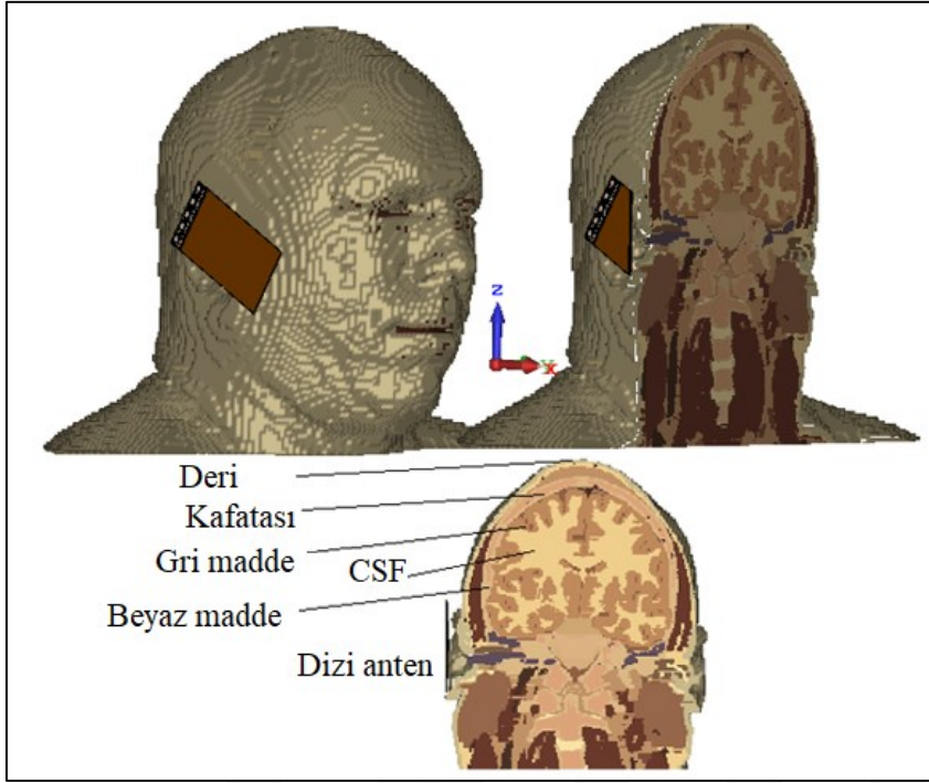
Şekil 5.11. CST paketinde yer alan Voxel Human tasarımı
