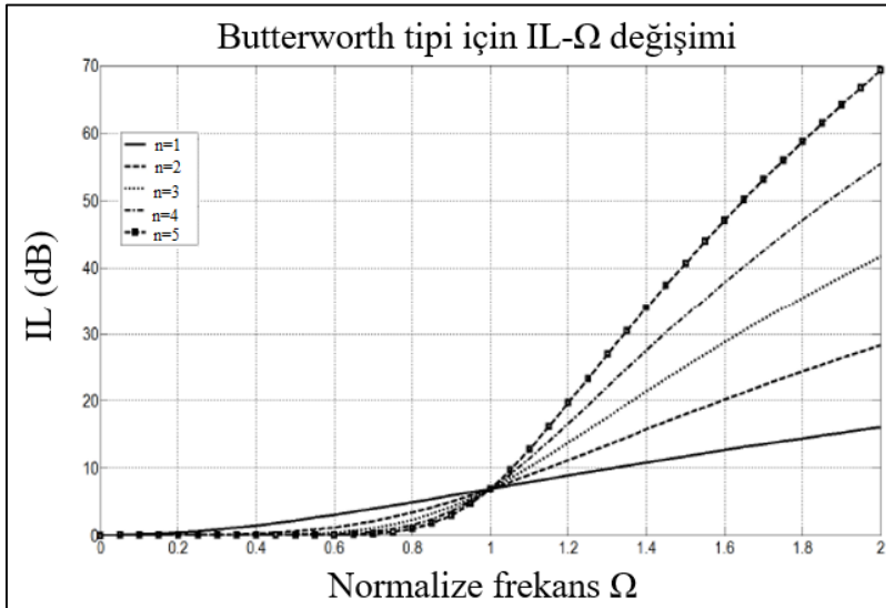
Şekil 3.8. Butterworth filtrenin farklı derecelerdeki zayıflama karakteristikleri [85]
