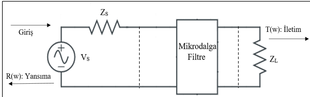
Şekil 3.1. İki kapılı mikrodalga filtre yapısı: R(\omega) ve T(\omega)
