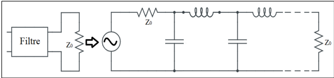
Şekil 3.5. AGK yöntemiyle filtre tasarımı
