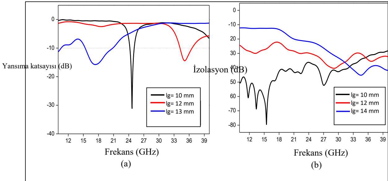
Şekil 8.2. (a) “lg” uzunluğunun yansıma katsayısına etkisi, (b) “lg” uzunluğunun izolasyona etkisi
