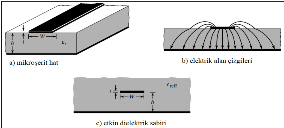
Şekil 2.8. Mikroşerit hat ve elektrik alan çizgileri
