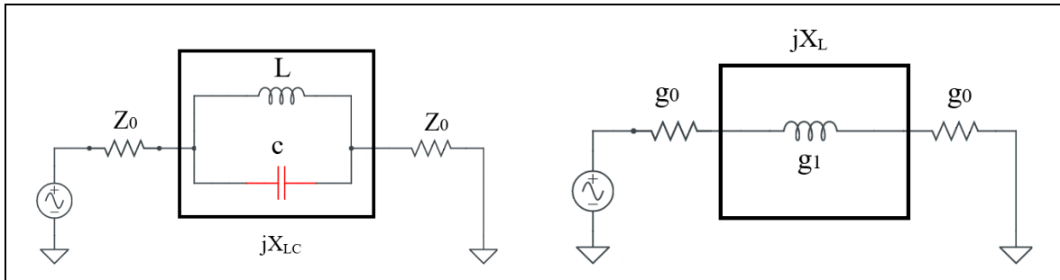
Şekil 4.12. (a). Halter DGS LC eşdeğer devresi (b). Butterworth alçak geçiren filtre
