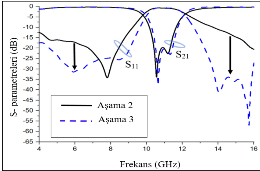
Şekil 7.9. Aşama-2 ve aşama-3 BSF simülasyon sonuçlarının karşılaştırılması
