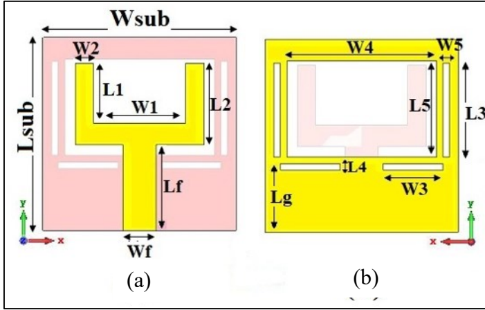
Şekil 5.3. Önerilen tekli antenin boyutları (a) üstten görünümü (b) alttan görünümü
