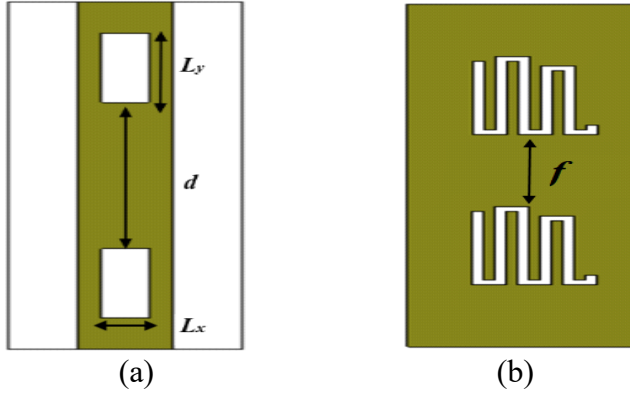
Şekil 7.5. Bant söndüren filtrenin geometrik yapısı (Aşama-2): (a) besleme yüzeyi (b) topraklama yüzeyi
