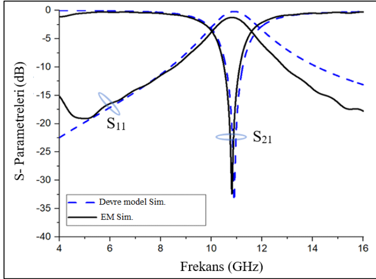
Şekil 7.3. EM simülasyon programı ile eşdeğer devre modelinin karşılaştırması (Adım-1)
