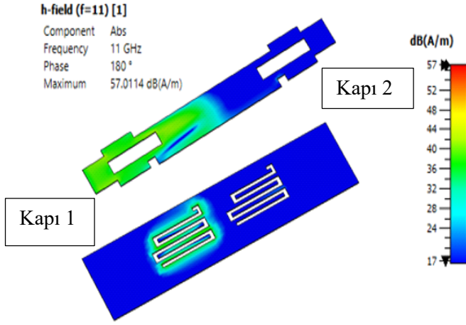
Şekil 7.12. Durdurma bandı (11 GHz) EM alan dağılımı
