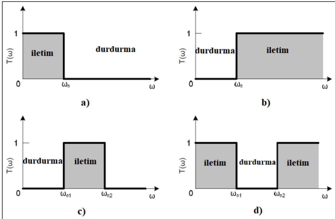
Şekil 3.2. İdeal filtre türleri: (a) alçak geçiren filtre; (b) yüksek geçiren filtre; (c) bant geçiren filtre; (d) bant durduran filtre
