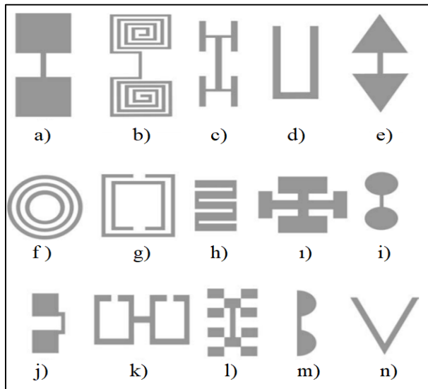
Şekil 4.3. Farklı DGS geometrileri
