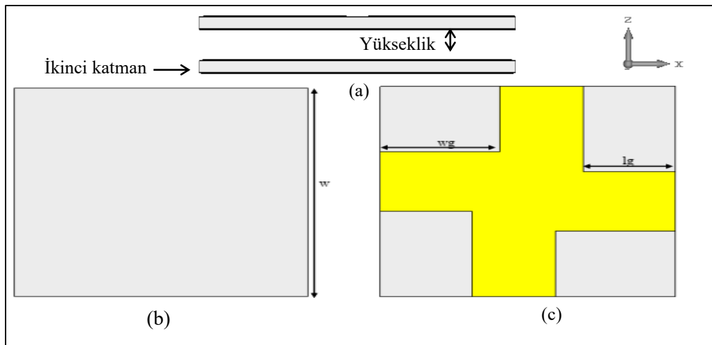
Şekil 8.4. Yansıtıcı olarak tasarlanan ikinci katman
