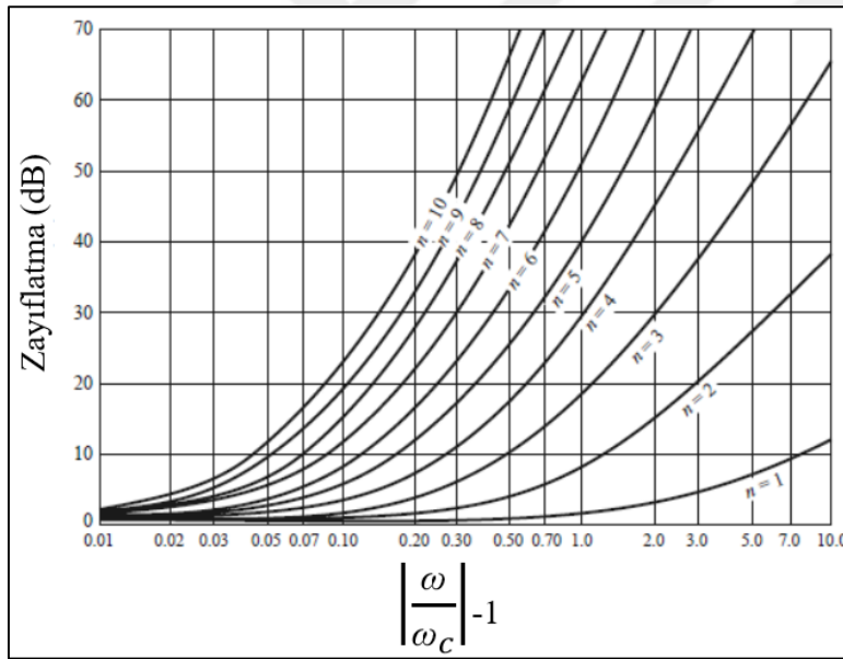
Şekil 3.10. Chebyshev filtrenin farklı derecelerdeki zayıflama karakteristikleri [85]
