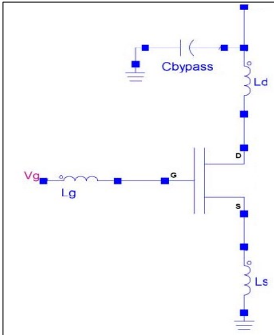
Şekil 6.3. Kaynak dejenerasyon tekniği
