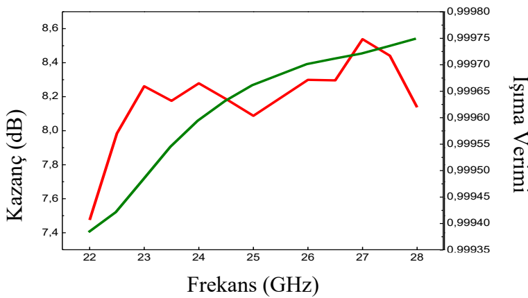
Şekil 8.10. Elde edilen kazanç ve verim grafiği (simülasyon)
