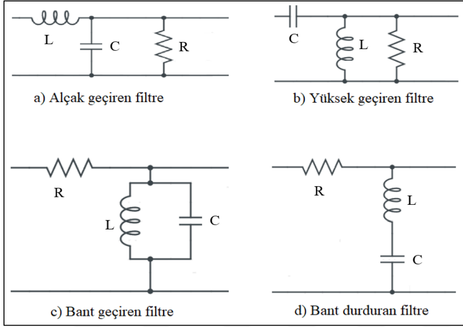
Şekil 3.3. İdeal filtre türlerine ait eşdeğer devreler (a) alçak geçiren filtre; (b) yüksek geçiren filtre; (c) bant geçiren filtre; (d) bant durduran filtre
