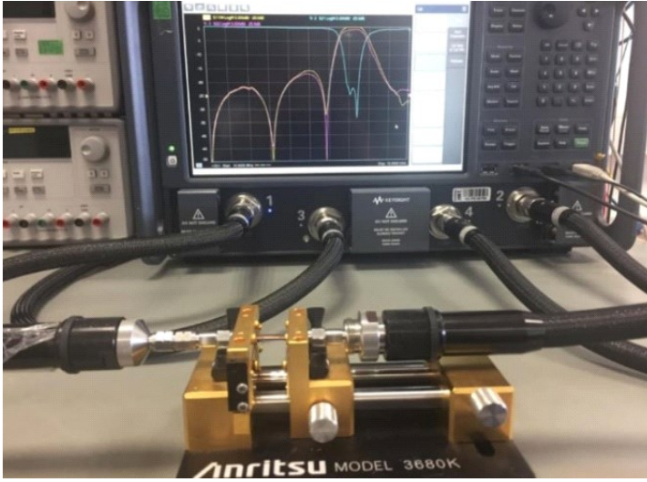
Resim 7.2. Bant söndüren filtre ölçüm düzeneği
