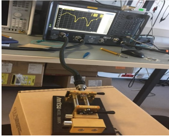
Resim 5.3. Ölçüm düzeneği
