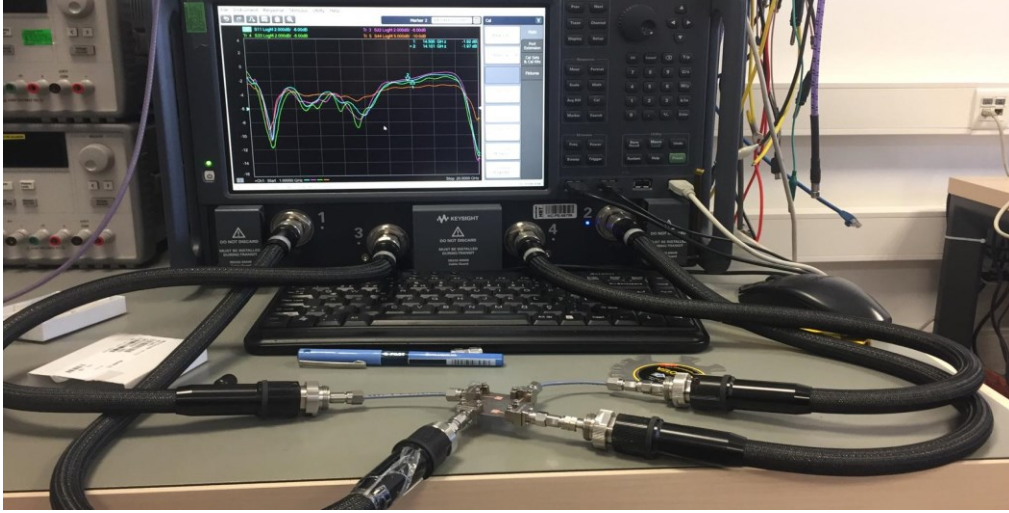
Resim 8.2. (c) S-parametre için ölçüm düzeneği
