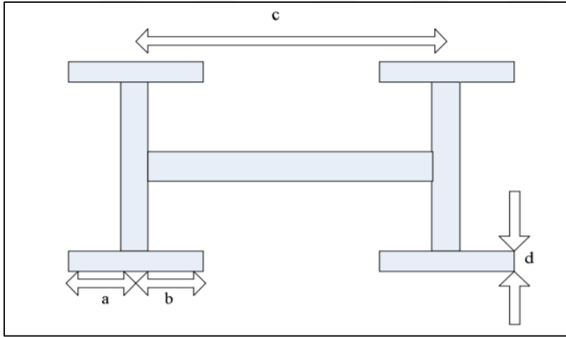
Şekil 4.6. H şekilli DGS
