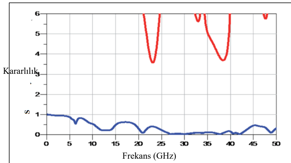
Şekil 6.10. MMIC LNA'nın kararlılık simülasyonu sonucu
