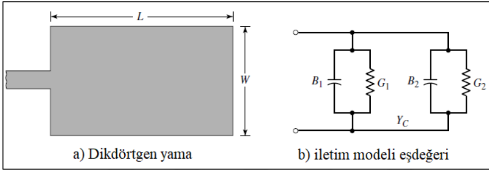
Şekil 2.10. Dikdörtgen mikroşerit anten için iletim hattı modeli eşdeğer devresi
