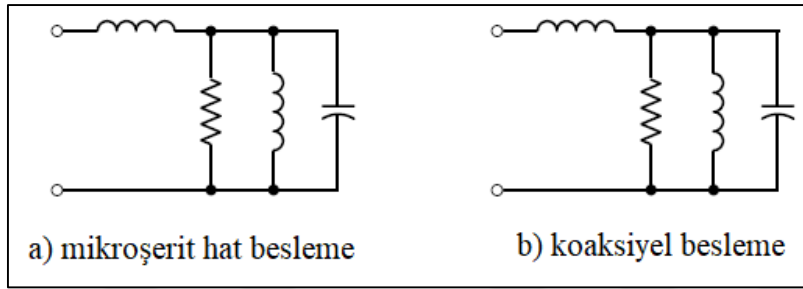
Şekil 2.7. Mikroşerit hat besleme türlerinin eşdeğer devreleri
