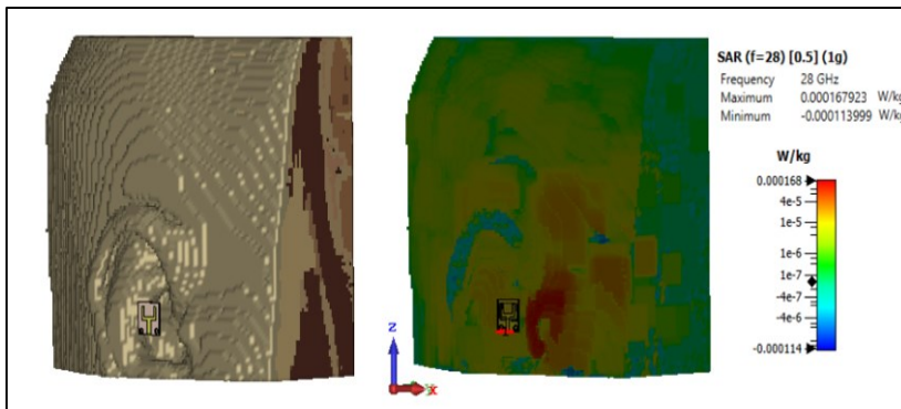
Şekil 5.12. Tekli anten SAR analizi
