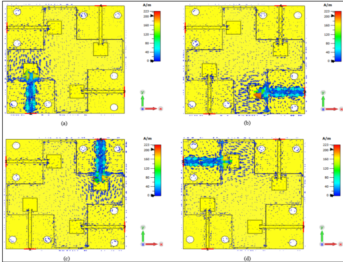
Şekil 8.3. (a) “lg” uzunluğunun akım dağılımına etkisi (a) anten 1, (b) anten 2, (c) anten 3, (d) anten 4
