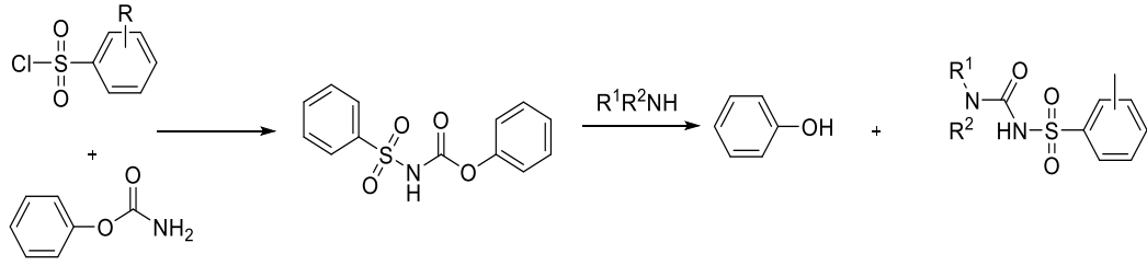
Şekil 2.18. Sülfonil üre sentezi için farklı bir yaklaşım [40]
