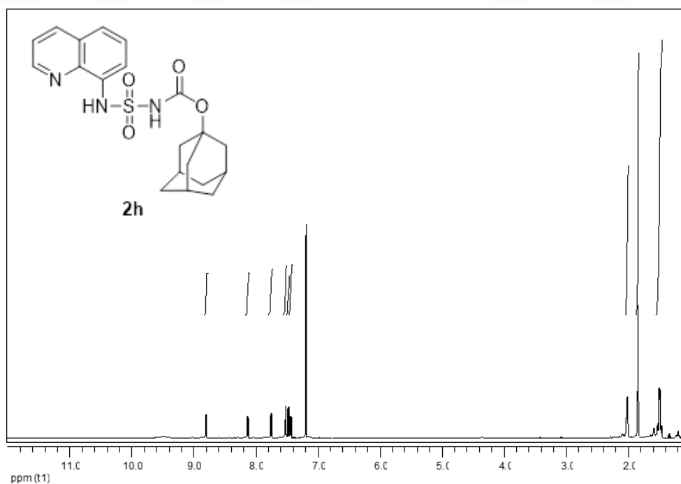
EK 22: 2h numaralı bileşiğin ^1\text{H} NMR spektrumu
