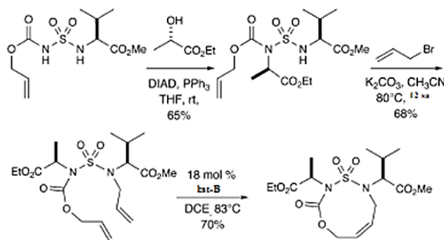
Şekil 2.13. Sülfonil karbamat sentezi için bir yöntem [6]
