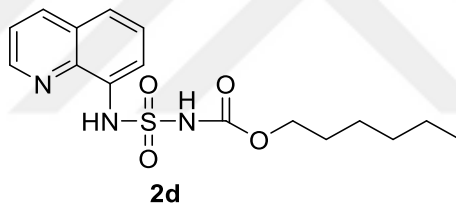
Şekil 4.4. 2d numaralı bileşiğin yapısı
