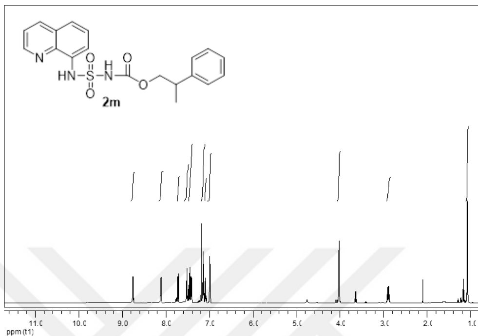
EK 37: 2m numaralı bileşiğin ^1\text{H} NMR spektrumu
