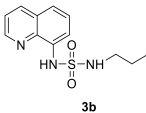
Şekil 4.17. 3b numaralı bileşiğin yapısı
