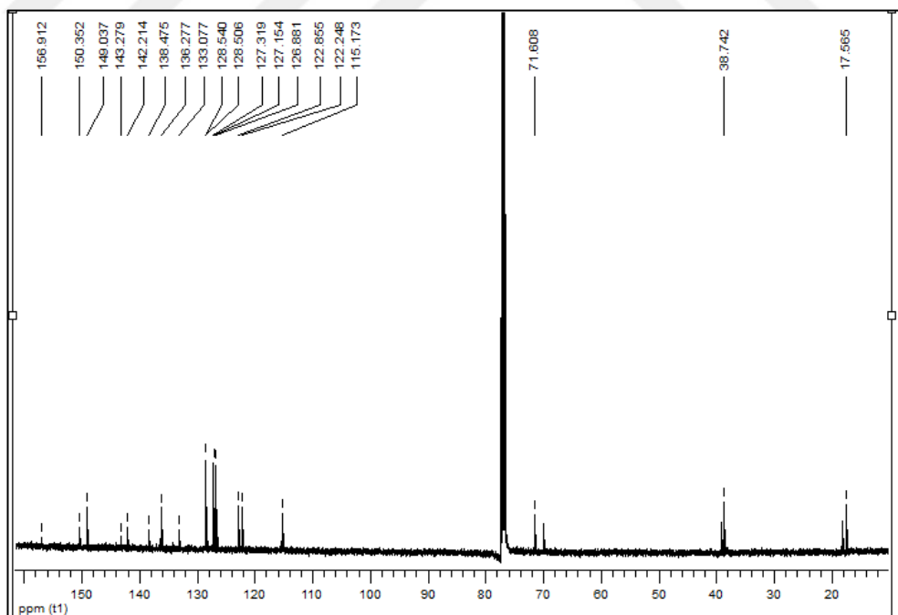
EK 38: 2m numaralı bileşiğin ^{13}\text{C} NMR spektrumu
