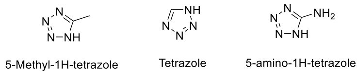
Şekil 2.11. Tetrazol grupları
