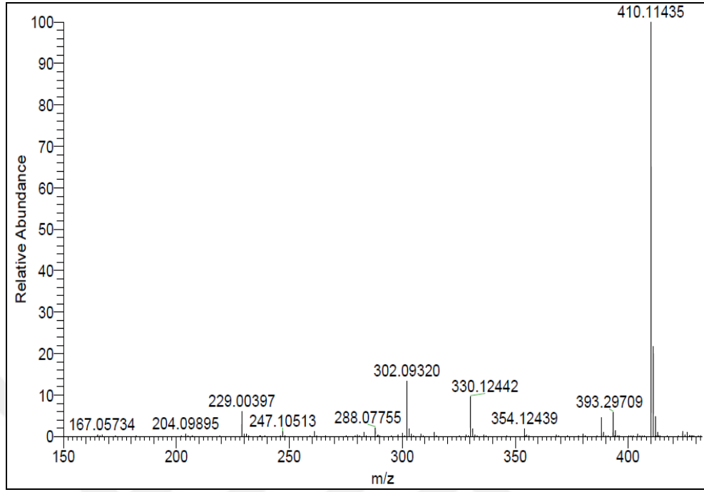
EK 81: 31 numaralı bileşğin kütle spektrumu
