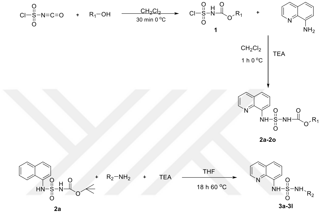
Şekil 3.1 8-aminokinolin bileşiğinin sülfamoil karbamat ve sülfonamid türevlerinin sentezinin genel şeması
