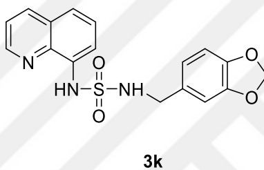
Şekil 4.26. 3k numaralı bileşiğin yapısı
