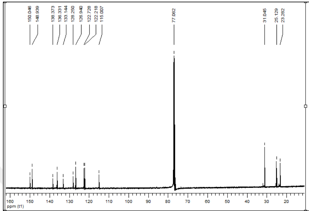
EK 17: 2f numaralı bileşiğin ^{13}\text{C} NMR spektrumu
