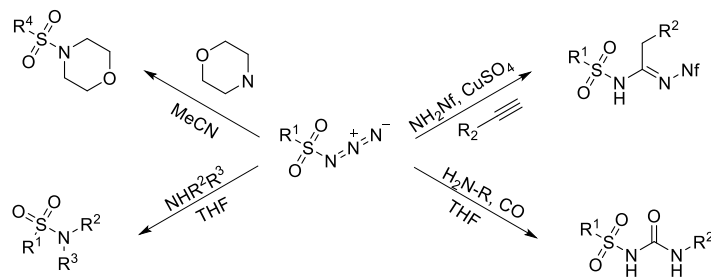
Şekil 2.9. Sülfonamid, sülfonil üre ve sülfonil karbamatların sentezi [27]
