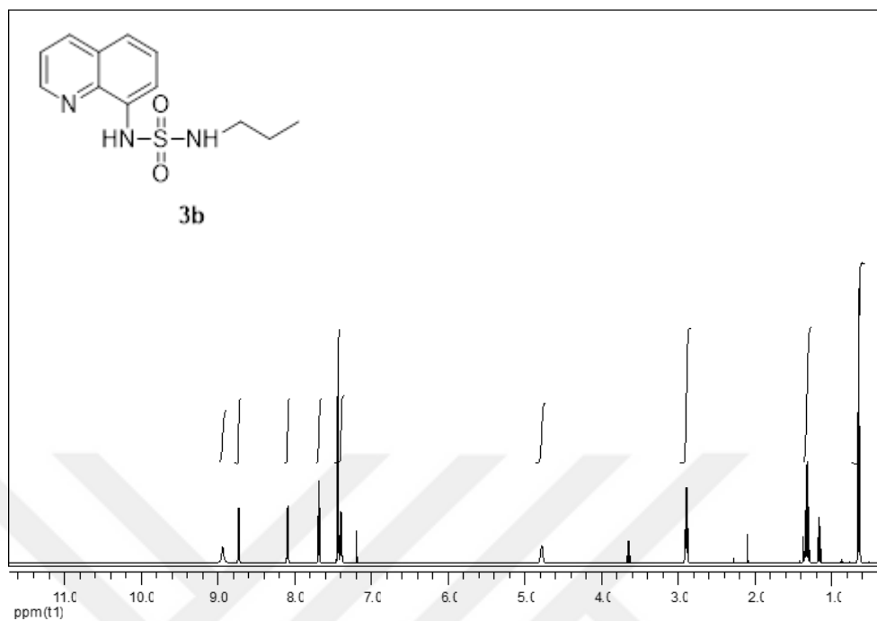
EK 49: 3b numaralı bileşiğin ^1\text{H} NMR spektrumu
