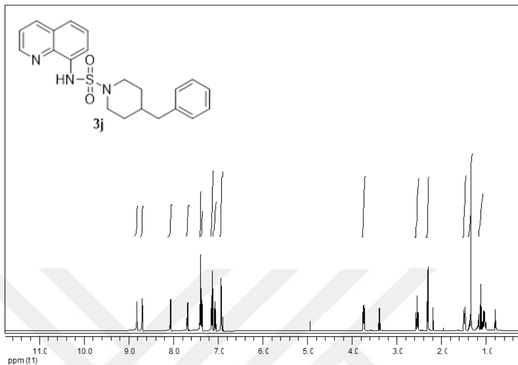
EK 73: 3j numaralı bileşiğin ^1\text{H} NMR spektrumu
