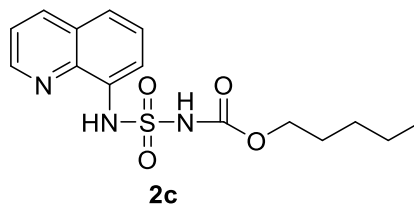
Şekil 4.3. 2c numaralı bileşiğin yapısı
