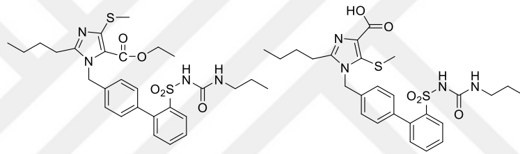
Şekil 2.10. Kardiyovasküler hastalıkların tedavisin de kullanılan bazı sülfamoil bileşikler [30]
