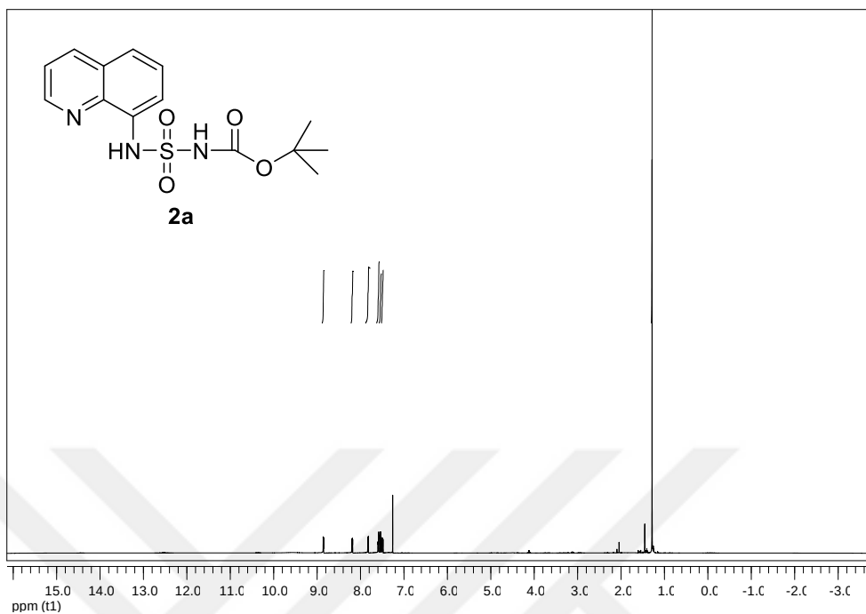
EK 1: 2a numaralı bileşiğin ^1\text{H} NMR spektrumu
