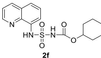
Şekil 4.6. 2f numaralı bileşiğin yapısı
