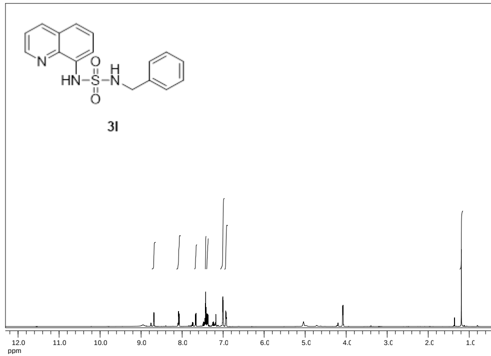
EK 70: 3i numaralı bileşiğin ^1\text{H} NMR spektrumu
