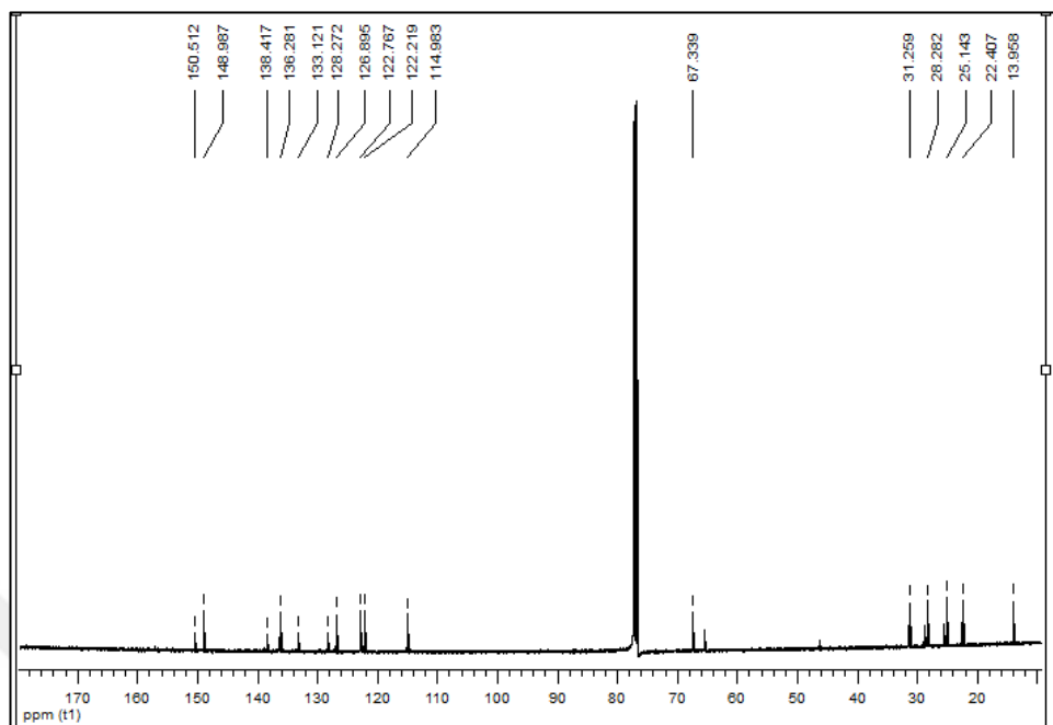
EK 11: 2d numaralı bileşiğin ^{13}\text{C} NMR spektrumu
