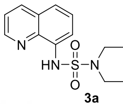
Şekil 4.16. 3a numaralı bileşiğin yapısı
