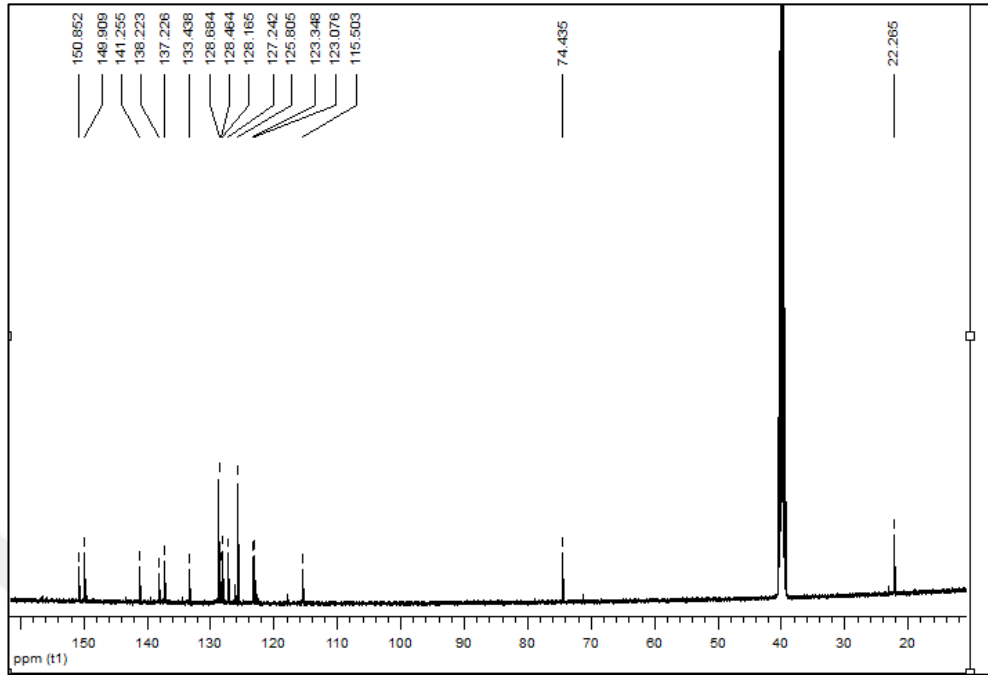
EK 35: 21 numaralı bileşiğin ^{13}\text{C} NMR spektrumu
