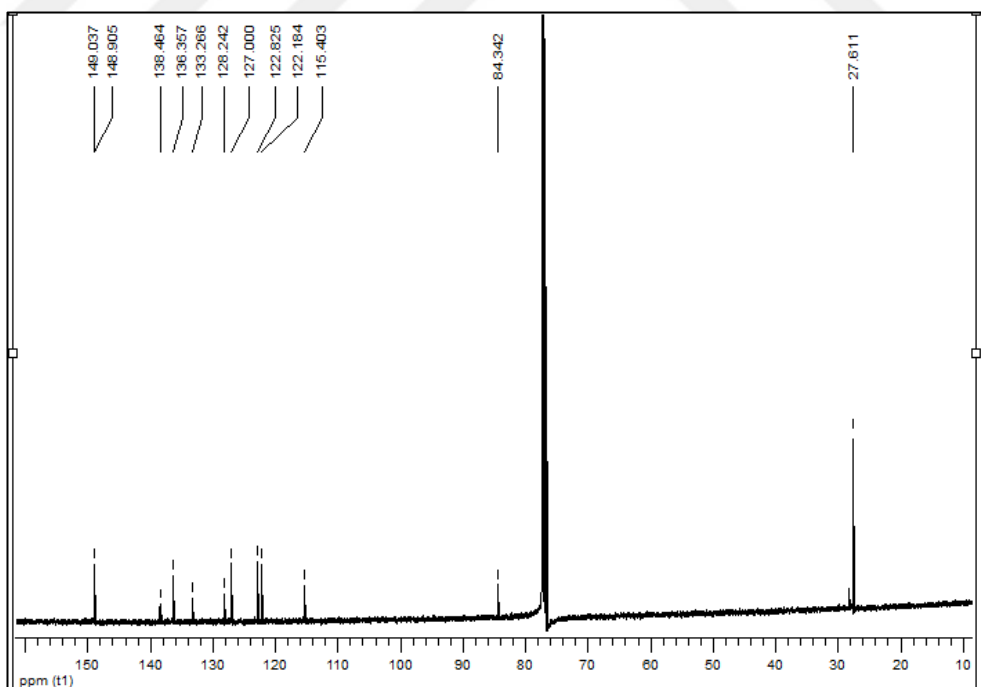
EK 2: 2a numaralı bileşiğin ^{13}\text{C} NMR spektrumu
