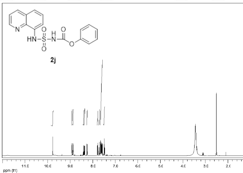
EK 28: 2j numaralı bileşiğin ^1\text{H} NMR spektrumu
