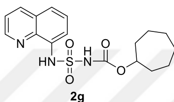
Şekil 4.7. 2g numaralı bileşiğin yapısı
