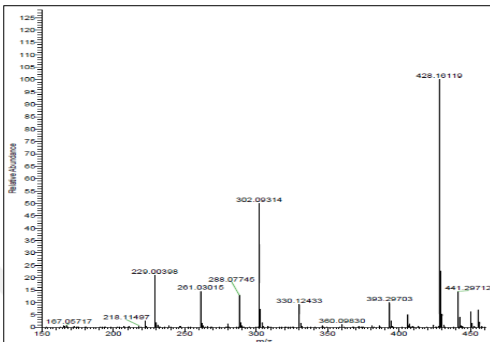
EK 27: 2i numaralı bileşiğin kütle spektrumu
