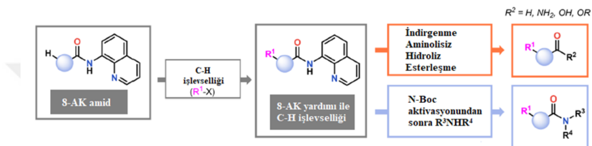
Şekil 2.3. Foksiyonelleşmiş C-H ürünlerini 8-amino kinolin yardımıyla farklı bileşik sınıflarına dönüştürülmesine yönelik yaklaşımlar [11].
