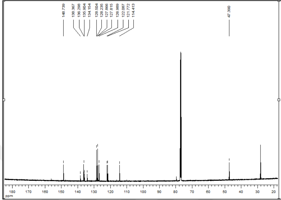
EK 71: 3i numaralı bileşiğin ^{13}\text{C} NMR spektrumu
