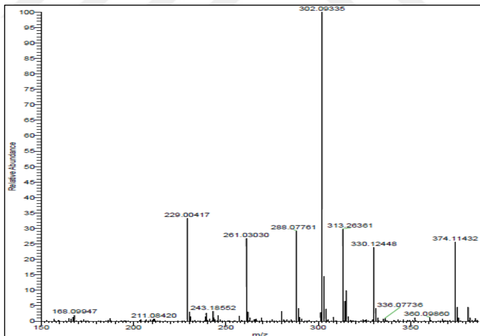
EK 12: 2d numaralı bileşiğin kütle spektrumu
