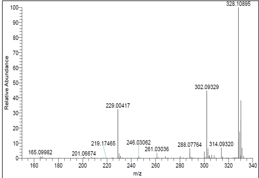
EK 66: 3g numaralı bileşiğin kütle spektrumu
