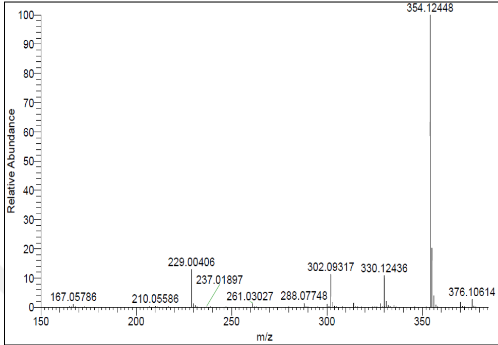
EK 69: 3h numaralı bileşiğin kütle spektrumu
