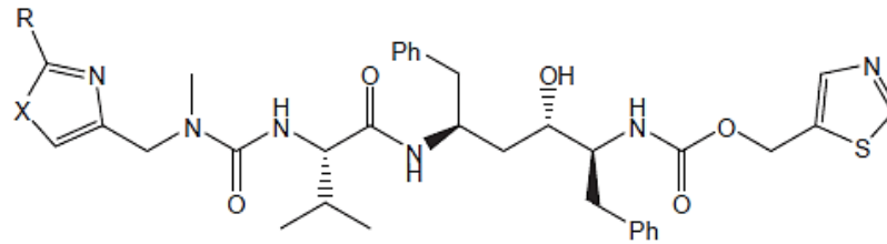
Şekil 2.17. Ritonavir yapısı [35]
