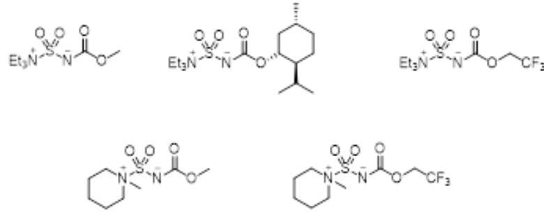
Şekil 2.6. Yeni nesil Burgess reaktifleri [23].
