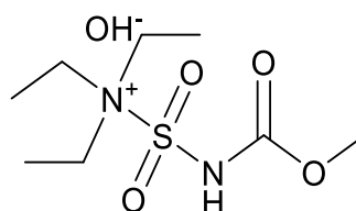
Şekil 2.4 İlk Burgess reaktifi ([metoksikarbonilsulfamoil]triethylamonyum hidroksit tuzu) [22].
