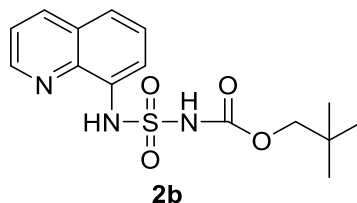
Şekil 4.2. 2b numaralı bileşiğin yapısı
