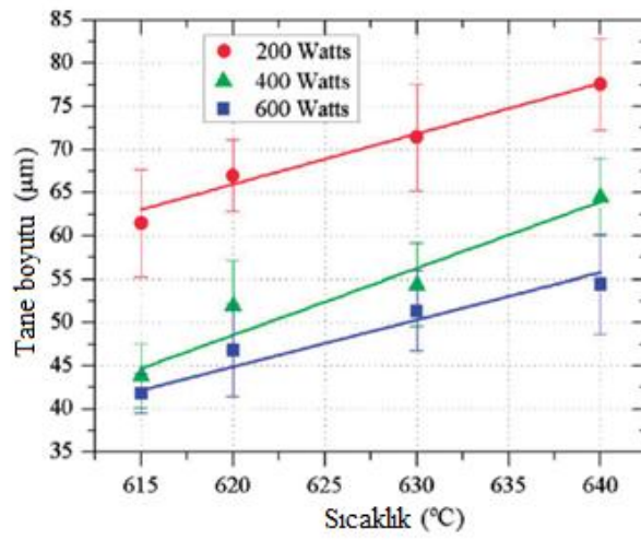
Şekil 2.8 19.8 kHz frekansta farklı sıcaklık ve elektrik gücüne karşılık tane boyutunda meydana gelen değişim (Puga ve diğerleri, 2011)
