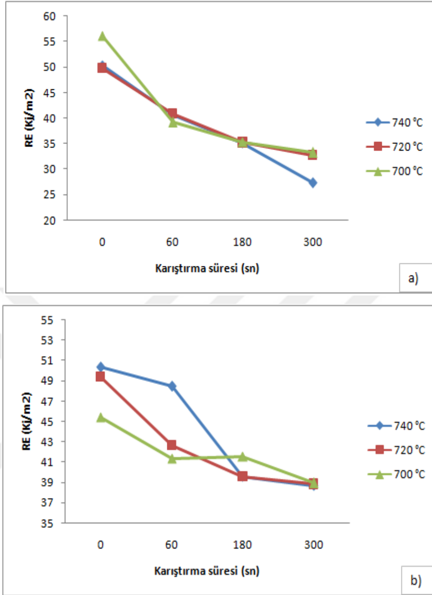
Şekil 4.9 Charpy darbe testi sonuçları a) 2 kg, b) 4 kg
