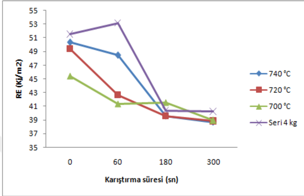
Şekil 4.10 4 kg lık seri üretim ve laboratuvar denemelerine ait charpy darbe testi sonuçları
