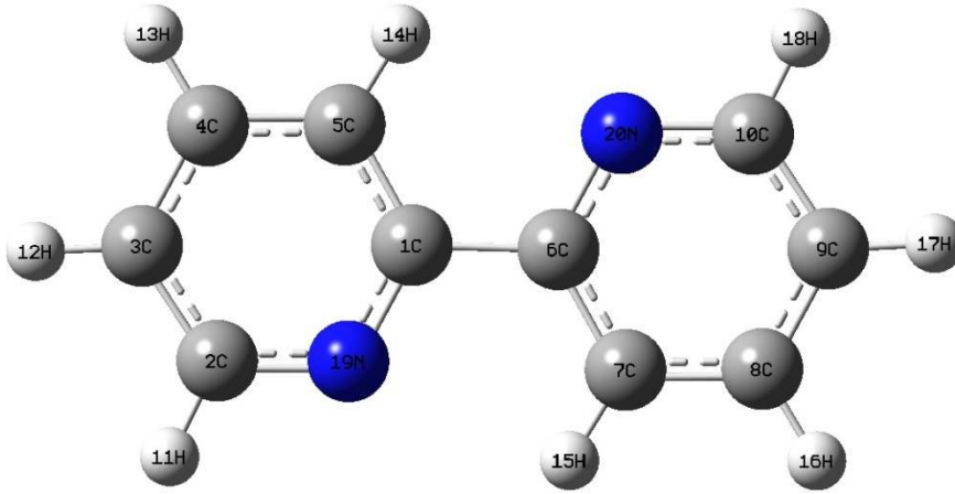
Şekil 5.19. 2,6'-bpy molekülünün yapısı
