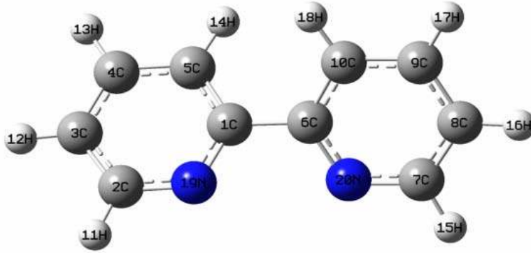
Şekil 5.2. cis -2,2'-bpy
