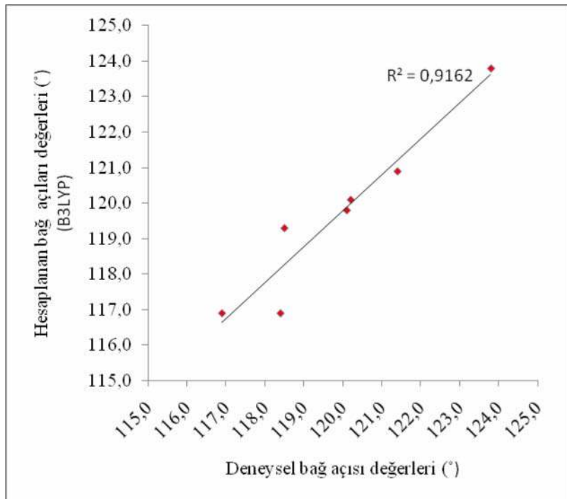
Şekil 5.41. 4,4'-bpy molekülünün hesaplanan bağ açılarının deneysel değerlere karşı korelasyonu
