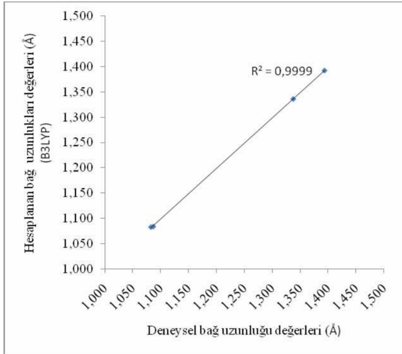
Şekil 5.40. 4,4'-bpy molekülünün hesaplanan bağ uzunluklarının deneysel değerlere karşı korelasyonu
