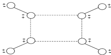
Şekil 2.11. Düzlem dışı açılı bükülme
