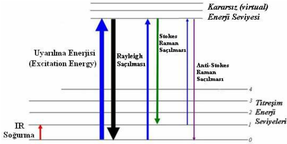
Şekil 2.2. IR soğurma ve Raman saçılmasının şematik gösterimi
