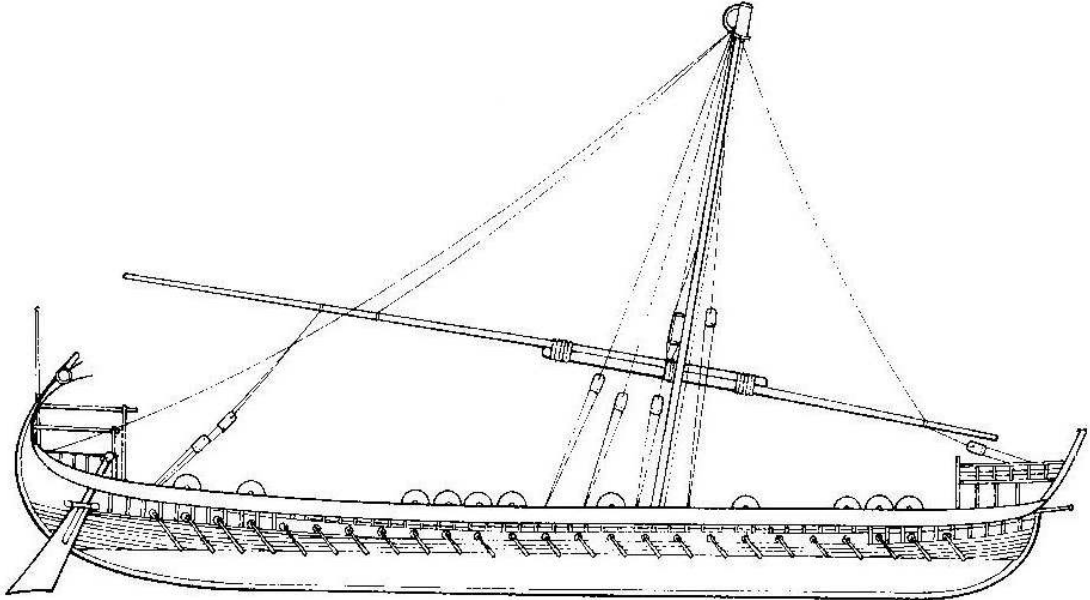
VII. yüzyıl Bizans Dromonunun rekonstrüksiyonu. Bu gemi sürat ve yüksek manevra kabiliyeti gözetilerek inşa ediliyordu. (Matthew Bennett-J. Bradbury, Ortaçağ Dünya Savaş Tarihi "Teçhizat, Savaş Yöntemleri, Taktikler 500-1500" , c. I, (çev. Özgür Kolçak), c. I, İstanbul, 2011, s. 212.)
