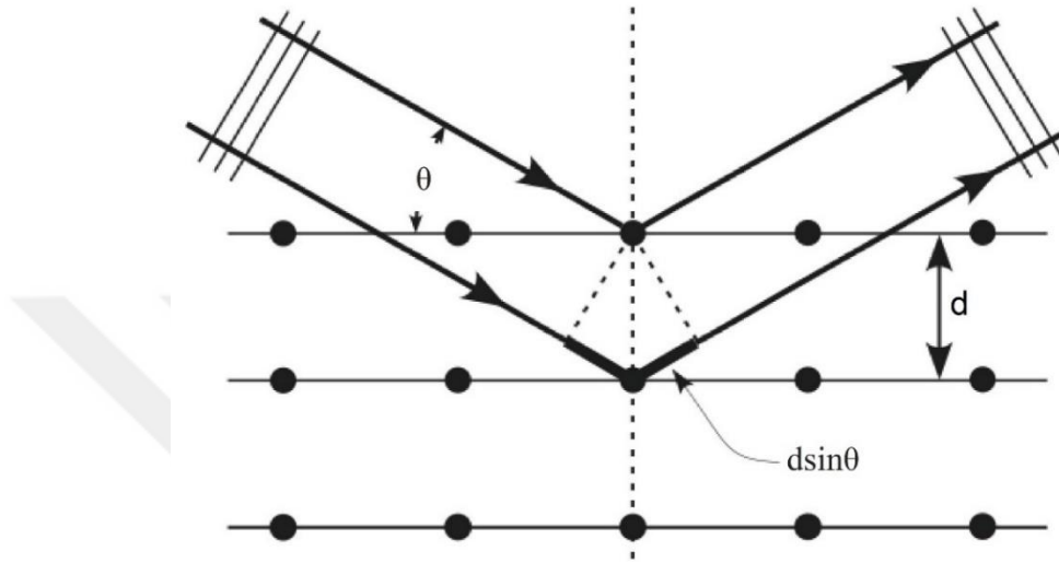
Şekil 4.5. XRD difraktometre sisteminin şematik diyagramı
