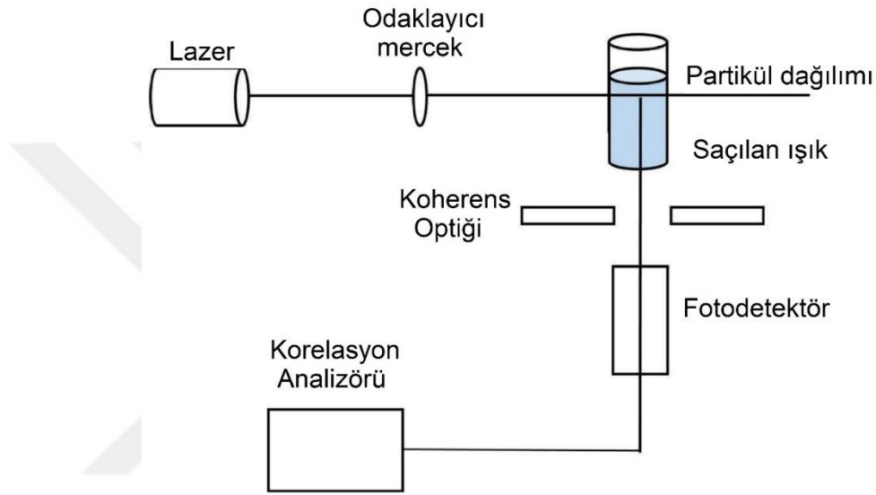
Şekil 4.6. DLS cihazının şematik gösterimi (Alam vd., 2025)
