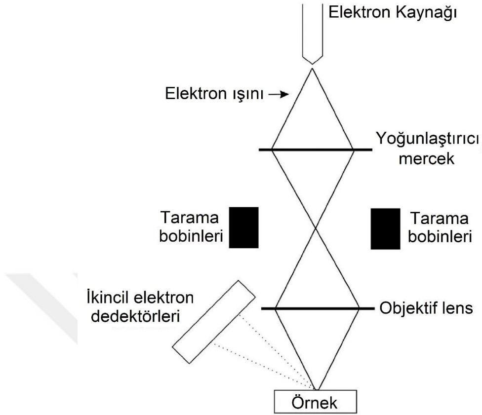
Şekil 4.3. Taramalı elektron mikroskobunun (SEM) çalışma prensibi (Kumar vd., 2019)
