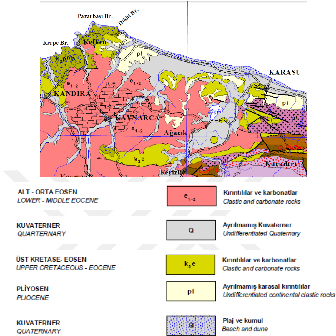
Şekil 2.6. Araştırma Alanının Jeolojik Yapısı
