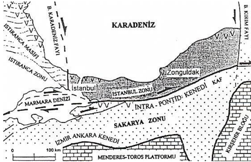
Şekil 2.5. Bölgedeki Temel Kayaların ait olduğu Sakarya ve İstanbul Zonları
