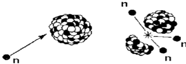
Şekil 1.7. Fisyon
