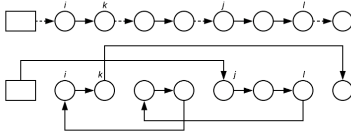
Şekil 4.10 Rota içi k-değişim komşuluğu düz yönlü örneği
