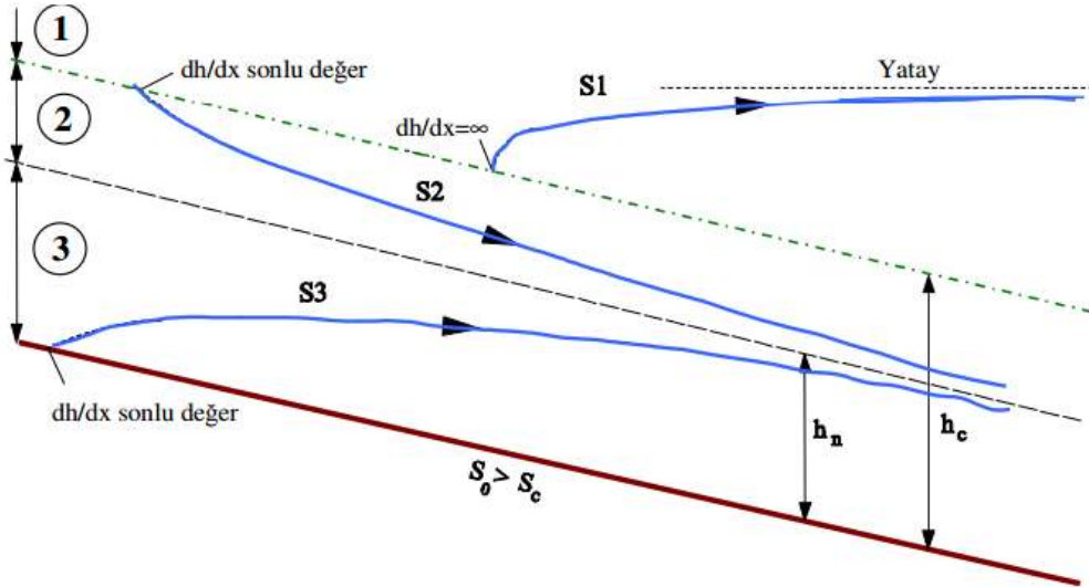
Şekil 3.12. S Profilleri
