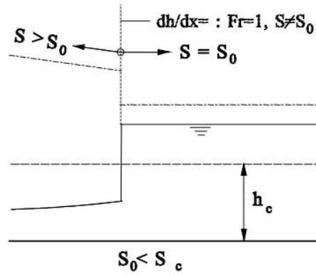
Şekil 3.10. Hidrolik sıçramanın oluştuğu durum
