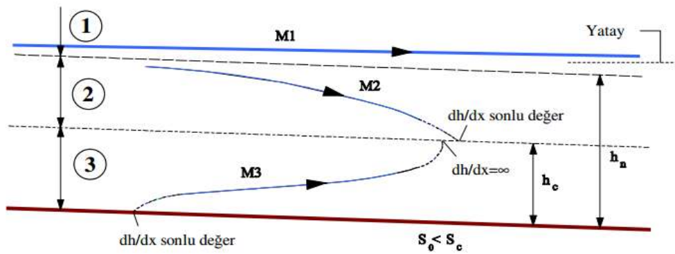
Şekil 3.11. M Profilleri
