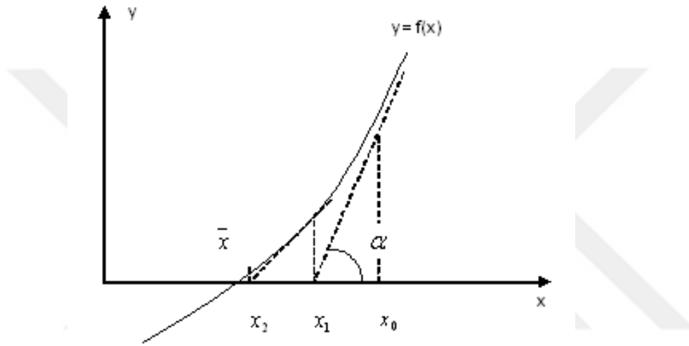
Şekil 3.15. Newton-Raphson metodunun grafiksel gösterilimi
