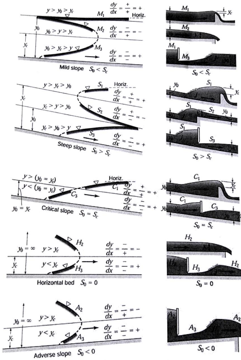
Şekil 3.6. Su yüzü profilleri ( Mild:Yumuşak eğim, Steep:Sert eğim , Critical: Kritik eğim, Horizontal: Yatay, Adverse: Ters eğim)
