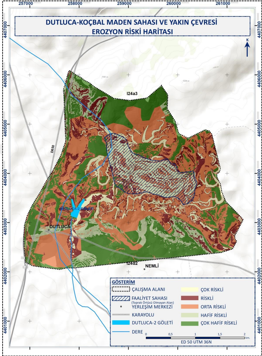
Şekil 4.19. Çalışma alanına ait erozyon riski analizi haritası
