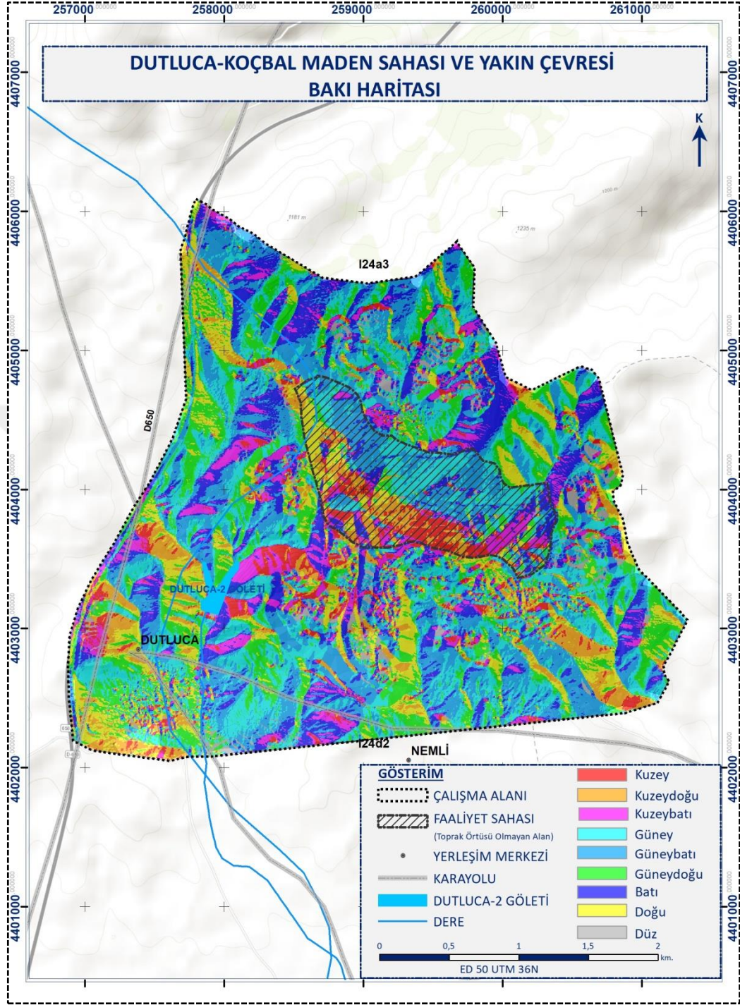
Şekil 4.3. Çalışma alanı bakı durumu haritası
