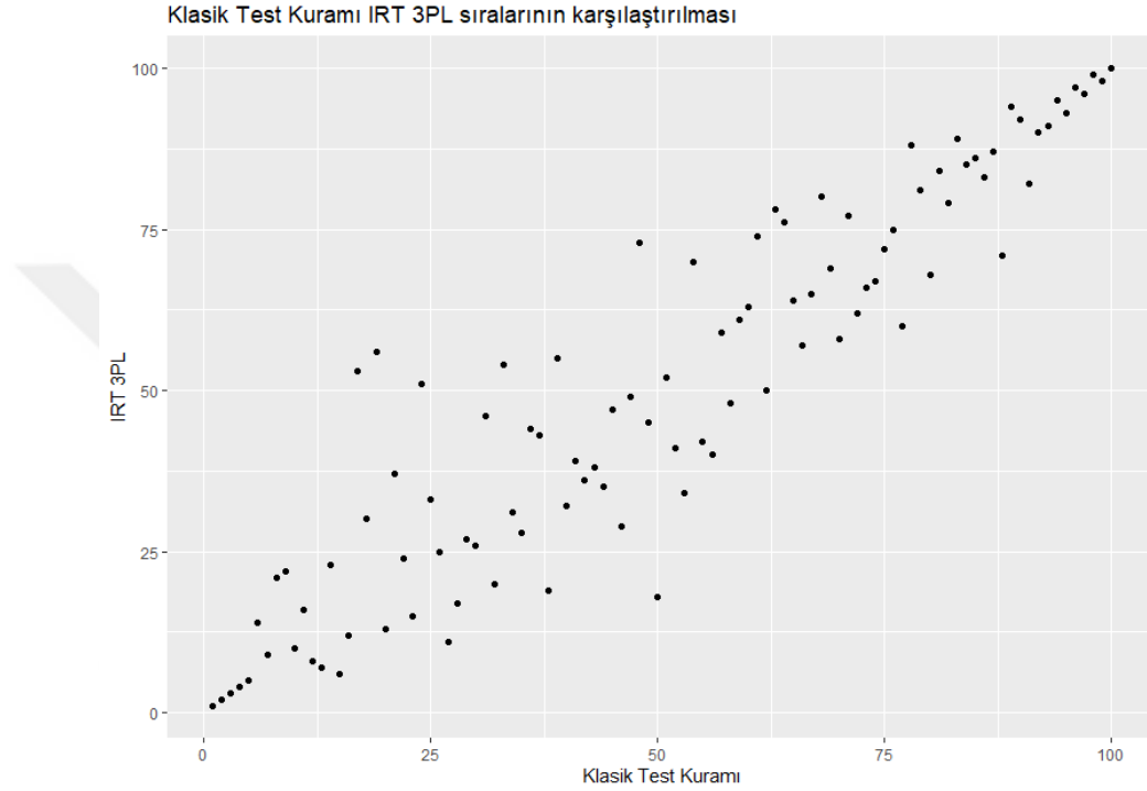
Grafik 4.25. “Routing” yöntemine göre üretilmiş normal olmayan (sola çarpık) dağılıma sahip 100 kişilik veri seti için KTK ve IRT 3PL puan sıralarının karşılaştırması
