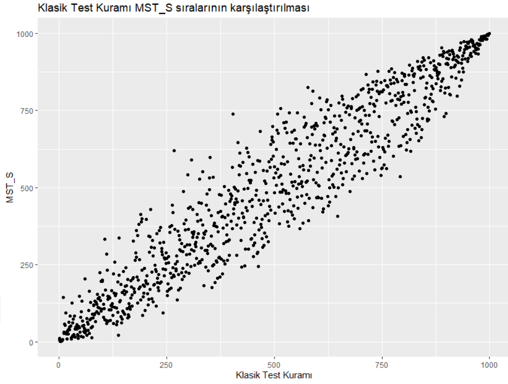
Grafik 4.38. “Shaping” yöntemine göre üretilmiş normal olmayan (sola çarpık) dağılıma sahip 1000 kişilik veri seti için KTK ve MST-S puan sıralarının karşılaştırması
