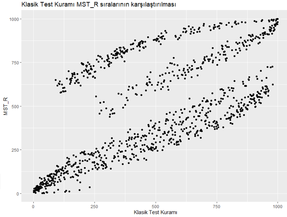
Grafik 4.11. “Routing” yöntemine göre üretilmiş normal dağılıma sahip 1000 kişilik veri seti için KTK ve MST-R puan sıralarının karşılaştırması
