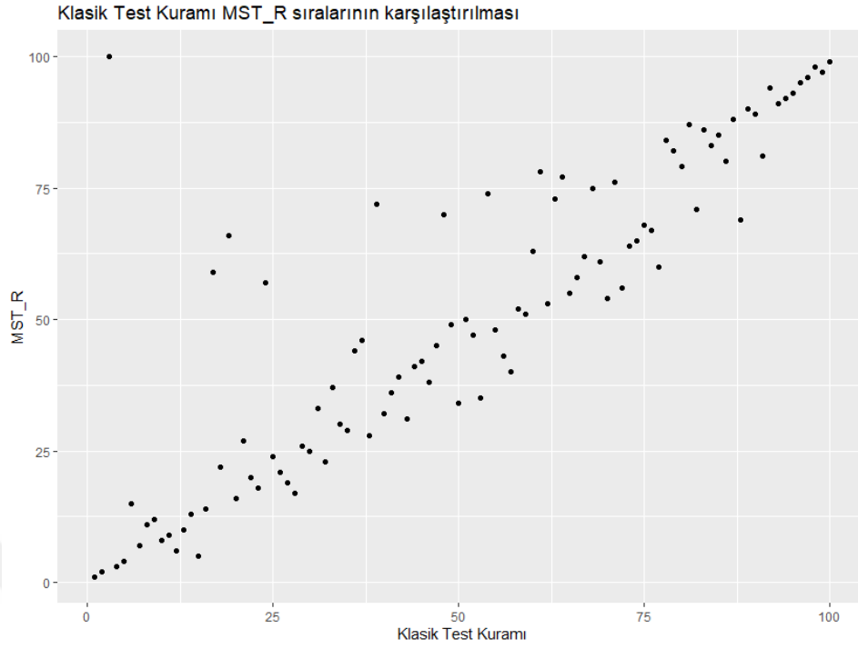
Grafik 4.26. “Routing” yöntemine göre üretilmiş normal olmayan (sola çarpık) dağılıma sahip 100 kişilik veri seti için KTK ve MST-R puan sıralarının karşılaştırması
