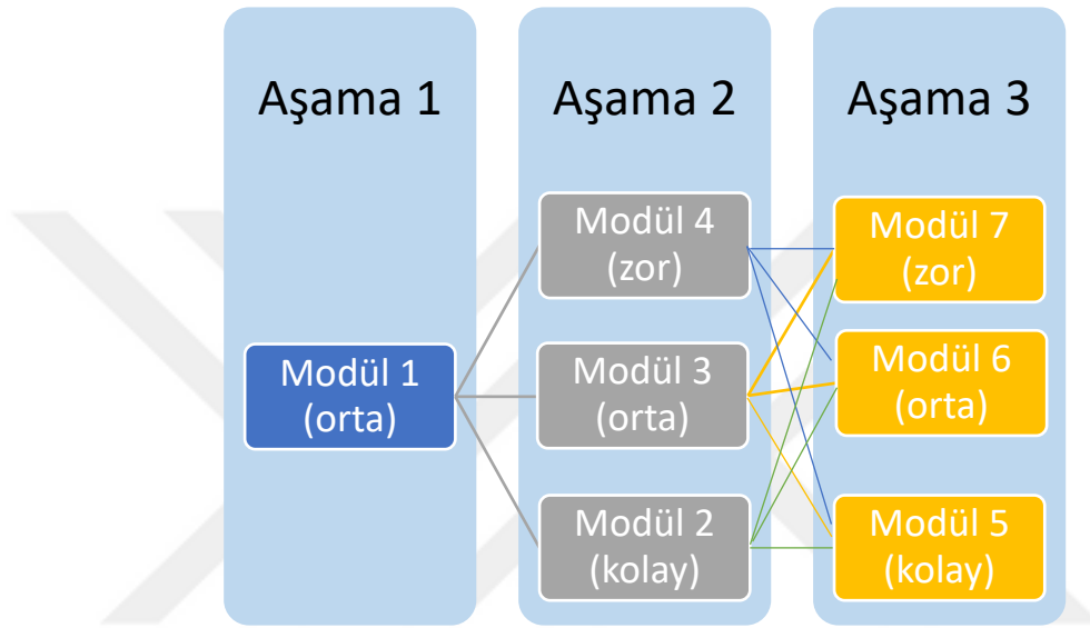
Şekil 3. 1. MST (Multistage Testing) test sunum yapısının simülatif modül ve panel montajı
