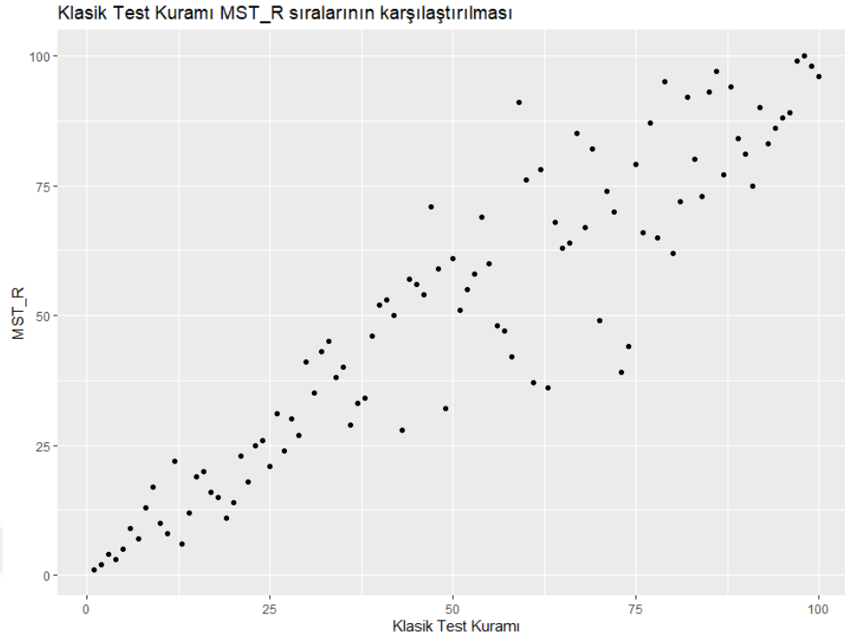
Grafik 4.44. “Routing” yöntemine göre üretilmiş normal olmayan (sağa çarpık) dağılıma sahip 100 kişilik veri seti için KTK ve MST-R puan sıralarının karşılaştırması
