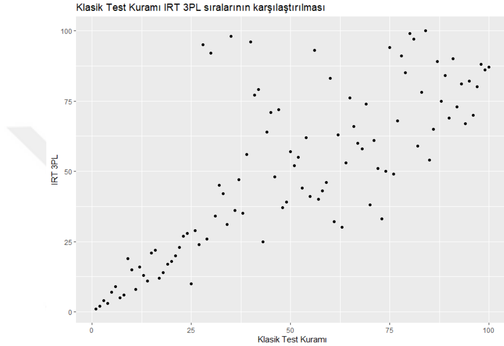
Grafik 4.43. “Routing” yöntemine göre üretilmiş normal olmayan (sağa çarpık) dağılıma sahip 100 kişilik veri seti için KTK ve IRT 3PL puan sıralarının karşılaştırması
