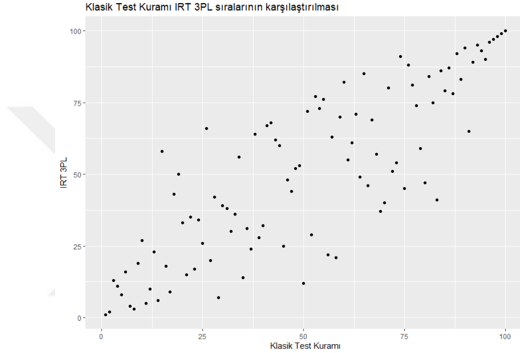
Grafik 4.7. “Routing” yöntemine göre üretilmiş normal dağılıma sahip 100 kişilik veri seti için KTK ve IRT 3PL puan sıralarının karşılaştırması
