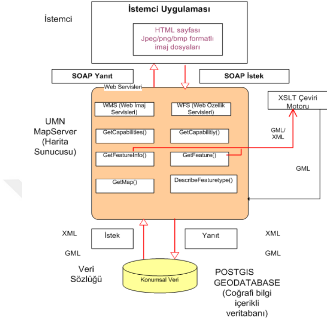
Şekil 2.11. Web Servis Sistem Mimarisi (Turan, 2006)
