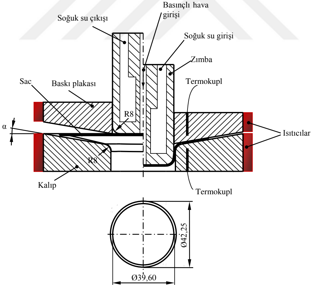
Şekil 4.2. Deneylerde kullanılan kalıp geometrileri, ölçüler mm
