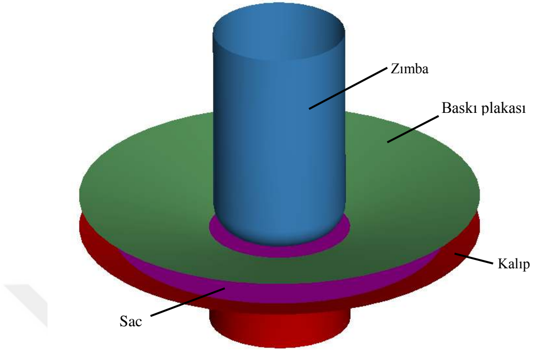
Şekil 4.6. Kalıp elemanlarının oluşturulması
