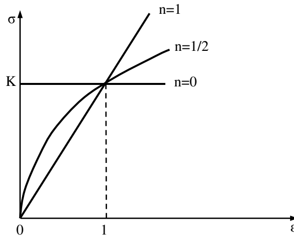
Şekil 3.15. Pekleşme üstelinin gerçek gerilme-gerçek şekil değişimine etkisi \sigma_g = K \cdot \varepsilon^n [64].
