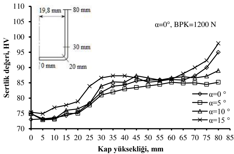
Şekil 5.69. \beta=2,75 için kalıp açısının( \alpha ) 250°C’de sertlik dağılımı üzerindeki etkisi
