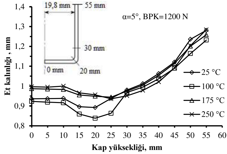
Şekil 5.55. \beta=2,17 için şekillendirme sıcaklığının et kalınlığı üzerindeki etkisi
