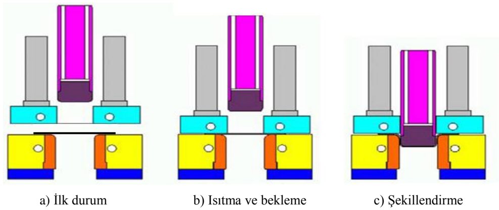
Şekil 4.3. İlk derin çekme işlem sıralaması
