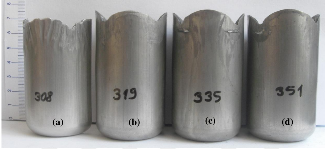
Şekil 5.18. 250 °C ve 1200 N BPK sonucunda elde edilen numuneler a) \alpha=0^\circ b) \alpha=5^\circ c) \alpha=10^\circ d) \alpha=15^\circ
