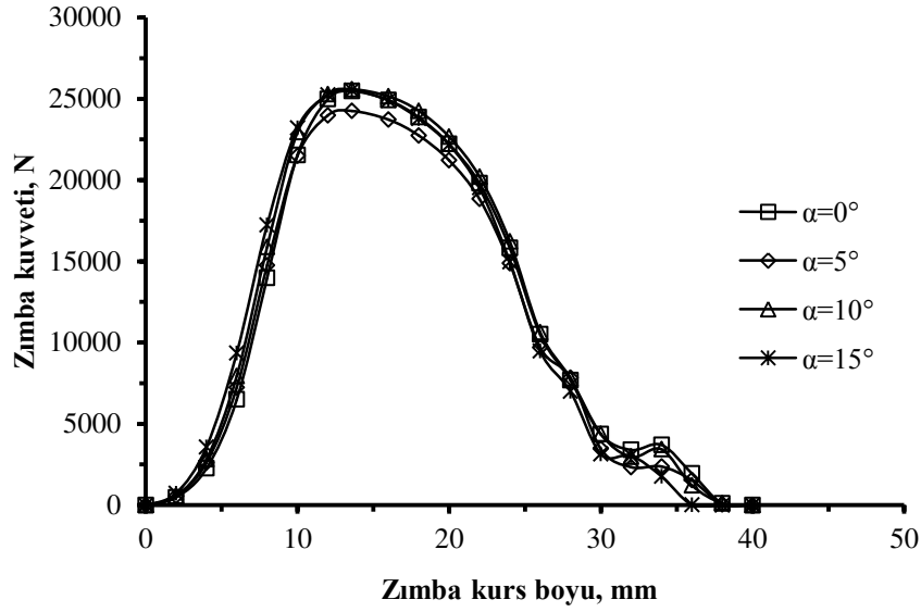
Şekil 5.17. T=175 °C sıcaklık ve 3600 N BPK sonucundaki zimba kuvvetleri değişimi
