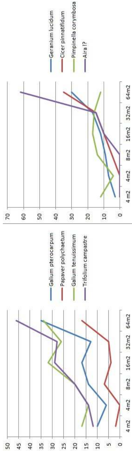
Şekil 4.6. Galium pterocarpum örneklik alanı bitkilerinin parsellerde bulunma durumları
