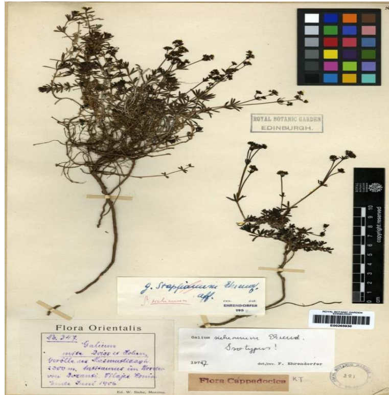
Şekil 3.5. Galium sieheanum Ehrend.
