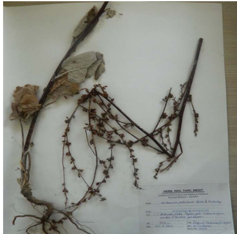
Şekil 3.11. V. Petiolare Boiss. et Kotschy (Ç.Ü. ADA Herbaryumu)
