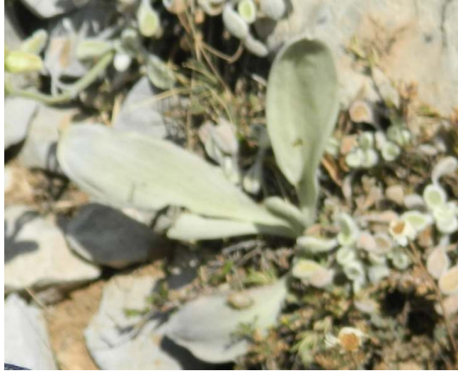
Şekil 4.10. Scorzonera boissieri Lipschitz.
