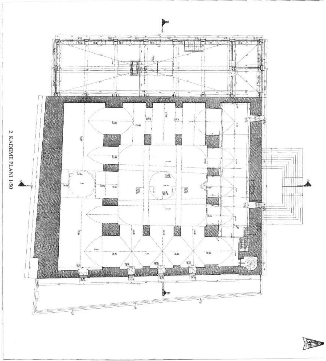
Ek 12: Caminin ikinci kademe planı (Vakıflar Genel Müdürlüğü Arşivi'nden)
