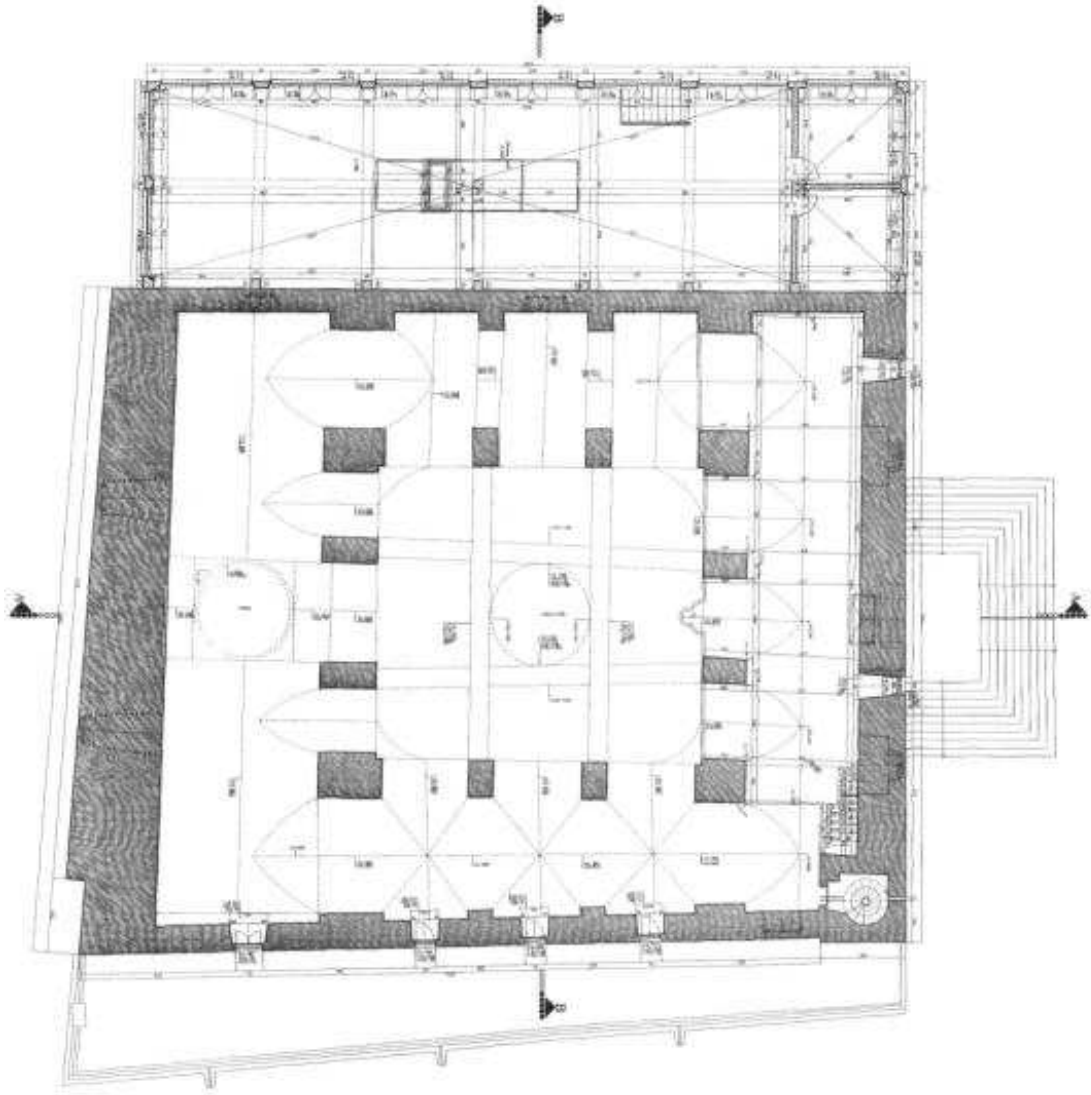
Ek 11: Caminin birinci kademe planı (Vakıflar Genel Müdürlüğü Arşivi'nden)
