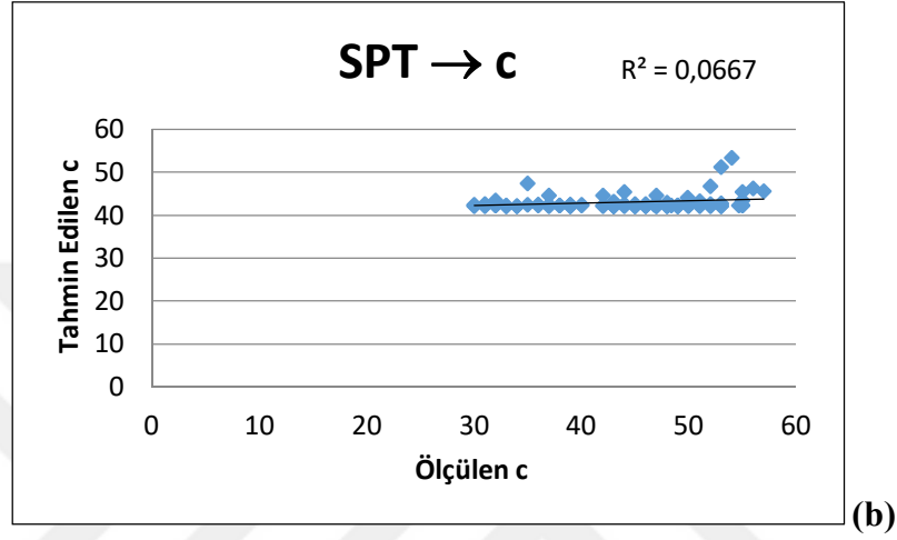
Şekil 5.3. (a) SPT değerine göre c değerini tahminleyen YSA modelinin şematik gösterimi. (b) YSA modelinin verdiği sonuç.
