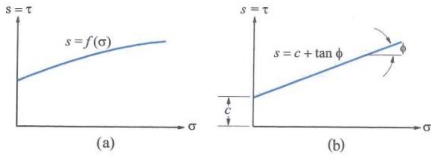
Şekil 2.20. Zeminlerde kayma direnci a) Mohr b) Mohr-Coulomb
