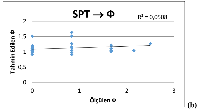
Şekil 5.4. (a) SPT değerine göre \Phi değerini tahminleyen YSA modelinin şematik gösterimi. (b) YSA modelinin verdiği sonuç.
