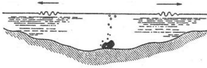
Şekil 2.6. Gölde bir taş atma neticesinde oluşan dalgacıklar [30].
