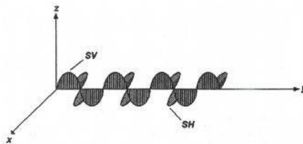
Şekil 2.3. SH ve SV dalga yayınımları [28].
