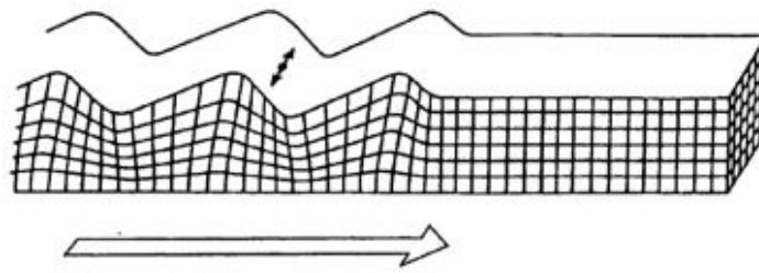
Şekil 2.5. Love dalgası hareketi [27].
