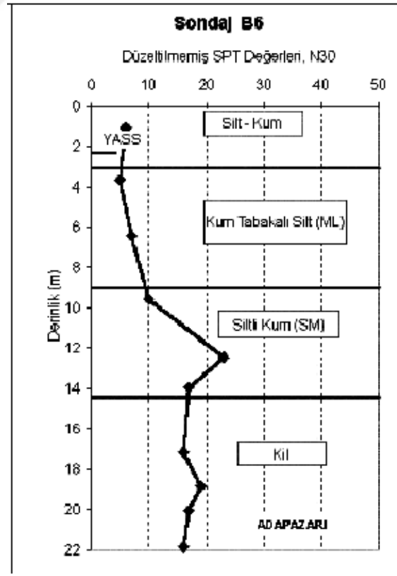
Şekil 3.6. Adapazarı'nda ağır hasar alan bölgeden zemin kesidi (B6) [66]
