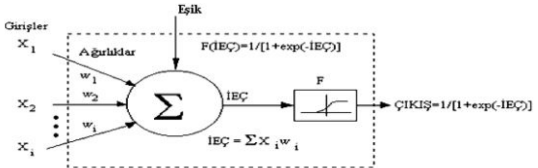
Şekil 4.2. Bir nöronun YSA modeli (İEÇ; İşlem Elemanının Çıkışı)
