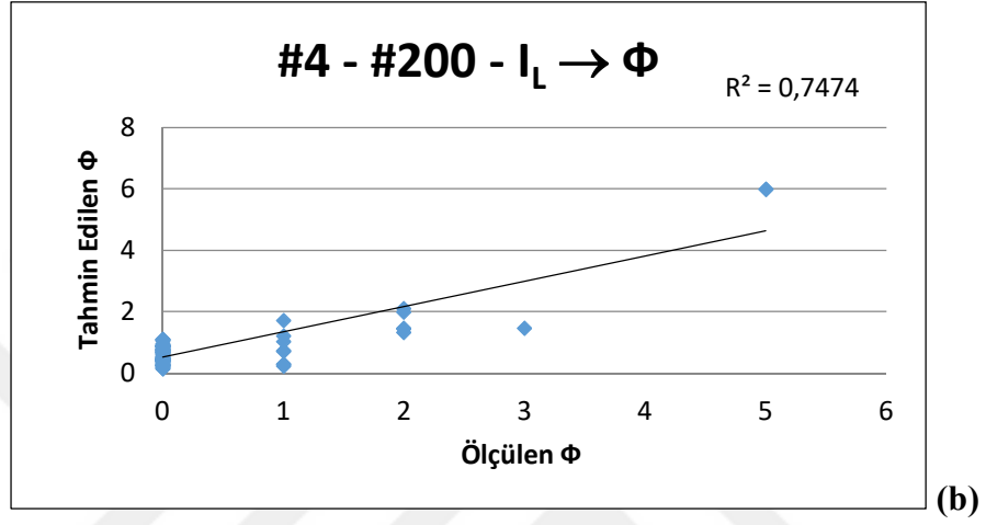
Şekil 5.19. (a) #4, #200 ve I_L değerine göre \Phi değerini tahminleyen YSA modelinin şematik gösterimi. (b) YSA modelinin verdiği sonuç.
