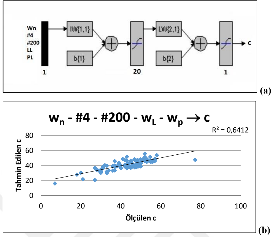
Şekil 5.25. (a) w_n , #4, #200, w_L ve w_p değerine göre c değerini tahminleyen YSA modelinin şematik gösterimi. (b) YSA modelinin verdiği sonuç.
