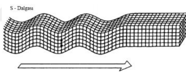
Şekil 2.2. S dalgası hareketi [27].
