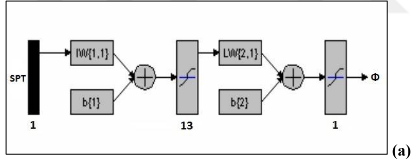
Şekil 5.3. (a) SPT değerine göre c değerini tahminleyen YSA modelinin şematik gösterimi. (b) YSA modelinin verdiği sonuç.
