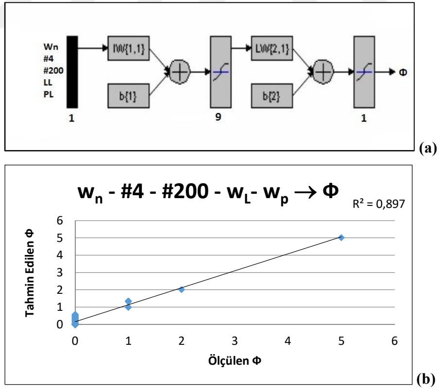
Şekil 5.26. (a) w_n , #4, #200, w_L ve w_p değerine göre \Phi değerini tahminleyen YSA modelinin şematik gösterimi. (b) YSA modelinin verdiği sonuç.
