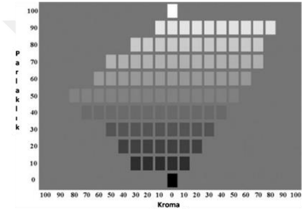
Şekil 3.6. Kroma ( C^* ) ve parlaklık ( L^* ) ilişkisi
