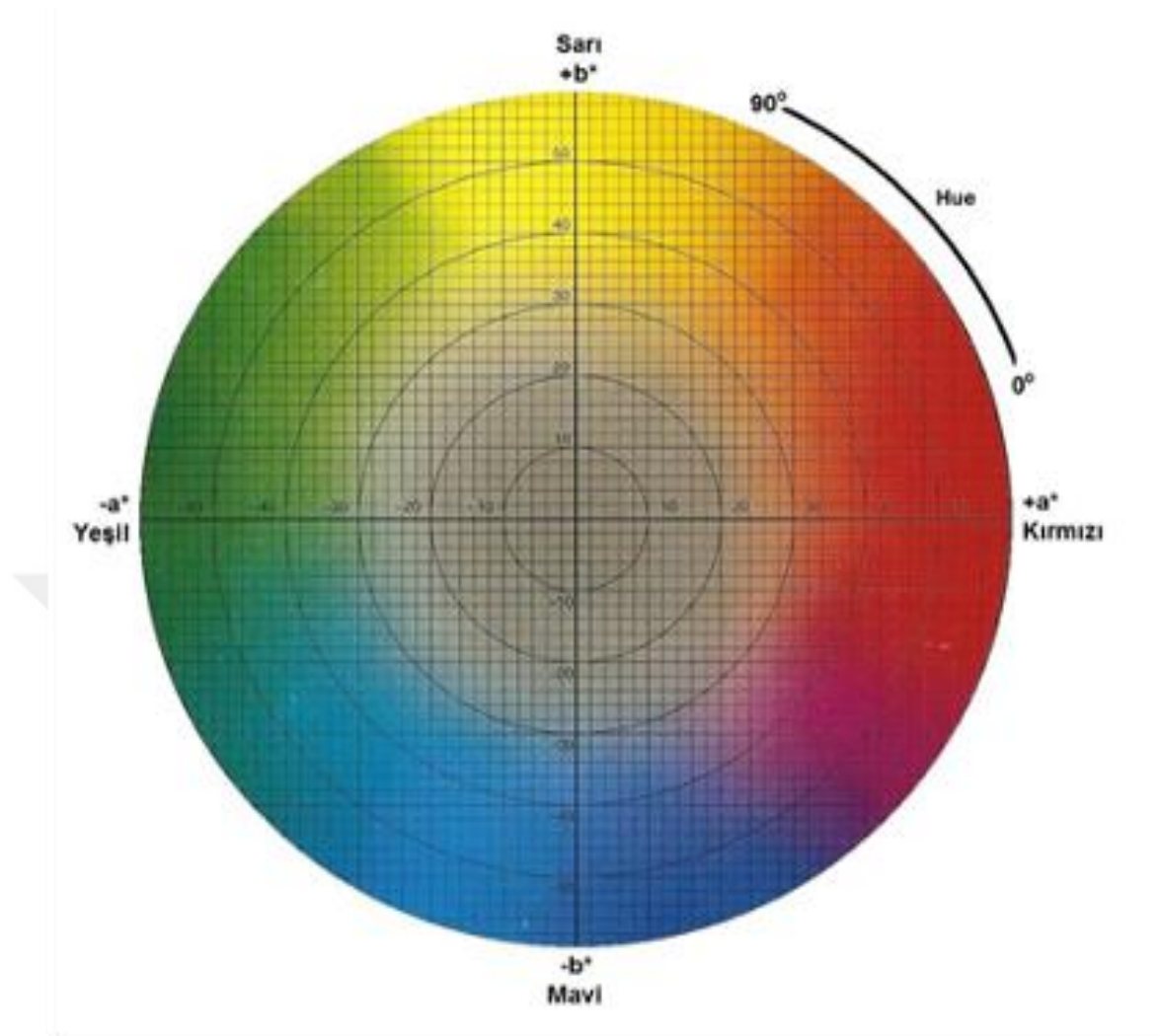
Şekil 3.7. Renk çizelgesinde a^* ve b^* değerlerinin karşılık geldiği renkler
