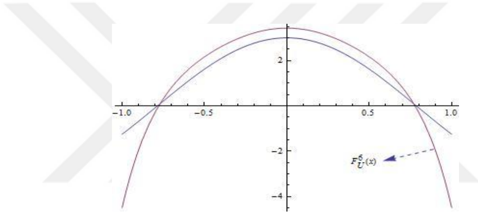
Şekil 4.2. f(x) = 3\cos(2x) ve F_U^6(x) in grafiği
