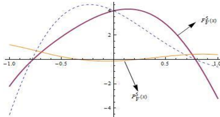
Şekil 4.11. f(x) = 4e^{-x} \cos(2x) , F_V^5(x) ve P_V^5(x) in grafiği
