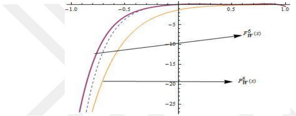
Şekil 4.8. F_w^6(x) ve P_w^6(x) in grafiği
