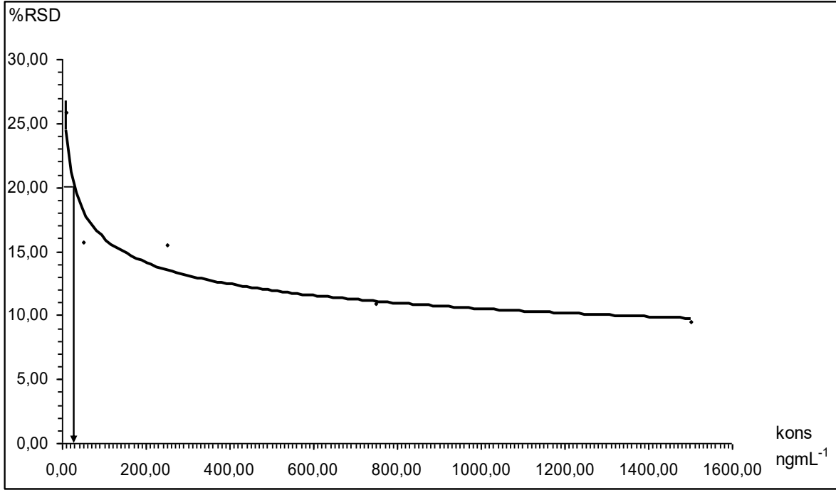
Şekil 113. Ciğer matrigsine ekstraksiyon öncesi 10,00, 50,00, 250,00, 750,00, 1500,00, 3000,00 ve 5000,00 ng mL -1 amitriptilin standart çözeltileri katılması (EÖAK) ile bulunan pik alanları yardımıyla Eurochem tarafından tavsiye edilen yönteme göre LOQ değerin bulunması için katılan amitriptilin konsantrasyonlarına karşı çizilen % RSD grafiğı (LOQ=25,00 ngmL -1 )
