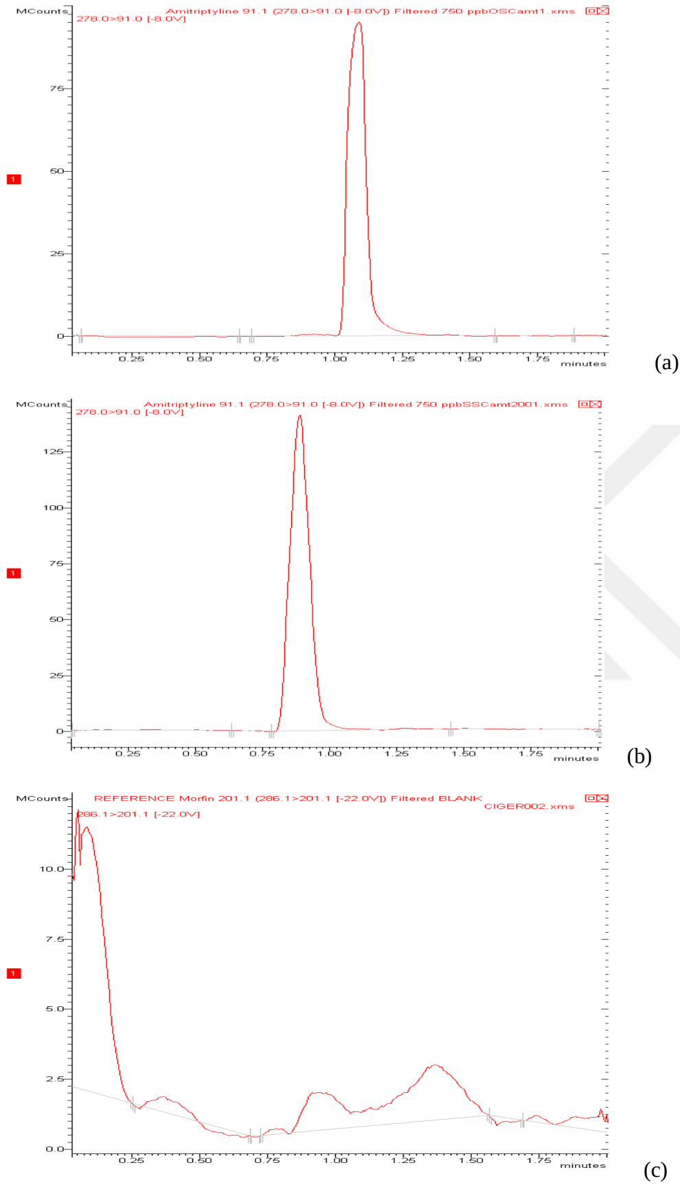
Şekil 111: Ekstraksiyon öncesi (a) ve ekstraksiyon sonrası katım yapılmış olan, 750,00 \text{ ngmL}^{-1}
