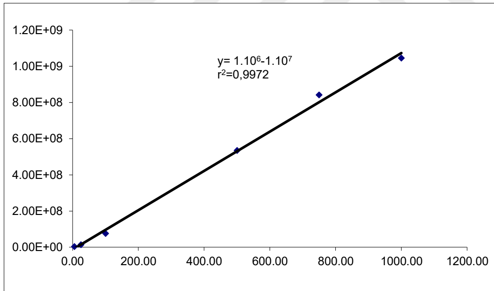
Şekil 107: 5,00, 25,00, 100,00, 500,00, 750,00 ve 1000,00 ngmL -1 morfin standart çözeltileri kullanılarak, larvadan ekstraksiyon çalışması öncesinde çizilen kalibrasyon grafiği
