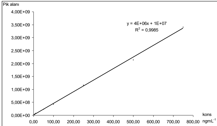
Şekil 109: 5,00, 10,00, 50,00, 100,00, 250,00, 500,00 ve 750,00 ngmL -1 amitriptilin standart çözeltileri kullanılarak, ekstraksiyon çalışmaları öncesinde çizilen kalibrasyon grafiği
