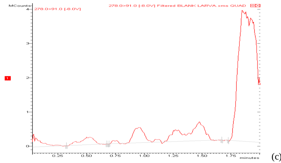
Şekil117: Ekstraksiyon öncesi (a) ve ekstraksiyon sonrası katım yapılmış olan, 500,00 \text{ ngmL}^{-1} konsantrasyondaki amitriptillin larva ekstraktları (b) ve blank larva kromatogramı (c).
