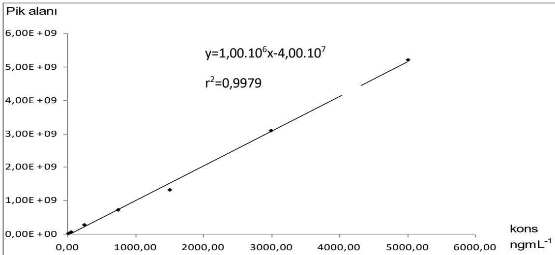
Şekil 116: Ciğer matriksine ekstraksiyon sonrası 10,00, 50,00, 250,00, 750,00, 1500,00, 3000,00 ve 5000,00 ngmL -1 amitriptilin standart çözeltilerinin katılması (ESAK) ile amitriptilin tayin yöntemi için oluşturulmuş olan kalibrasyon grafiği (LOQ: 10,00 ngmL -1 )
