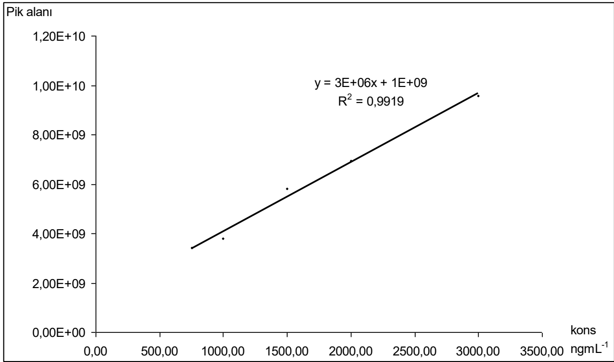
Şekil 110: 750,00, 1000,00, 1500,00, 2000,00, 3000,00 ngmL -1 amitriptillin standart çözeltiler kullanılarak, ekstraksiyon çalışmaları öncesinde çizilen kalibrasyon grafiği
