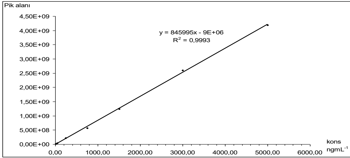
Şekil 115: Ciğer matrigksine ekstraksiyon öncesi 10,00, 50,00, 250,00, 750,00, 1500,00, 3000,00 ve 5000,00 ng mL -1 konsantrasyonlarda amitriptilin katılması (EÖAK) ile amitriptilin tayin yöntemi için oluşturulmuş olan kalibrasyon grafiğidir (LOQ: 25,00 ng mL -1 )
