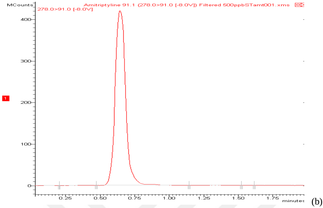
Şekil 108: Metanol çözücüsüne ilişkin amitriptillin kanalında gözlenen kromatogram (a), ciğerden ekstraksiyon çalışması öncesinde hazırlanmış olan, 500,0 ngmL -1 amitriptillin standart çözeltisinde gerçekleştirilen analiz sonucu gözlenen amitriptillin piki (b)
