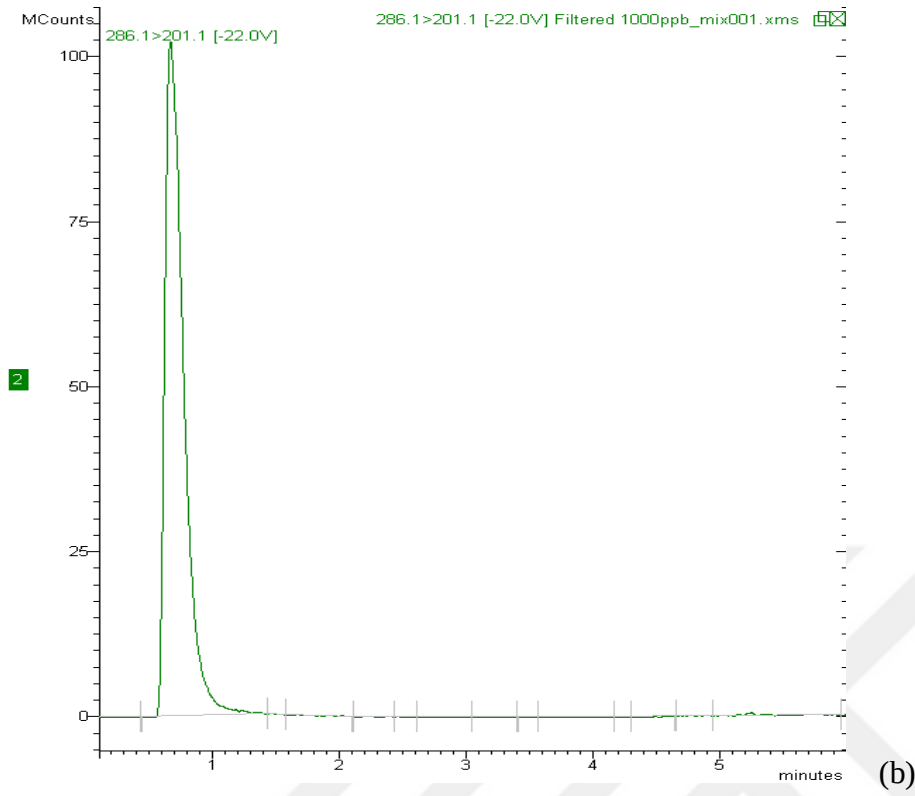
Şekil 105: Metanol çözücüsüne ilişkin morfin kanalında gözlenen kromatogram (a), 1000,0 ngmL -1 konsantrasyonda morfin içeren metanolde gerçekleştirilen analiz sonucu gözlenen morfin piki (b)
