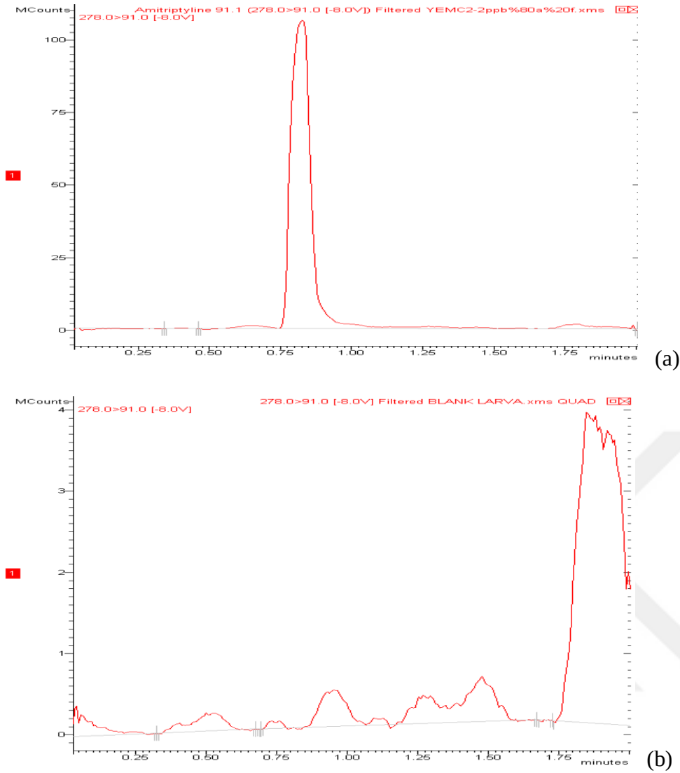
Şekil 118: 250,00 g çiğereC2=750000,00 ng amitriptillin katılmış olan ciğerden yemiş larva ekstraktının (a) ve larva blank ekstraktın kromatogramı (b).
