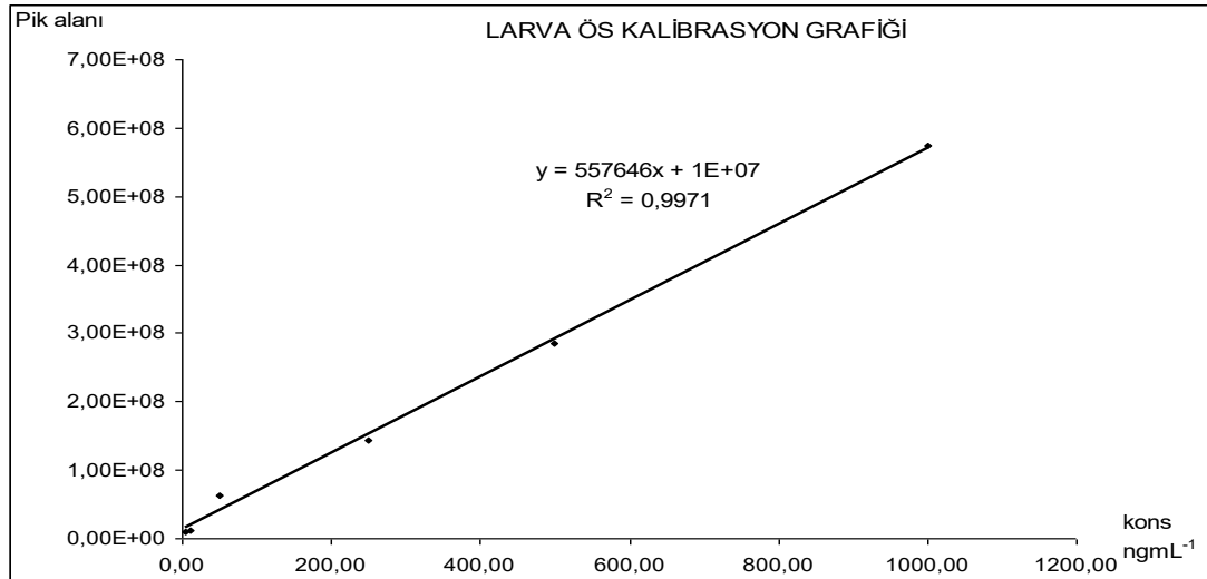
Şekil 201: Larva matriksine ekstraksiyon öncesi 5,00, 10,00, 50,00, 250,00, 500,00 ve 1000,00 ngmL -1 amitriptillin katılması (ESAK) ile amitriptillin tayin yöntemi için oluşturulmuş olan kalibrasyon grafiği (LOQ: 7,00 ngml -1 )
