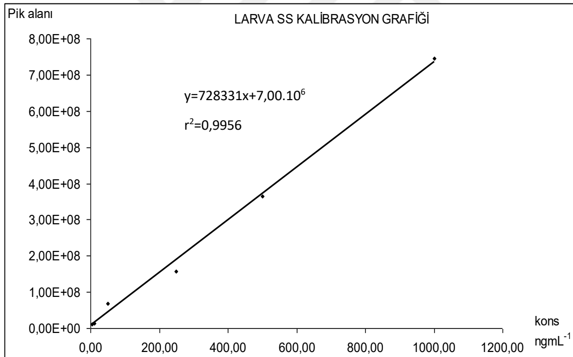
Şekil 202: Larva matrisine ekstraksiyon sonrası 5,00, 10,00, 50,00, 250,00, 500,00 ve 1000,00 ngmL -1 amitriptilin katılması (ESAK) ile amitriptilin tayin yöntemi için oluşturulmuş olan kalibrasyon grafiği (LOQ: 6,00 ngmL -1 )
