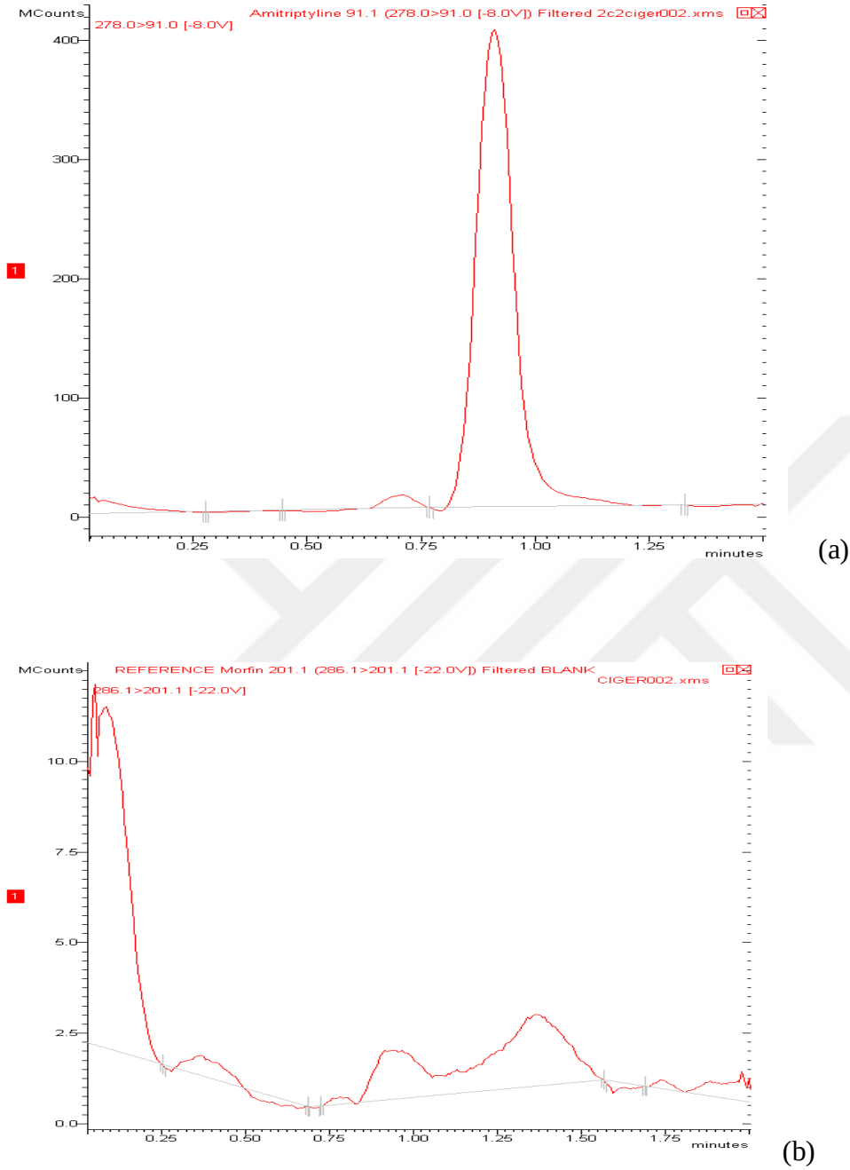
Şekil 112: C2 ngmL -1 konsantrasyondaki amitriptillin katılmış olan ve larvaların üzerinden yediği ciğerden alınan örneğin ekstraktının (a) ve blank ekstraktın kromatogramı (b).
