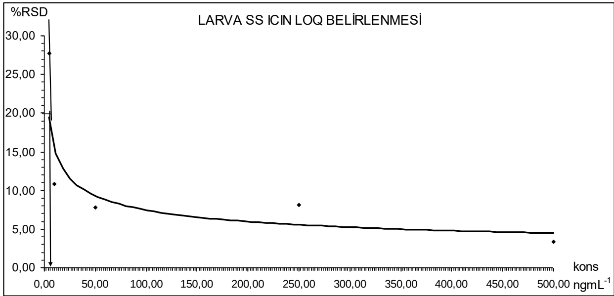
Şekil 200: Larva matriksine ekstraksiyon sonrası 5,00, 10,00, 50,00, 250,00 ve 500,00 ngmL -1 amitriptilin standart çözeltileri katılması (ESAK) ile bulunan pik alanları yardımıyla Eurachem tarafından tavsiye edilen yöntemle göre LOQ değerinin bulunması için katılan amitriptilin konsantrasyonlarına karşı çizilmiş olan %RSD grafiği (LOQ=6,00 ngmL -1 ) (Grafikte %20,00 RSD ye denk gelen konsantrasyon, LOQ değeri olarak alınmıştır.)
