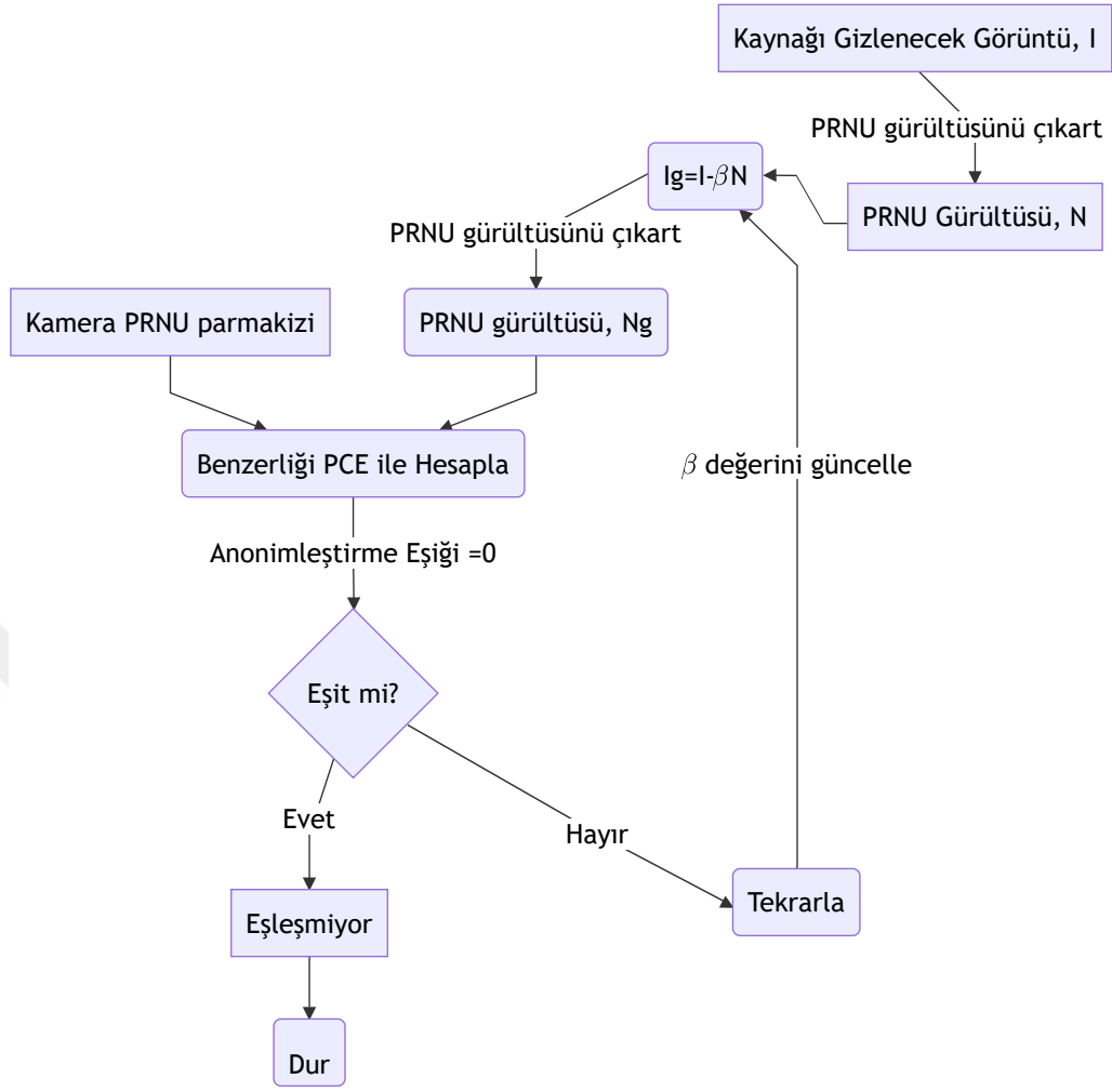
Şekil 3.2. Önerilen Yöntem Akış Diyagramı
