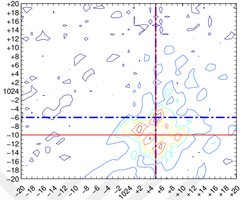
Şekil 4.18. Izgara tarama işlemi ile dönüşüme uğramış görüntü #3 için elde edilen PRNU benzerlik konturunun çizimi. Mavi çizgi ile kestirilen (\hat{x}'_1, \hat{y}'_1) , kırmızı çizgi ile uygulanan dönüşüme ilişkin gerçek ters dönüşüm parametresi (x'_1, y'_1) gösterilmektedir. Şeklin yatay eksenini görüntünün X eksenine, dikey eksenini ise Y eksenine tekabül etmektedir.
