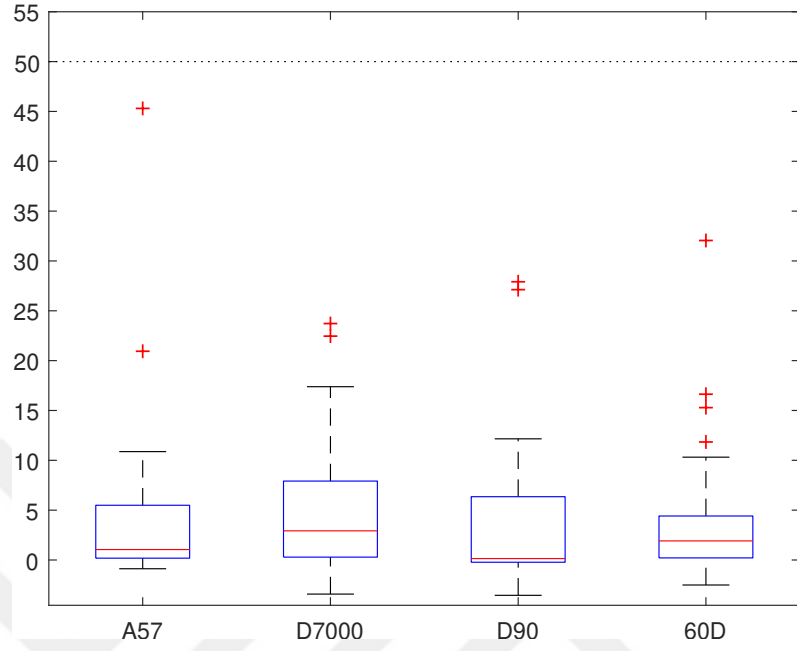
(a) Her bir kamera için PRNU benzerliğini gösteren PCE değeri dağılımları
