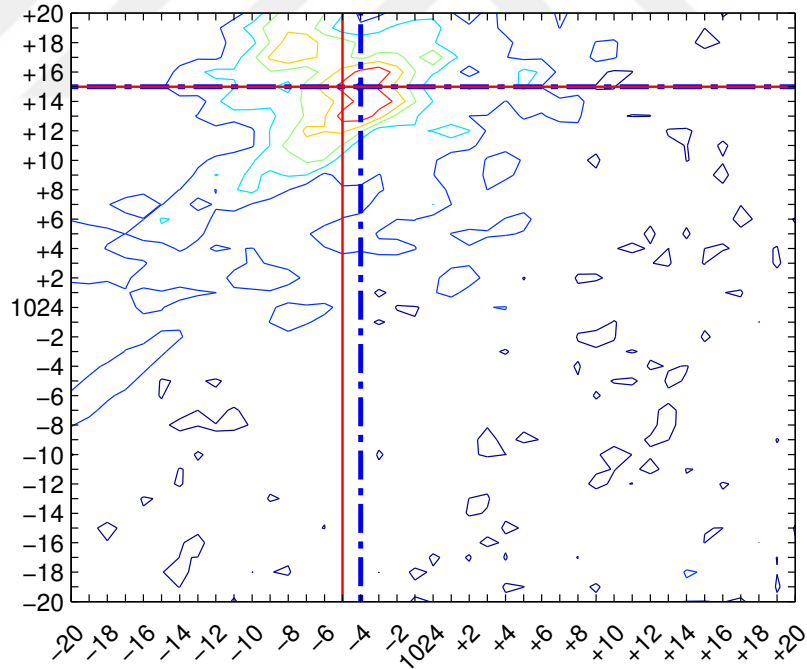
Şekil 4.16. ızgara tarama işlemi ile dönüşüme uğramış görüntü #1 için elde edilen PRNU benzerlik konturunun çizimi. Mavi çizgi ile kestirilen (\hat{x}'_1, \hat{y}'_1) , kırmızı çizgi ile uygulanan dönüşüme ilişkin gerçek ters dönüşüm parametresi (x_1, y_1) gösterilmektedir. Şeklin yatay eksenı görüntünün X eksenine, dikey eksenı ise Y eksenine tekabül etmektedir.
