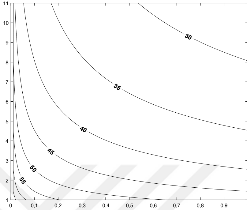
Şekil 3.1. Basitleştirilmiş görüntü kalitesi modeline göre, görüntü kalitesinin (PSNR [dB]), yatay ekseninde var(\Phi_2) (PRNU harici gürültülerin gücü) ve dikey ekseninde \beta (PRNU gürültü gücü katsayısı) değerlerine karşın değişimi. Konturlerdeki rakamlar PSNR seviyelerini göstermektedir. Şekile sığmayan kontur değerlerinden, en yüksek 65, sonraki 60 dB değerindedir. Örneğin \beta = 2 bulunduğunda, görüntünün diğer güçlerinin varyansı 0,1 ise, 50 ile 55 dB arasında bir PSNR seviyesine erişilebilir.
