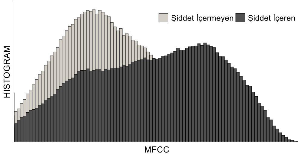
Şekil 5.2 Şiddet sahnesi sınıflandırması veri kümesinde MFCC özneliliğinin dağılımı
