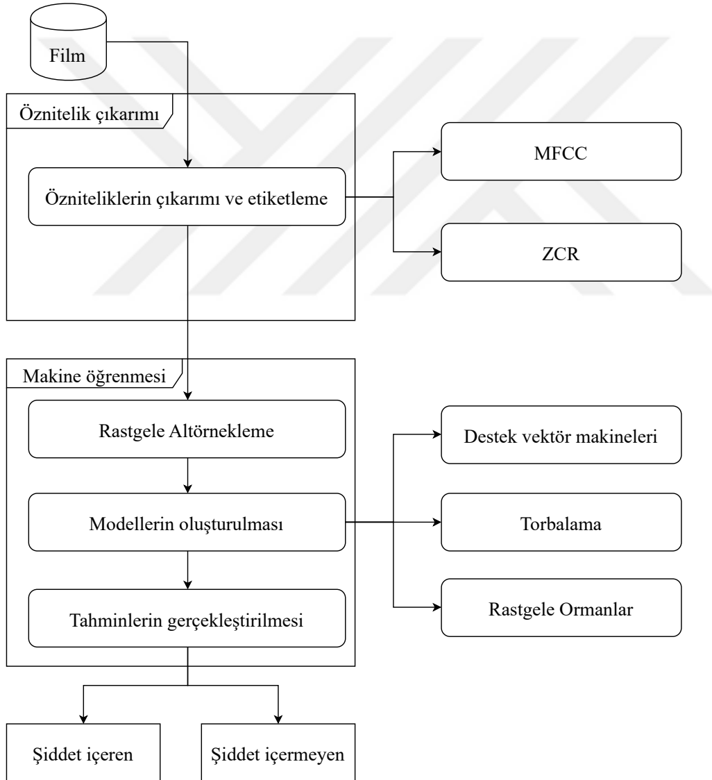
Şekil 5.1 Şiddet sahnesi sınıflandırma işleminin aşamaları
