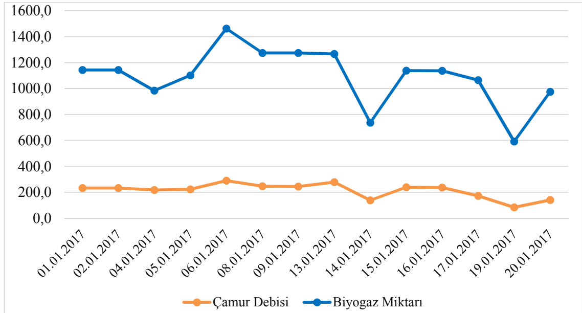
Şekil 6.5. Ocak ayı çamur debisi-biyogaz miktarı grafiği
