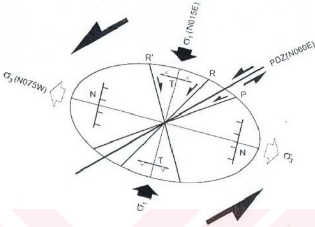
Şekil 4.18. Tarihîsel dönemde basit kayma deformasyonu süresince, Sivrice Fay Zonu'na (K60D) paralel olarak şekillenmiş yapılar arasındaki geometrik ilişkilerin görünümü. PDZ'ye göre Sintetik Riedel ve eşlenik antitetik makaslama kırıkları başlangıç açılarına göre sırasıyla \phi/2 ve 90^\circ - (\phi/2) 'dir. \phi açısı; içsel sürtünme açısı (teorik olarak 30^\circ ). \phi/2 açısı; PDZ'ye göre ikincil olarak gelişen sintetik kırık (P-kırığı). Gerilme (strain) elipsinin uzun eksenine paralel olarak gelişen ters fayların doğrultusu K075B olup ana yer değiştirme zonu ile 45^\circ 'lik açı yapmaktadır. Gerilme elipsinin kısa eksenine göre paralel olarak gelişen normal fayların doğrultusu ise K015D olup, ana yer değiştirme zonu 45^\circ 'lik açı yapmaktadır (Ramsay, 1967).
