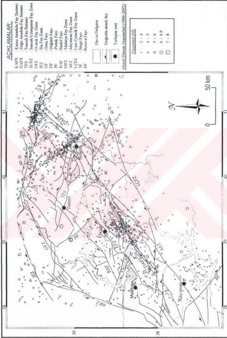
Şekil 4.24. İnceleme alanı ve yakın çevresinde alelcel dönemde meydana gelen depremler. (Veriler ISC ve Türknet kataloglarından alınmıştır).
