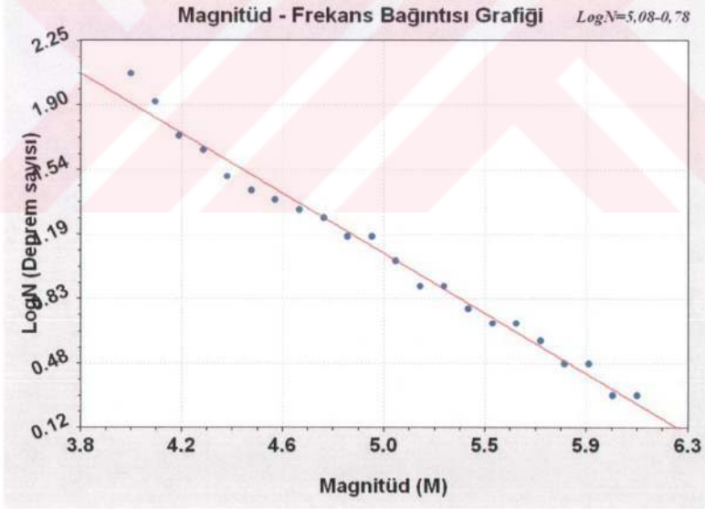
Şekil 4.27. Zaman magnitüdü değerleri için hesaplanan Magnitüd – Frekans grafiği.
