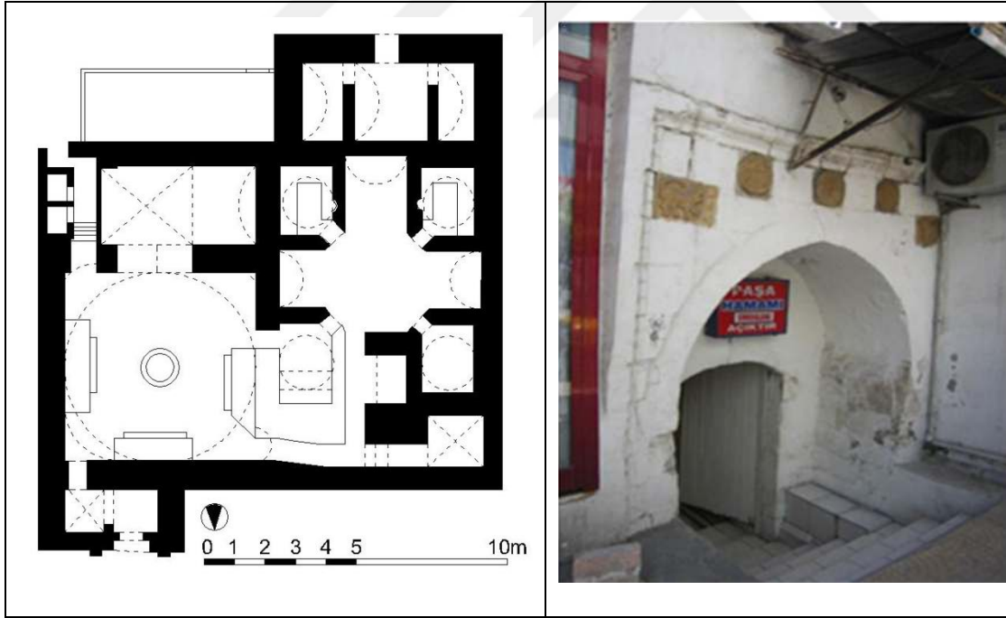
Şekil 4.19. Adıyaman Paşa (Kap) Hamamı planı (Bayhan ve Salman 2010) ve hamam girişi
