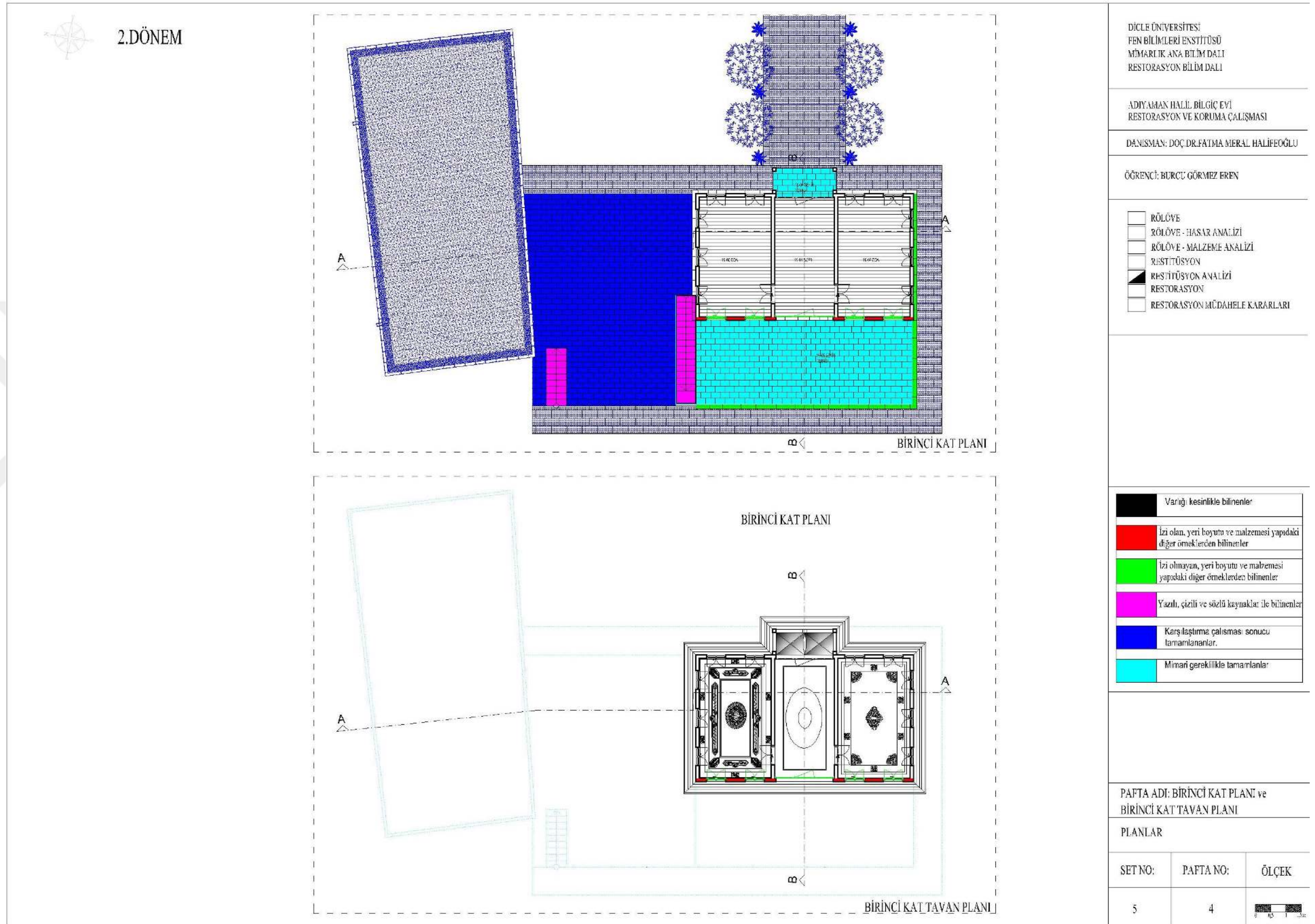
Şekil 4.140. Planlar ( a: Birinci kat planı; b: Birinci kat tavan planı)
