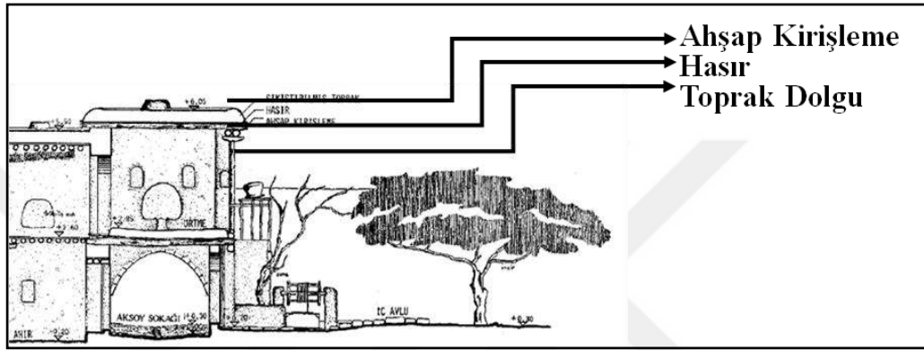
Şekil 4.47. Düz toprak dam katmanları (Erdim 1979)
