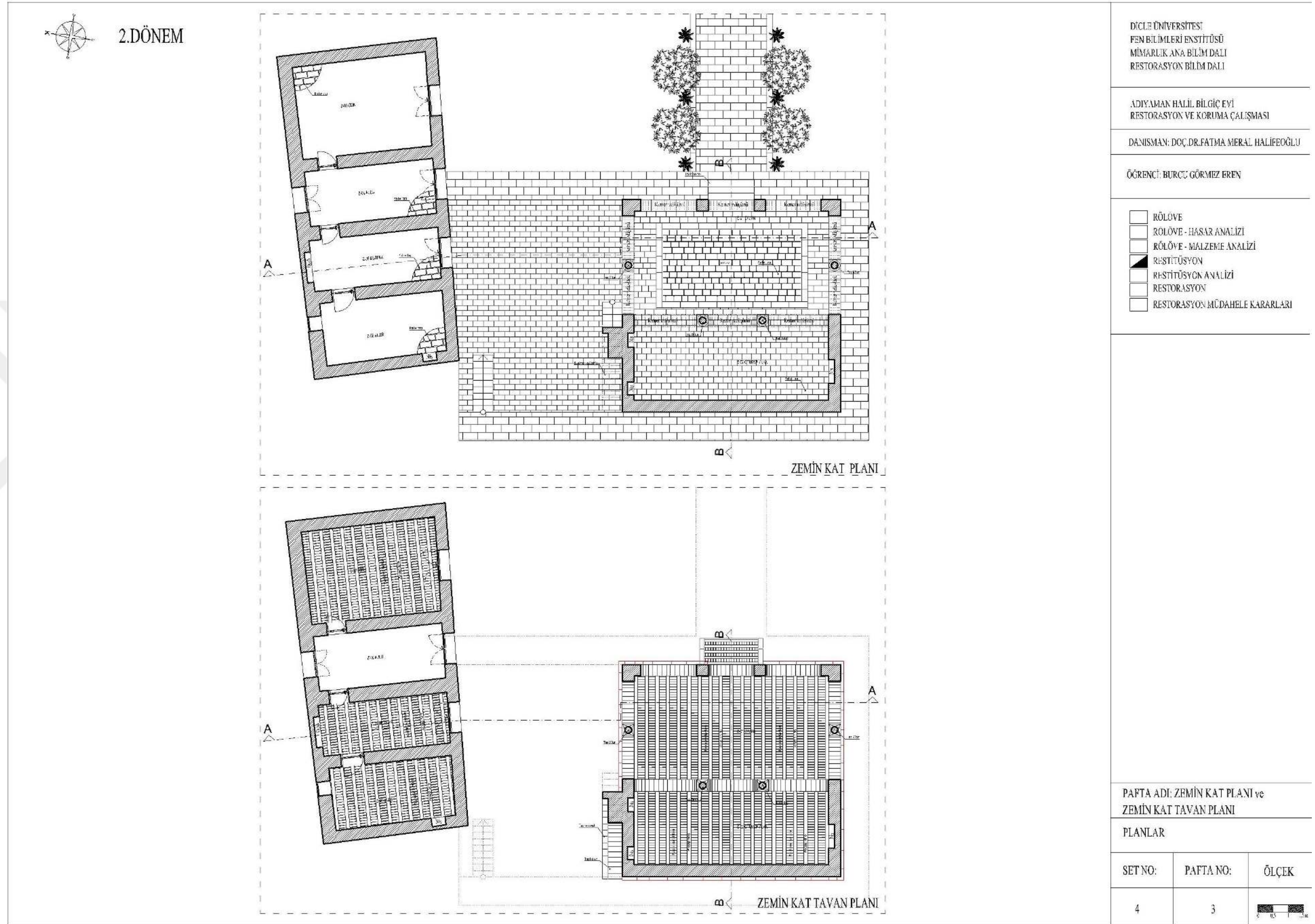
Şekil 4.133. Planlar ( a: Zemin kat planı; b: Zemin kat tavan planı)
