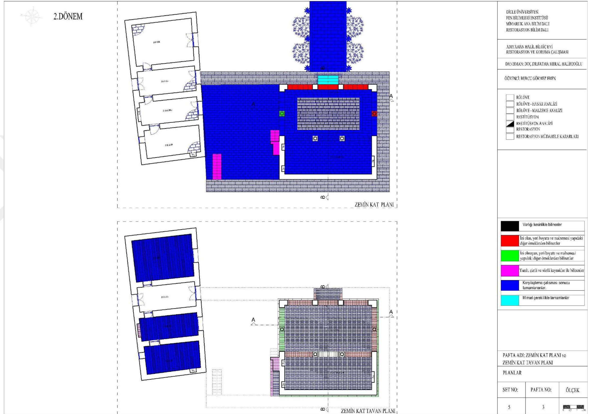
Şekil 4.139. Planlar ( a: Zemin kat planı; b: Zemin kat tavan planı)
