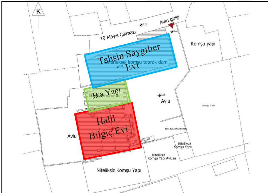
Şekil 4.57. Halil Bilgiç Evi vaziyet planı rölöve çizimi
