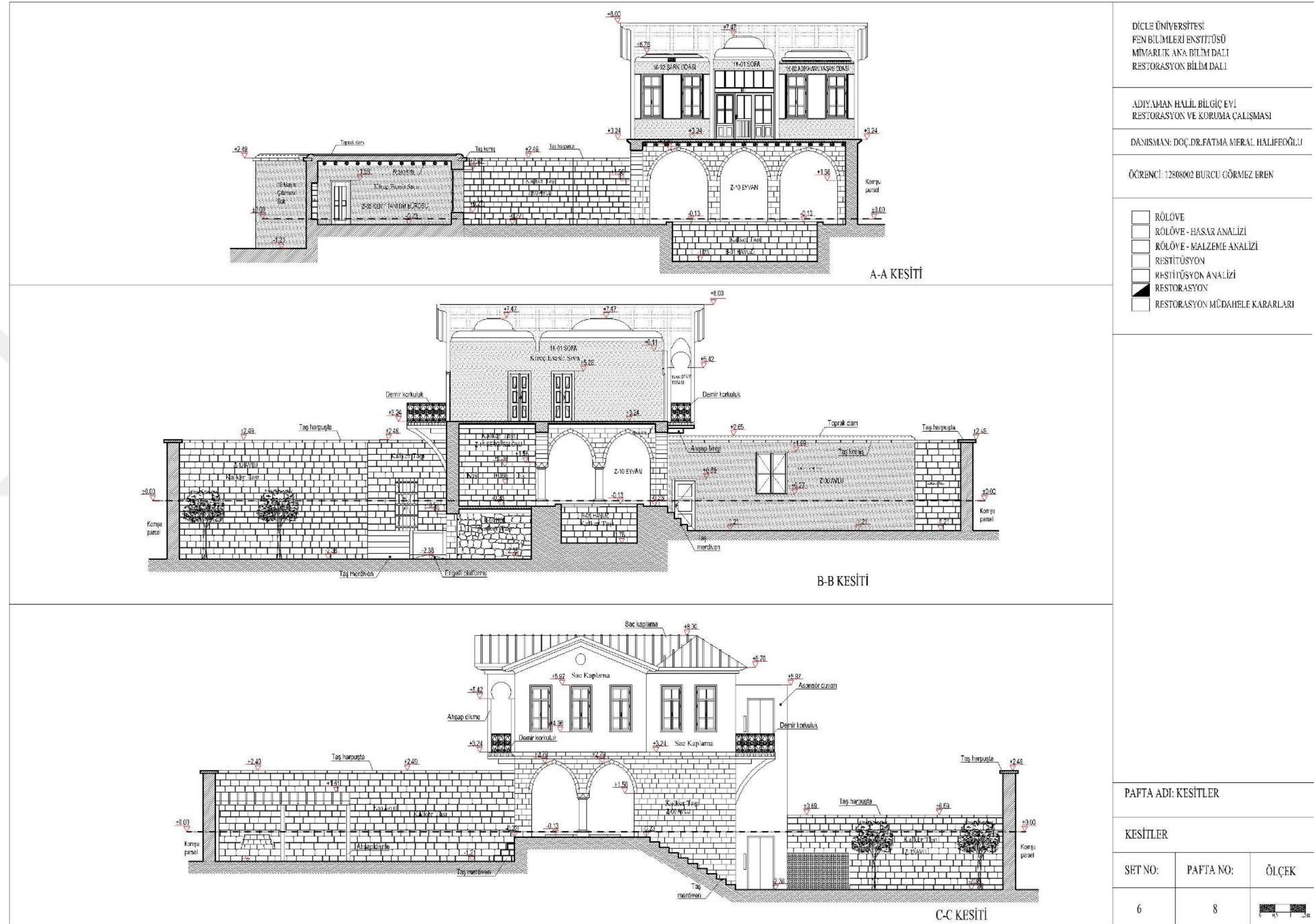
Şekil 4.154. Kesitler (a: Sokak cephesi; b: A-A kesiti; c: A-A kesiti)
