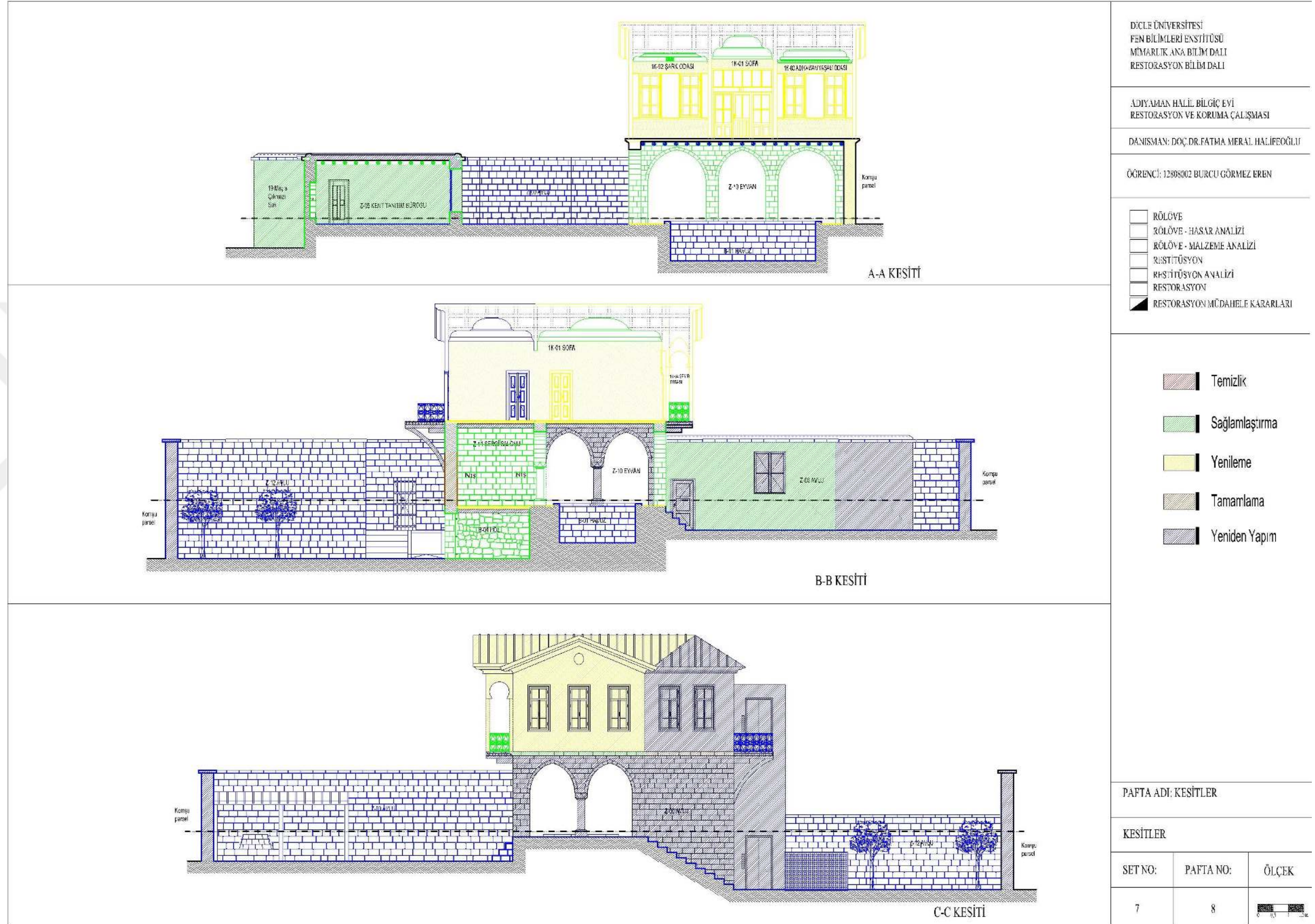
Şekil 4.163. Kesitler (a: A-A kesiti; b: B-B kesiti; c: C-C kesiti)
