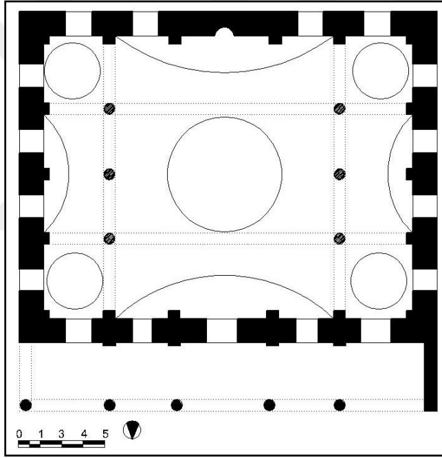
Şekil 4.13. Çarşı Camii planı (Bayhan ve Salman 2010)
