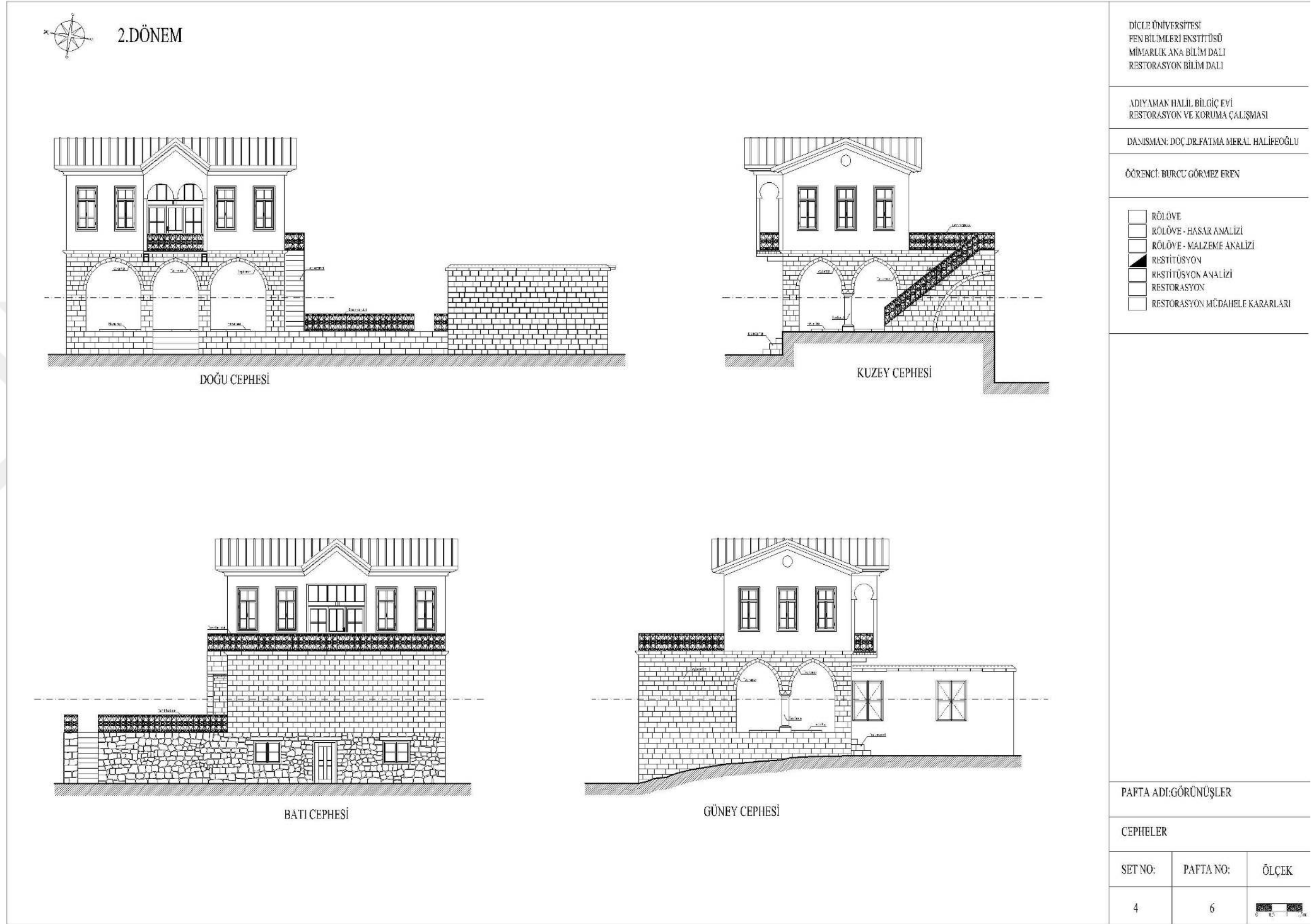
Şekil 4.136. Görünüşler ( a: Doğu cephesi; b: Kuzey cephesi; c: Batı cephesi; d: Güney cephesi )
