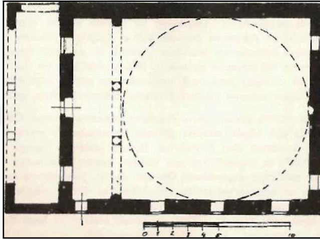
Şekil 4.11. Adıyaman Kap Camii Planı-(Erken 1983)
