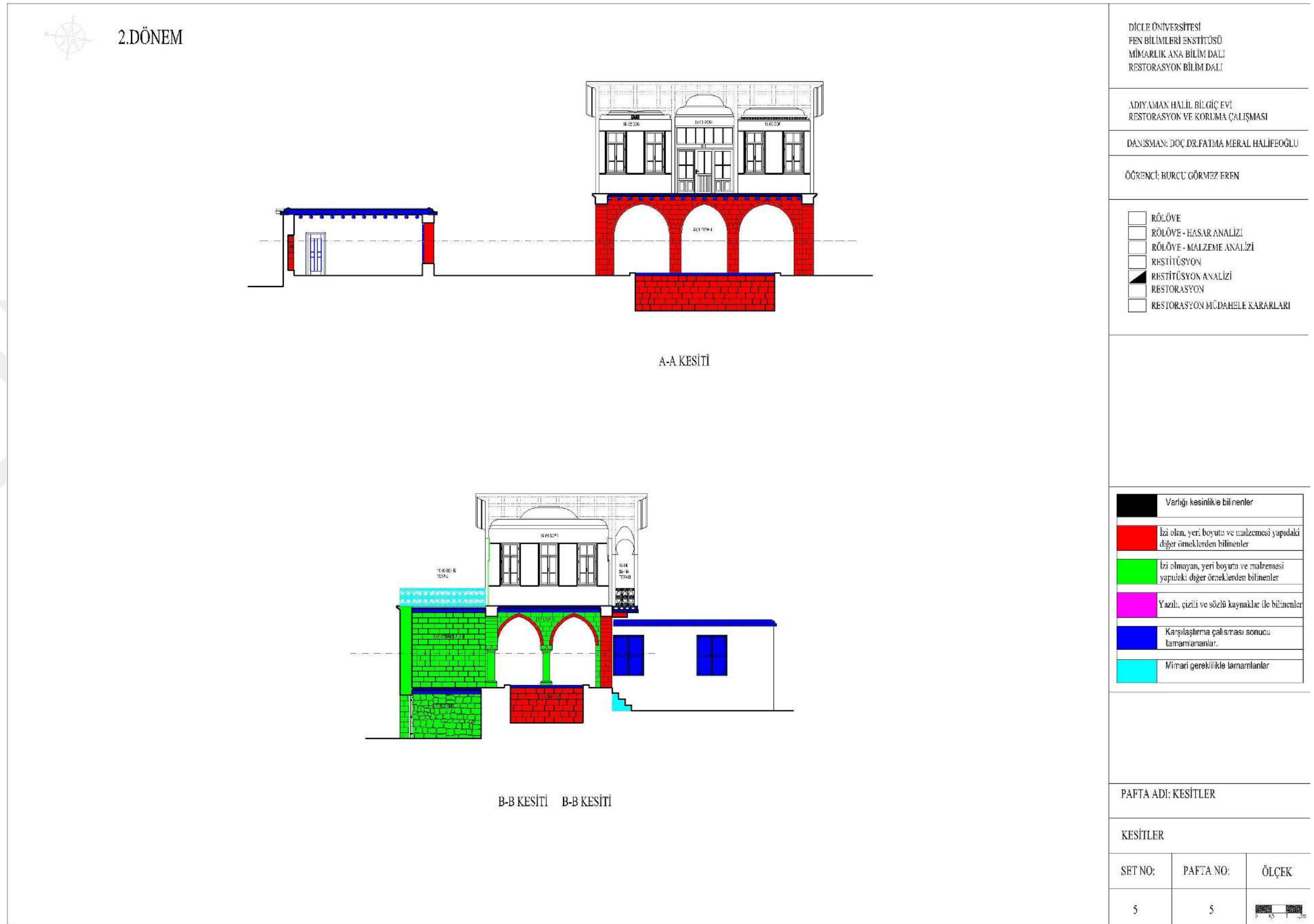
Şekil 4.141. Kesitler ( a: A-A kesiti; b: B-B kesiti)
