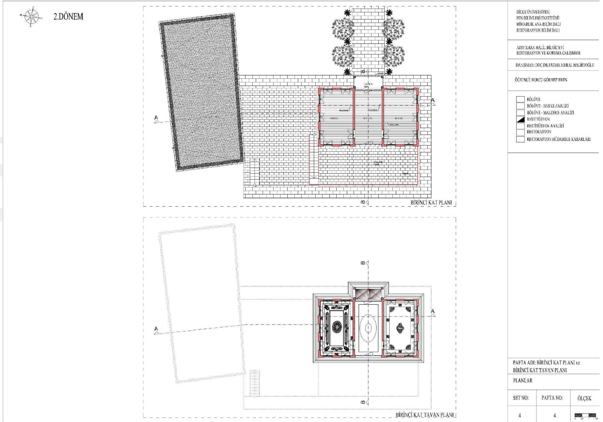
Şekil 4.134. Planlar ( a: Birinci kat planı; b: Birinci kat tavan planı)
