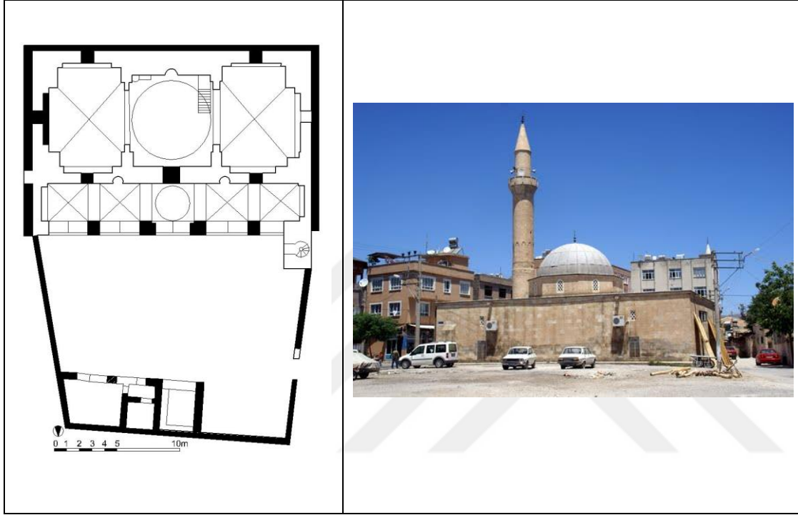
Şekil 4.16. Musalla Camii (2012) ve planı (Bayhan ve Salman 2010)
