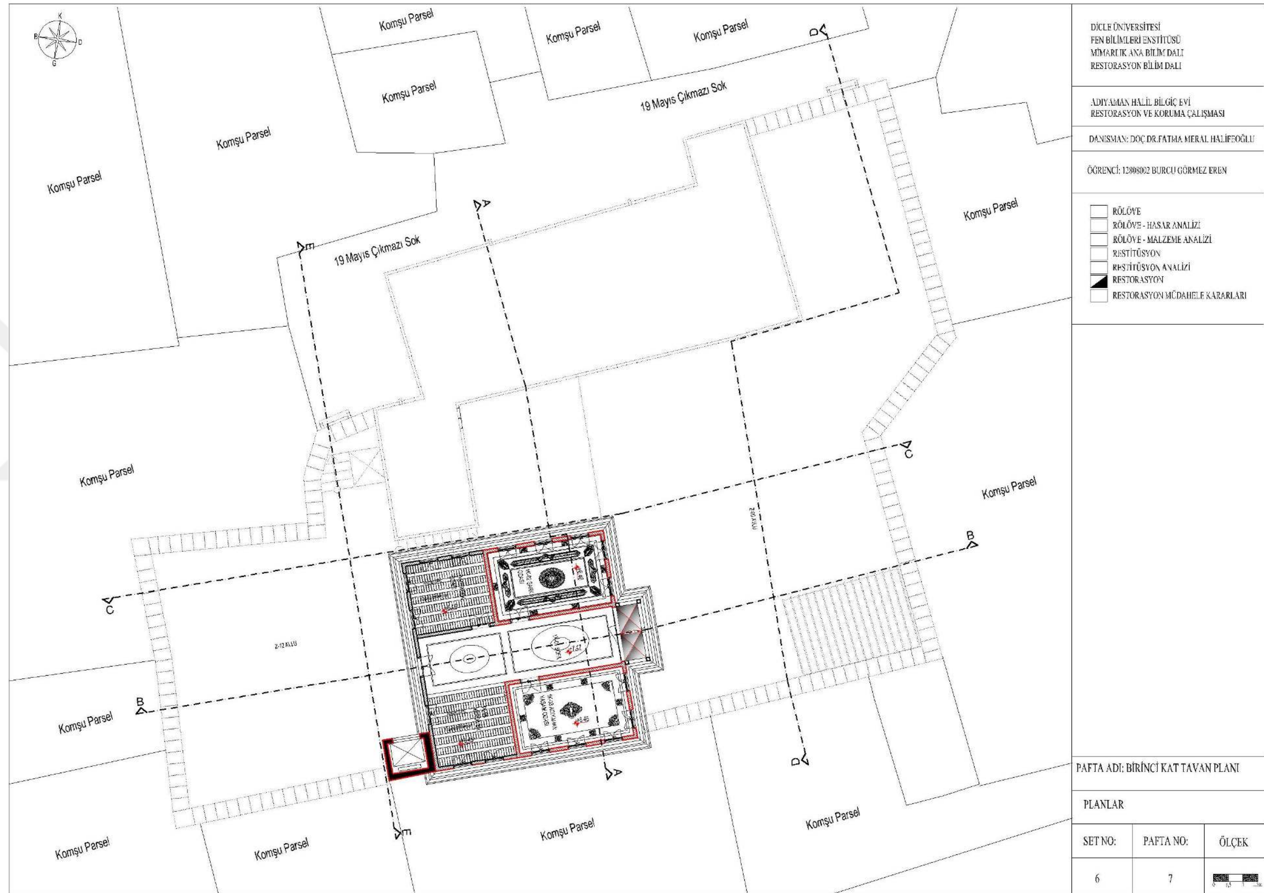
Şekil 4.153. Birinci kat tavan planı
