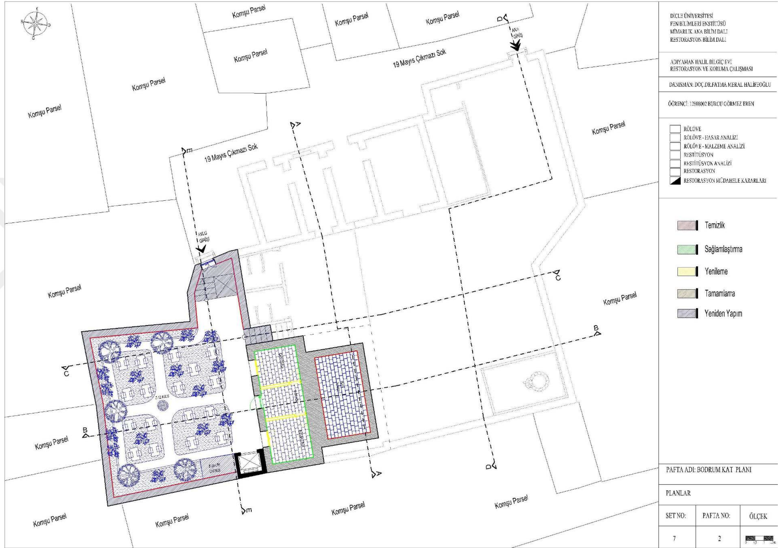
Şekil 4.157. Bodrum kat yakın çevre planı
