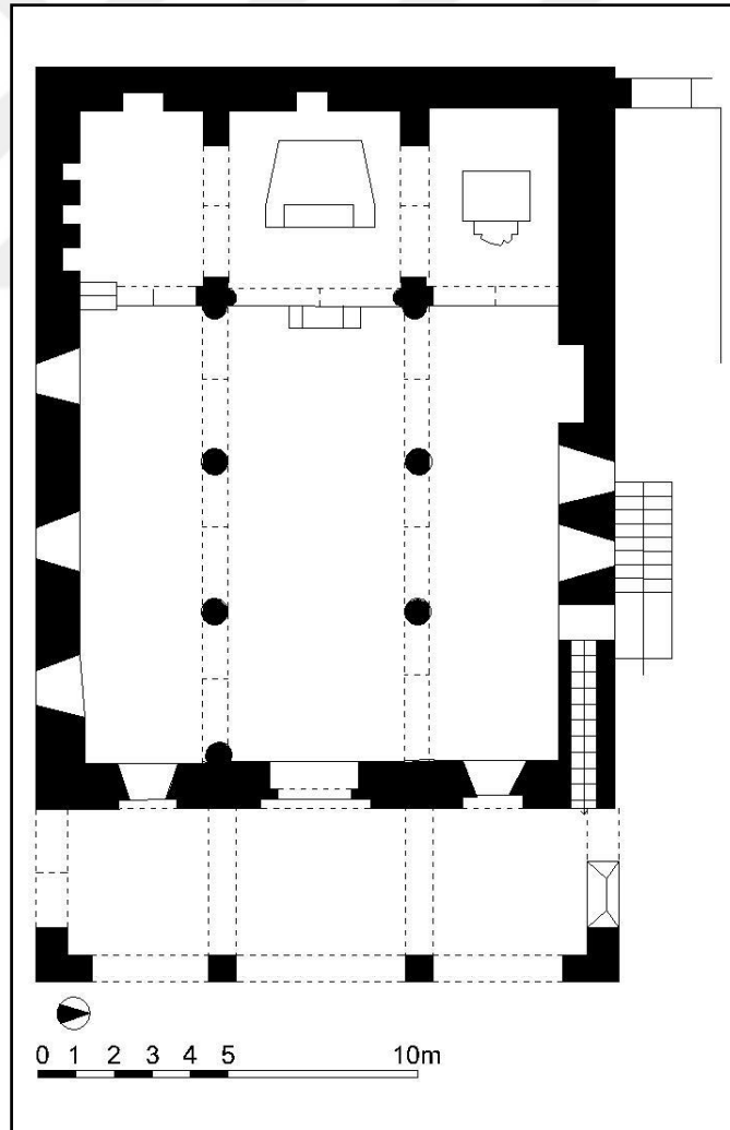
Şekil 4.18. Adıyaman St. Paul Kilisesi Planı (Bayhan ve Salman 2010)
