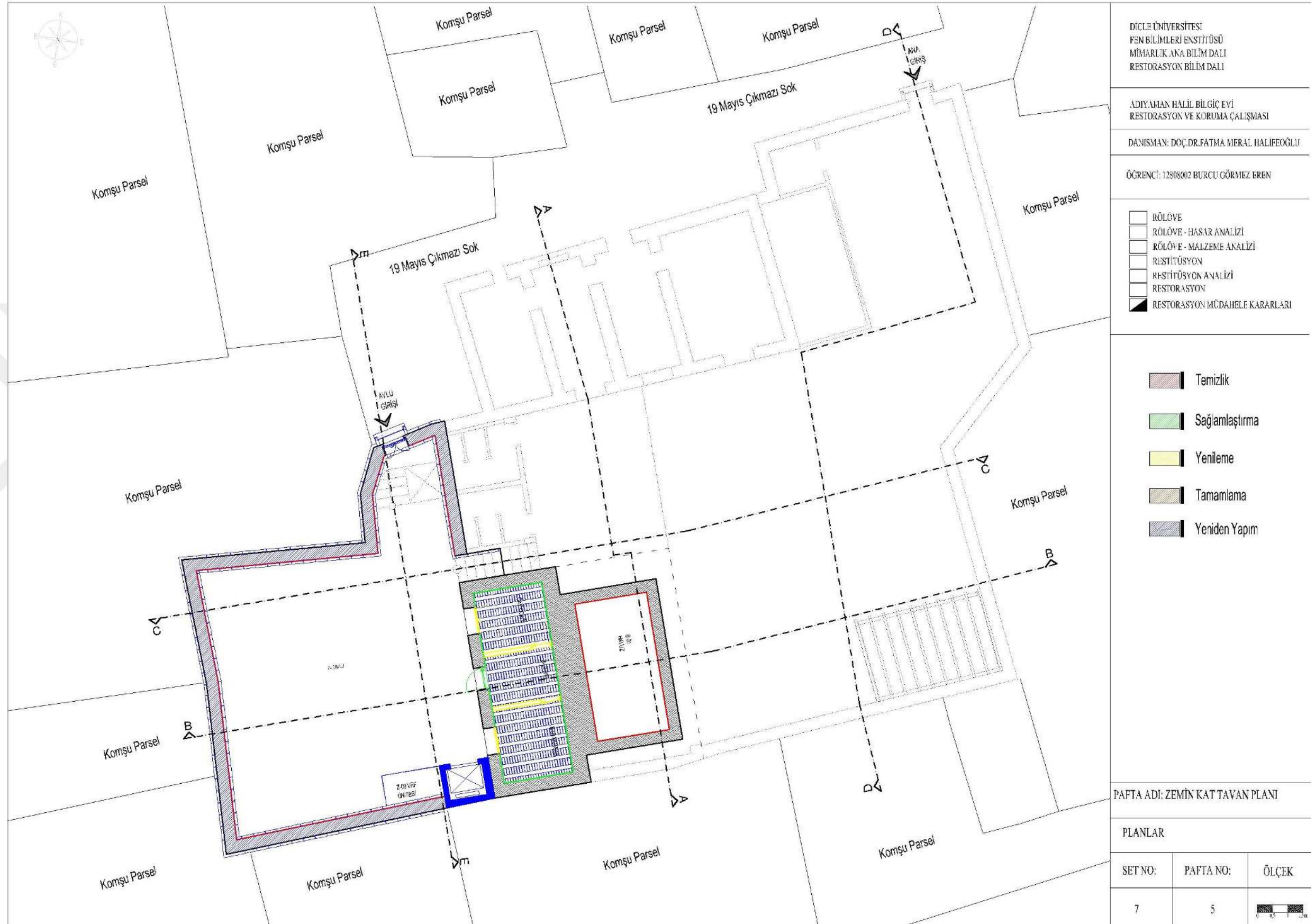
Şekil 4.160. Bodrum kat tavan planı
