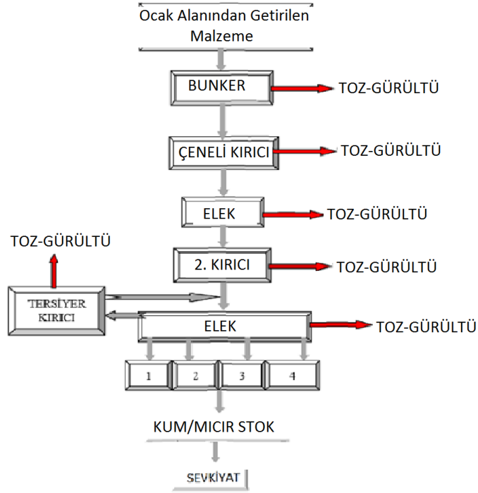
Şekil 1.3 Kum-çakıl kırma-eleme tesisi iş akım şeması
