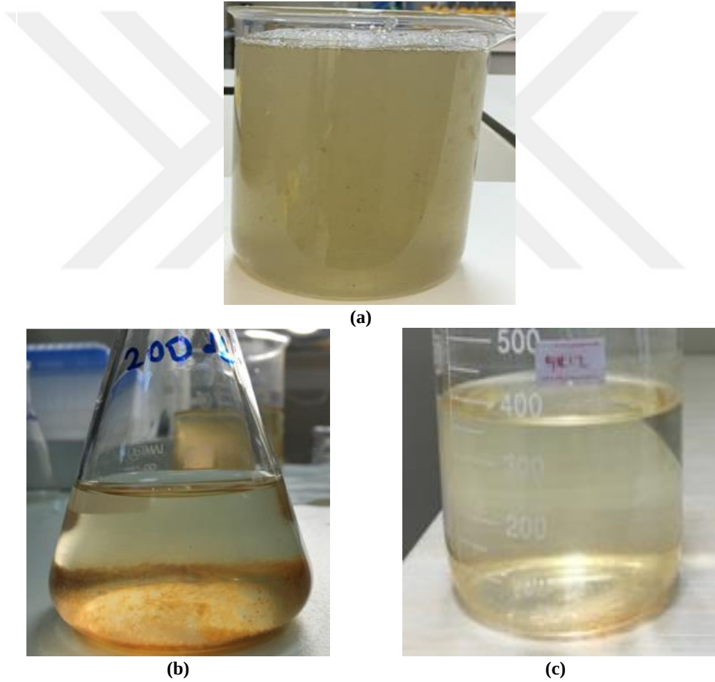
Şekil 3.3. Elektroflotasyon prosesi giriş atıksuyu ve arıtılmış çıkış suyundan görüntüler a) Kahta Yüzüncü Yıl Göletine deşarj edilen atıksu b) Çöktürme öncesi arıtılmış su c) Çöktürme sonrası arıtılmış su
