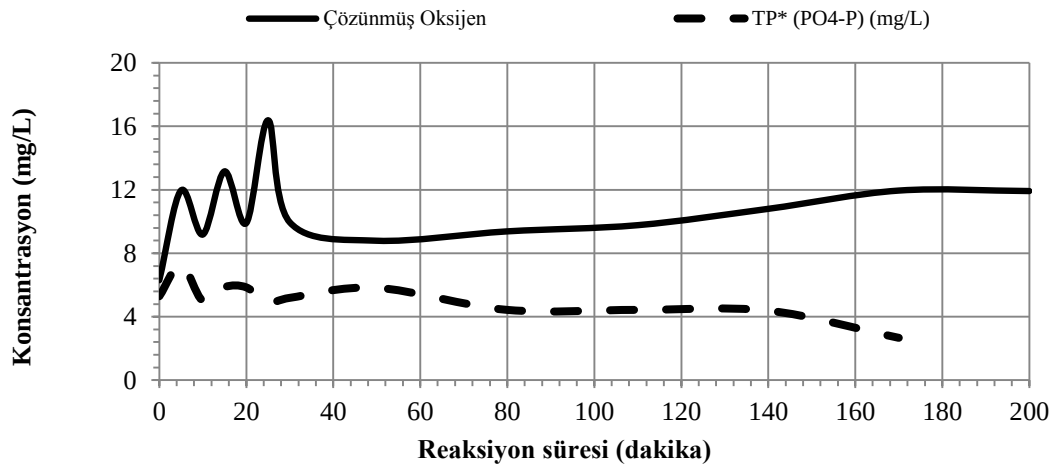
Şekil 3.14. EF sisteminde reaksiyon süresinde TP ve çözünmüş oksijen konsantrasyon değişimi
