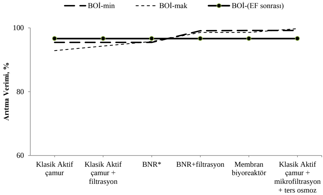
Şekil 3.17. BOİ 5 arıtma verimleri karşılaştırması
