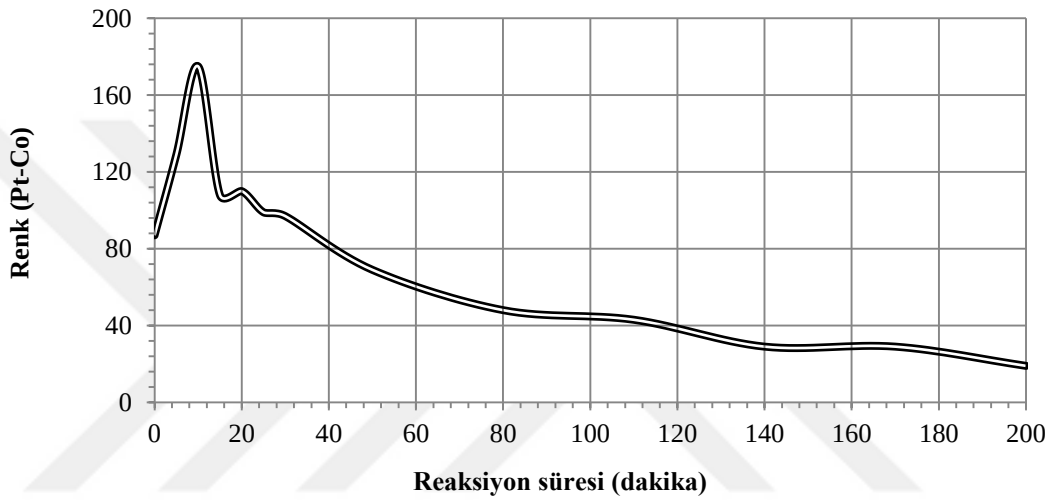
Şekil 3.6. EF sisteminde renk değişim konsantrasyonu
