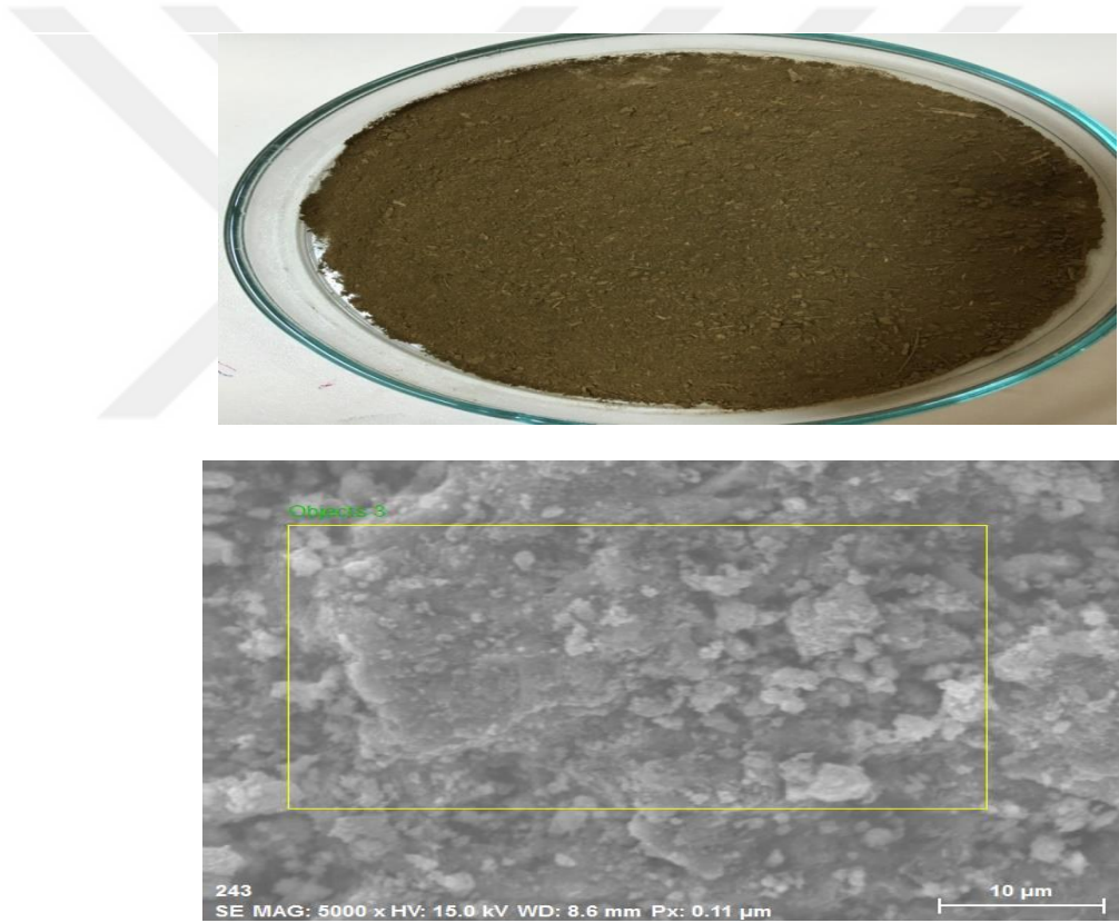
Şekil 3.24. Elektroflotasyon proses çıkış çamuru katı maddesinin SEM, EDX görüntüleri ve analizleri
