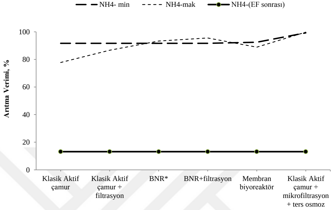
Şekil 3.19. \text{NH}_4 arıtma verimleri karşılaştırması
