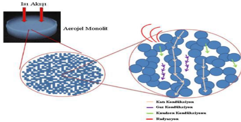
Şekil 3.15. Aerojel ısı transfer mekanizması
