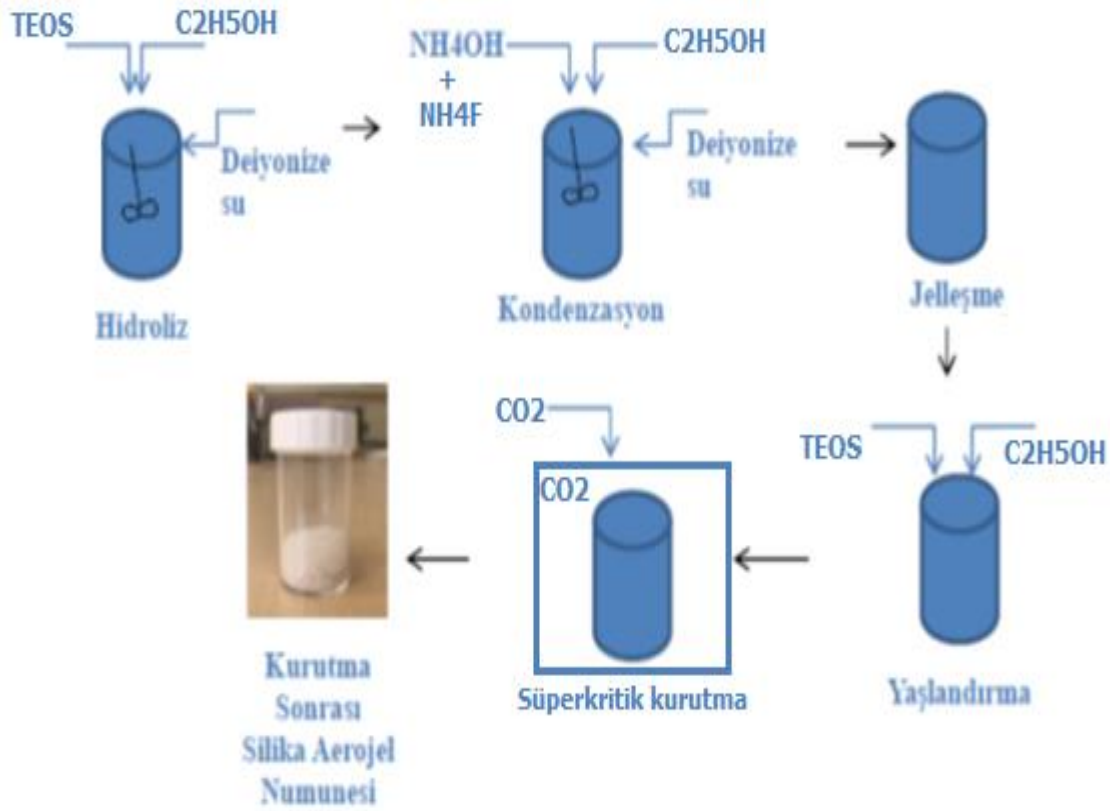
Şekil 3.21. TEOS silika aerojel sentezi deneysel prosedür
