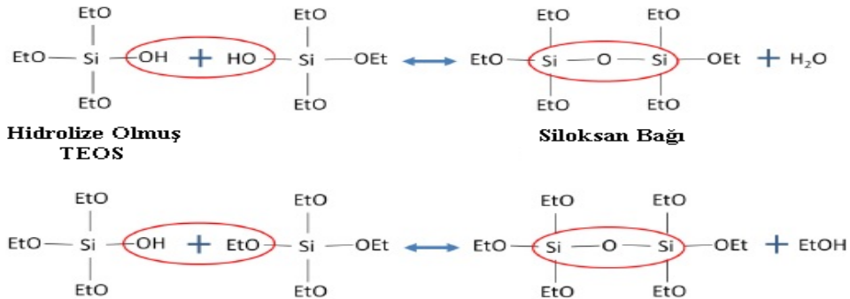
Şekil 3.7. TEOS’un hidroliz ve kondenzasyon tepkimeleri (Malay ve vd. 2013).
