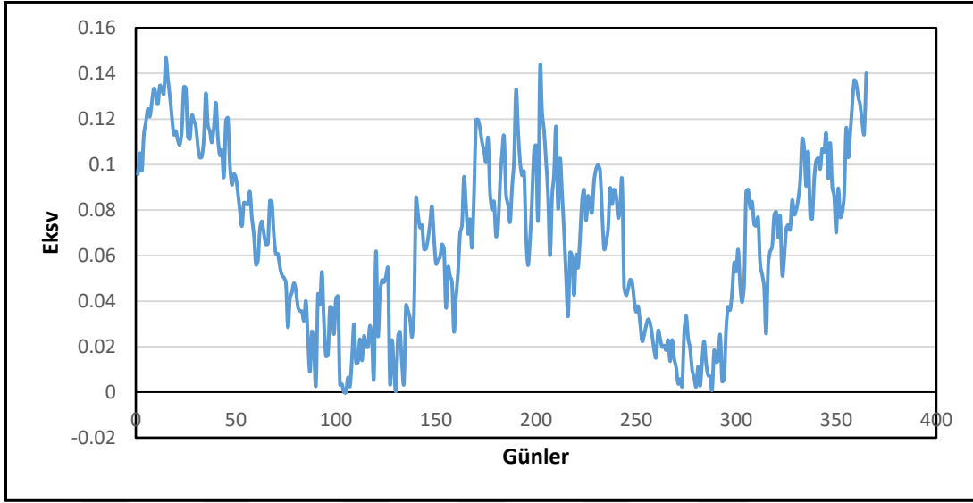
Şekil 6.10. Kandahar Şehrine ait ekserji verimi
