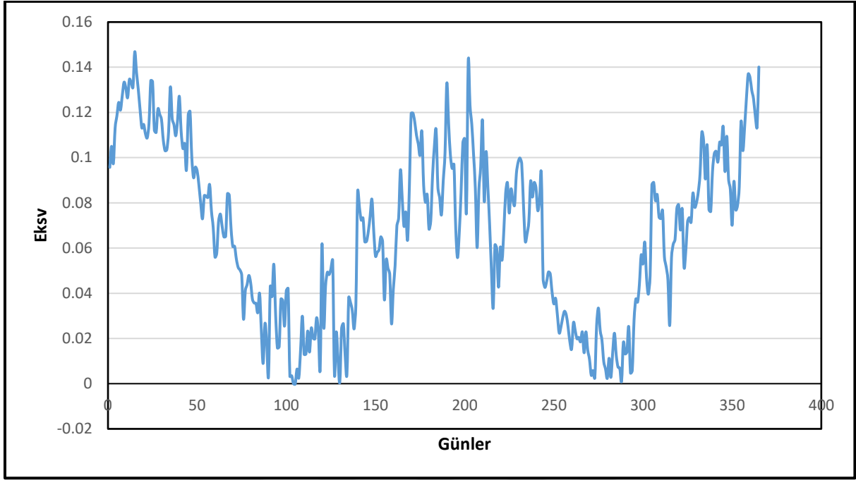
Şekil 6.6. Herat Şehrine ait ekserji verimi
