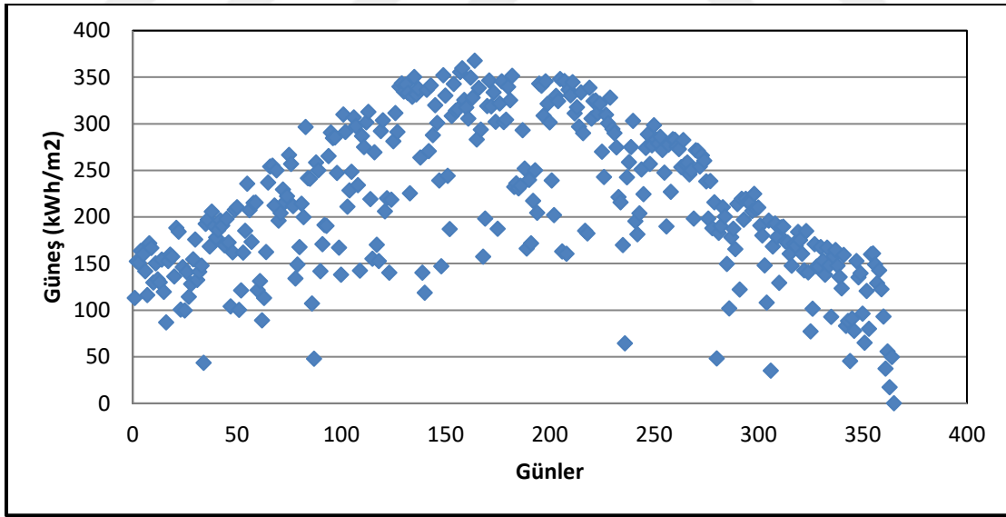
Şekil 6.9. Kandağhar şehrine ait gün- güneş ışıınıımı grafiğı
